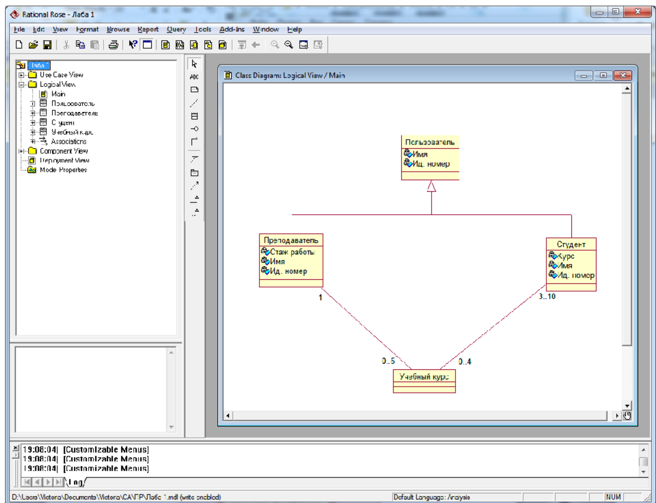
Рисунок 4.12 – Окончательный вариант простой диаграммы классов
