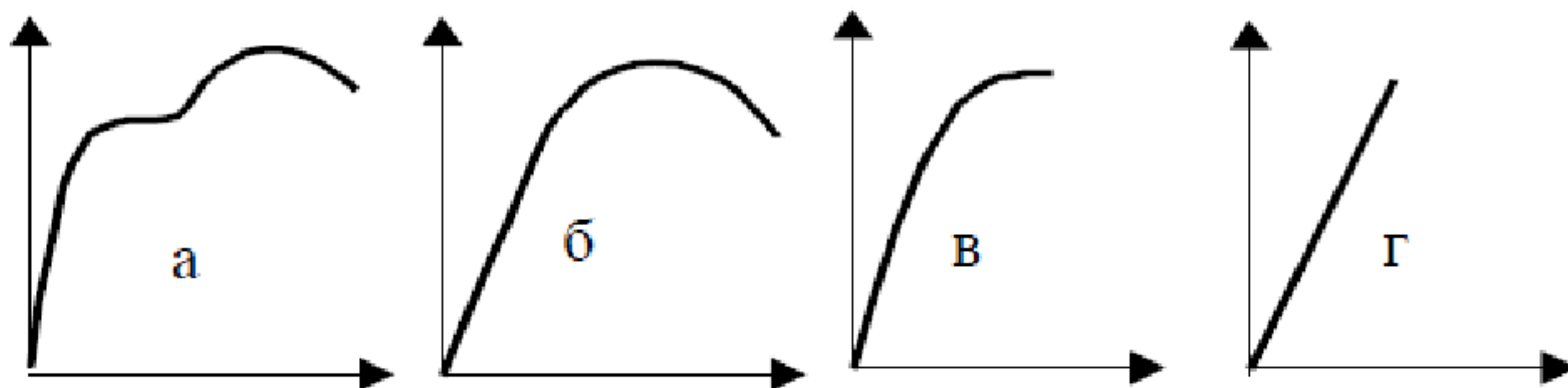
Рисунок 2 – Диаграммы растяжений
