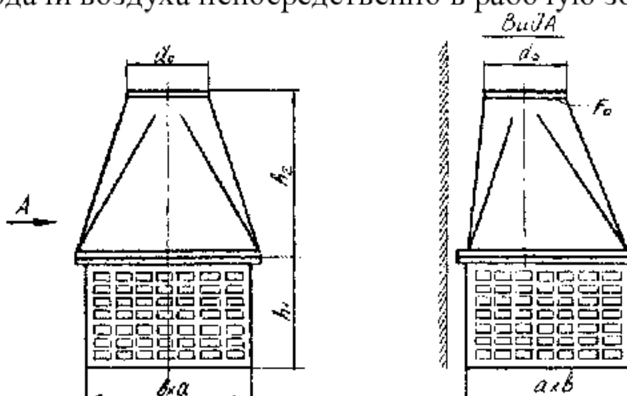
Рис.6. Пристенный воздухораспределитель типа ВП
