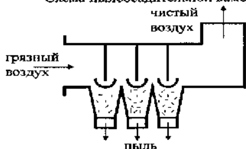
Схема пылеосадительной камеры:
