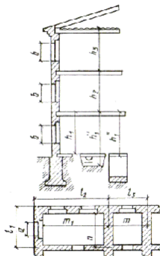
Рис. 1. Смеха обмера теплопередающих ограждений
