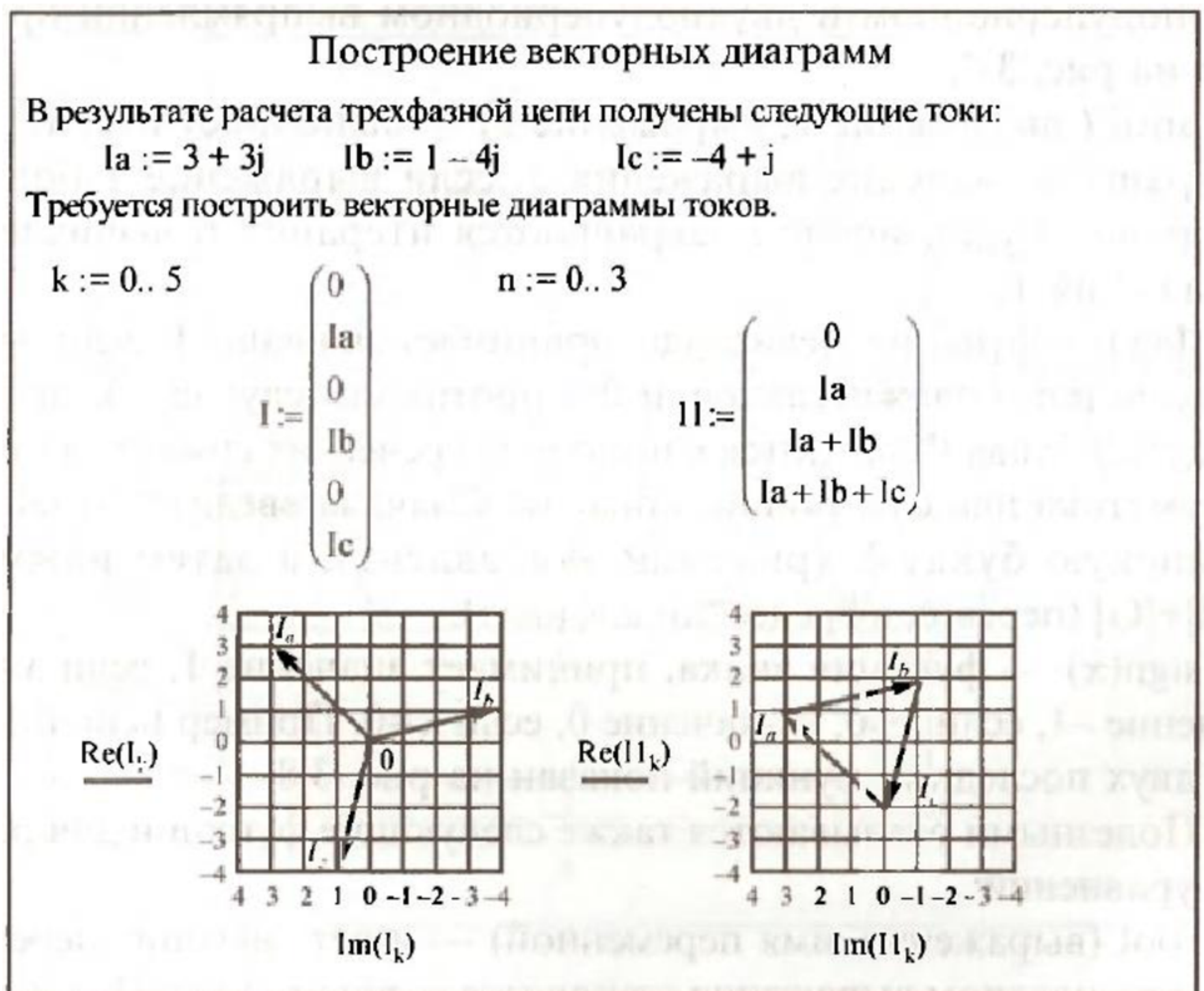
Рис. 3.6. Построение векторных диаграмм для симметричной трехфазной цепи
