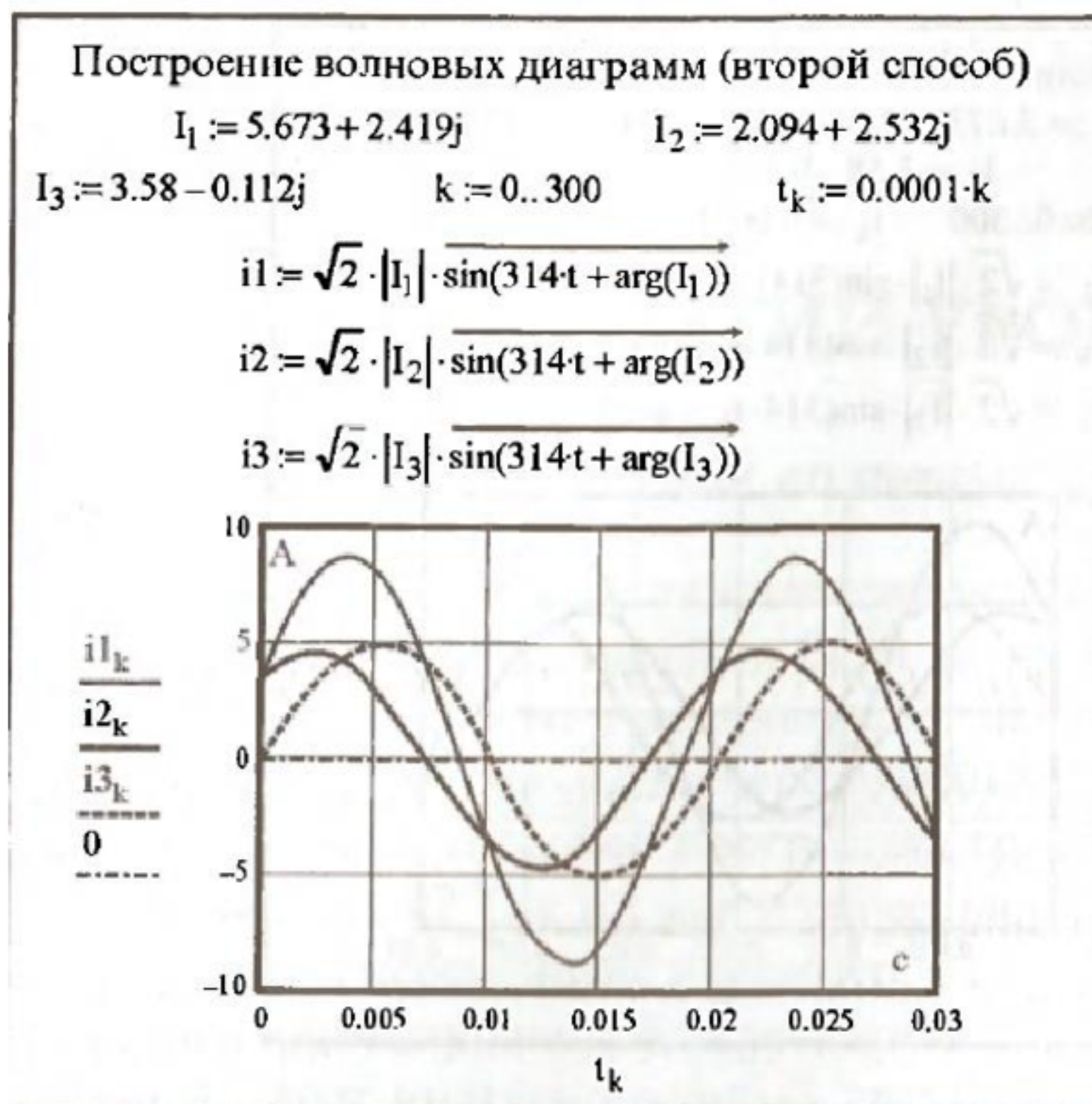
Рис. 3.2. Построение волновых диаграмм с использованием оператора векторизации
