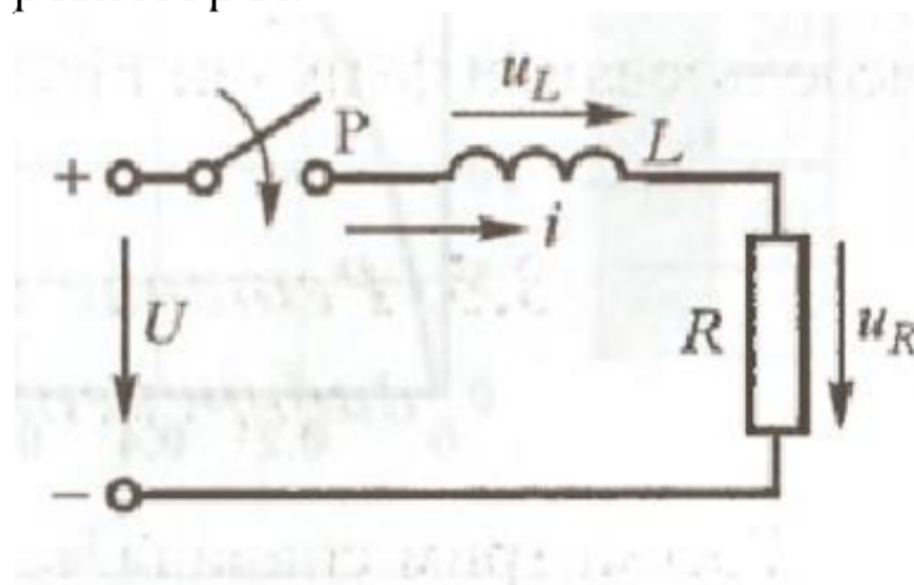
Рис. 3.10. Включение цепи R , L на постоянное напряжение
