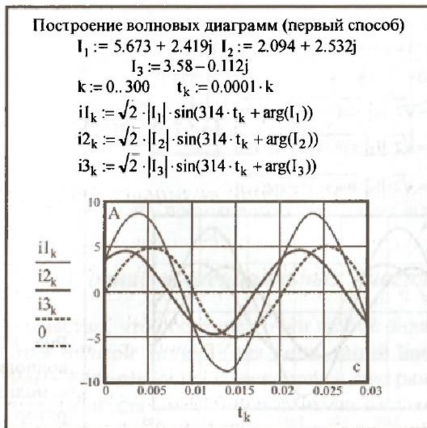
Рис. 3.1 Построение волновых диаграмм с применением индексированных переменных
