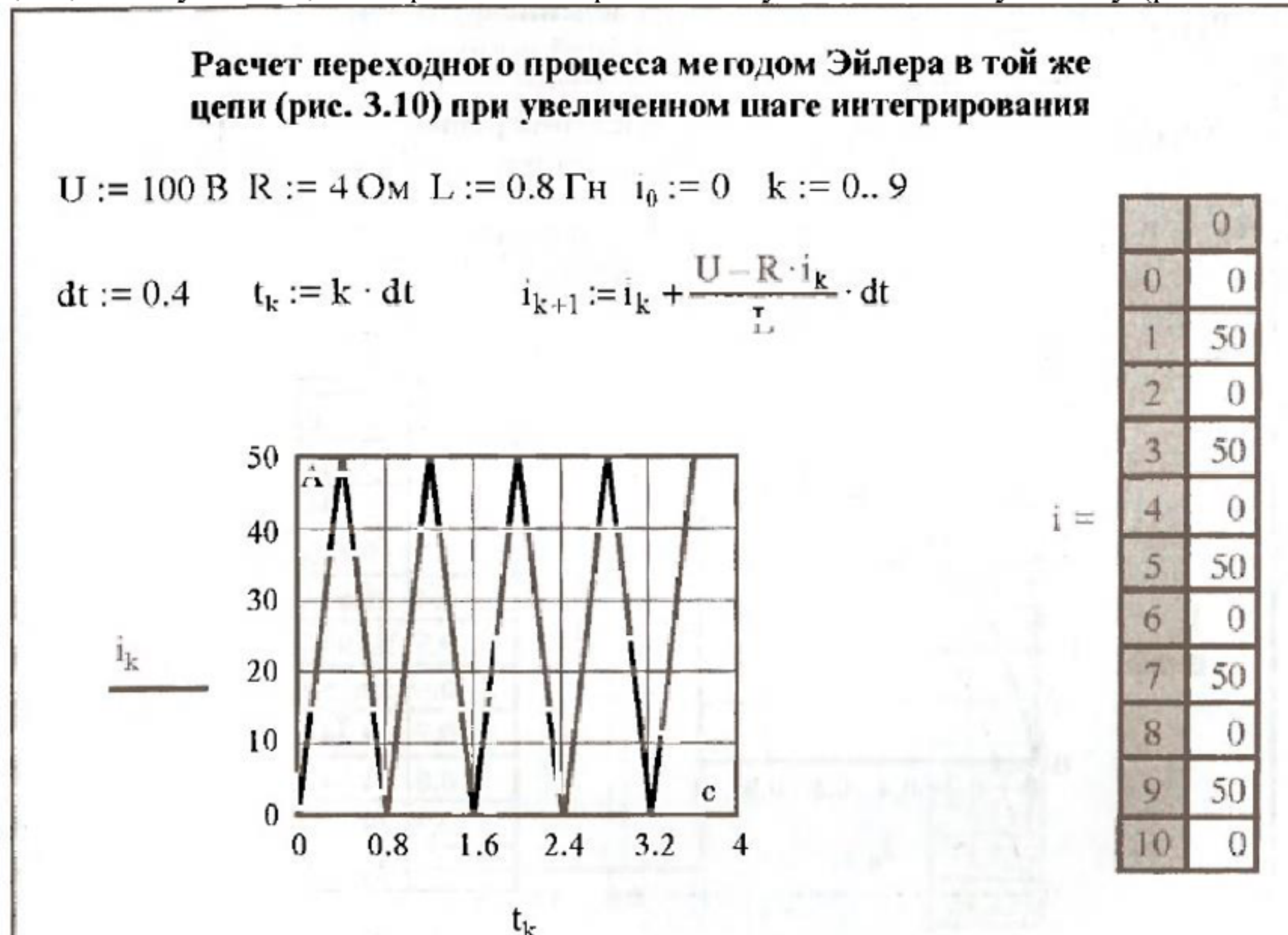
Рис. 3.12. Неустойчивый процесс при увеличении шага интегрирования
