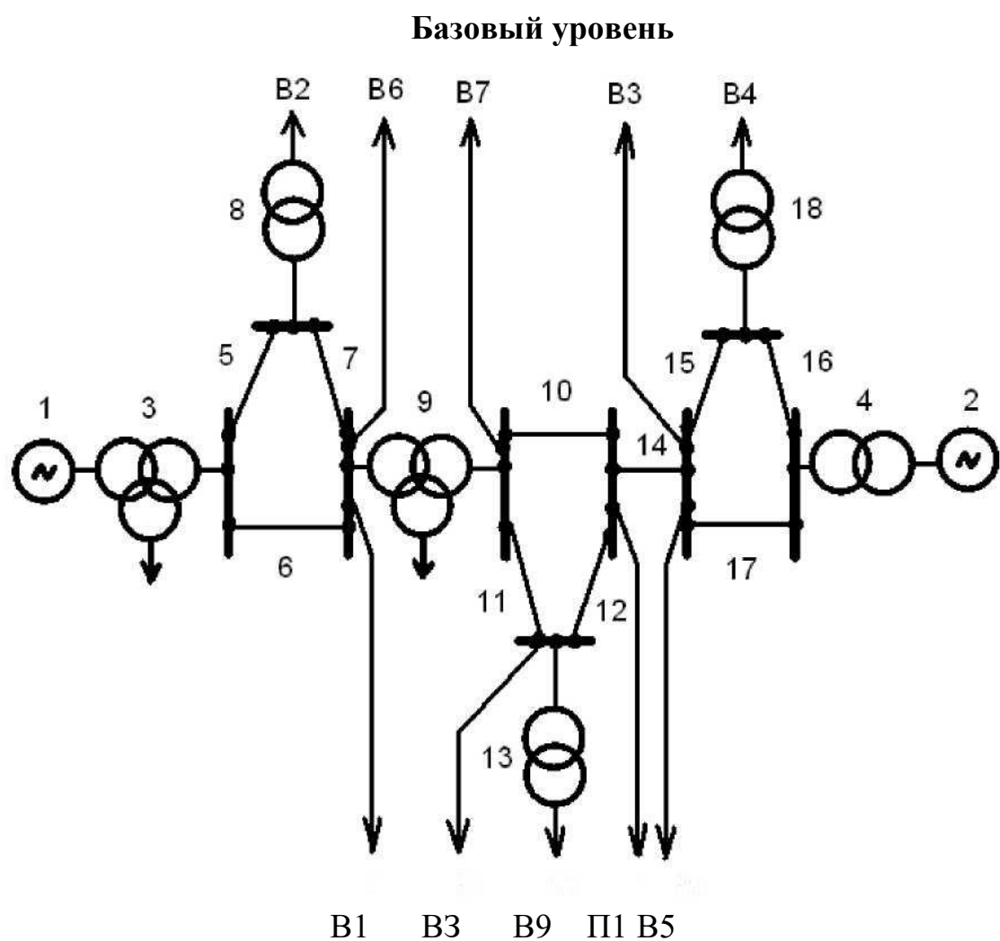
Рис. 1. Схема системы электроснабжения потребителей по вариантам
