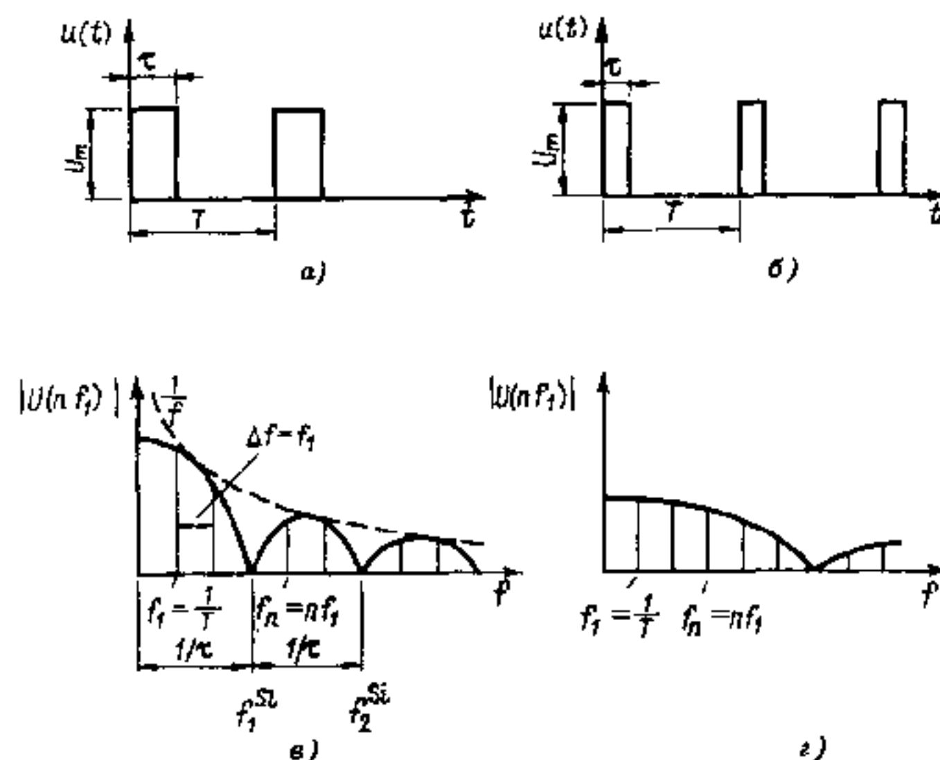
Рисунок 4 – Линеячатые спектры двух периодических последовательностей прямоугольных импульсов напряжений с личной скважностью (1:2): функция Si(x) - огибающая спектральных амплитуд (сплошная кривая); функция 1/f - огибающая функции Si(x) (пунктирная кривая)
