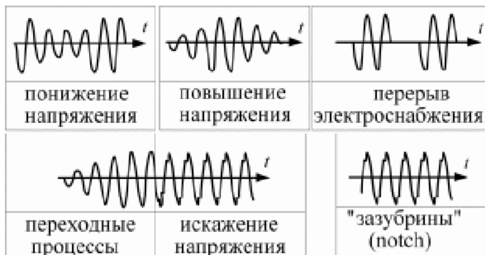
Рисунок 1 – Основные случаи ухудшения качества электроэнергии
