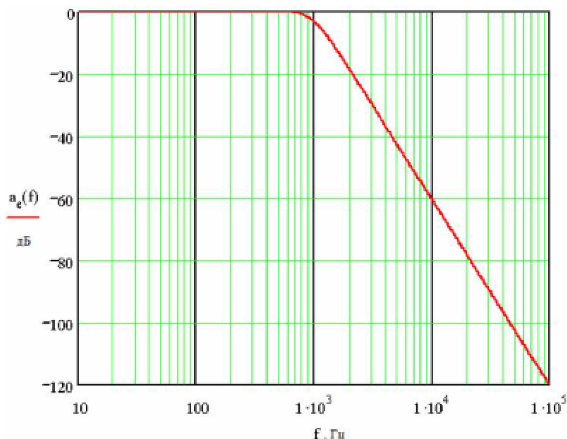
Рисунок 1 - АЧХ фильтра
