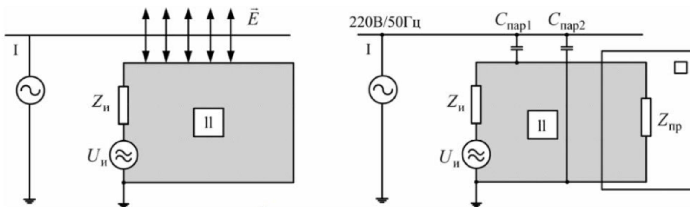
Рисунок 2 – Ёмкостной путь передачи ЭМС
