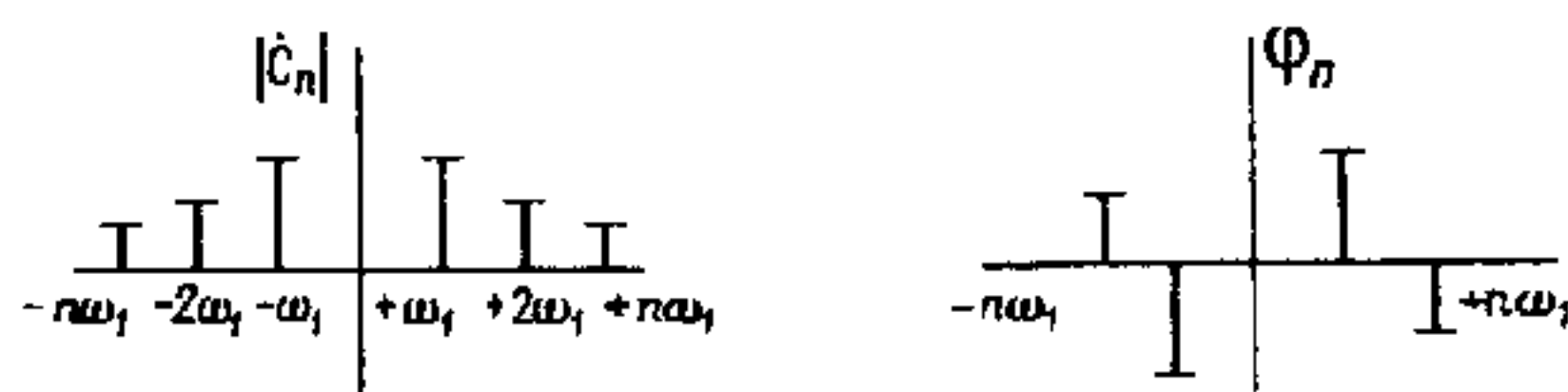
Рисунок 3 – Амплитудный и фазовый спектры комплексного ряда Фурье
