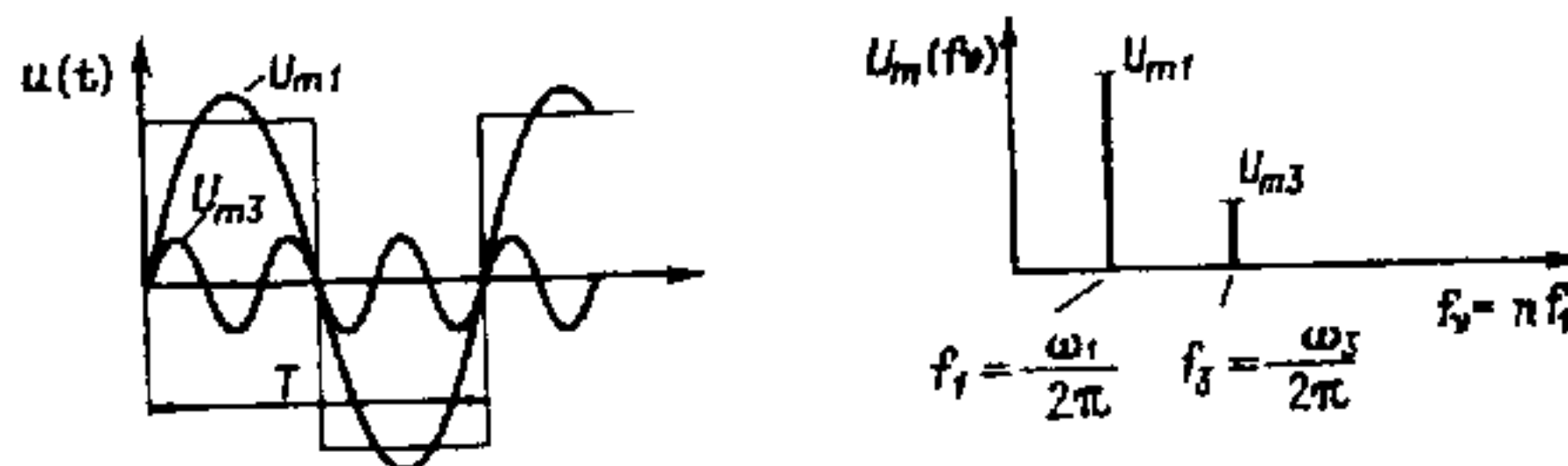
Рисунок 2 – Периодическая несинусоидальная функция
