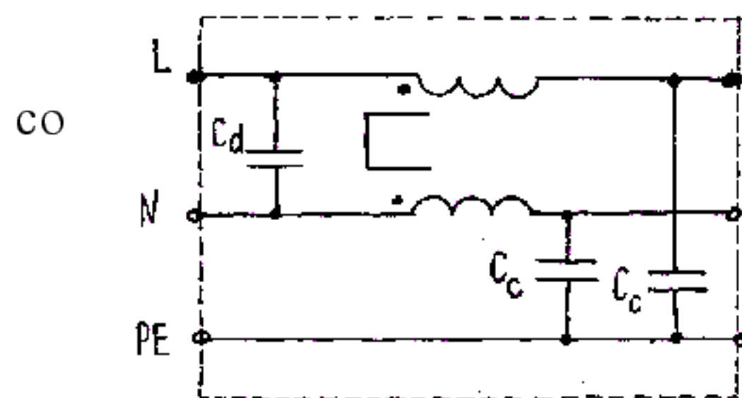
Рисунок 4 - Пример сетевого фильтра на 220 В, ток 1 А, а) схема, б) частотные зависимости: 1 – противофазные
