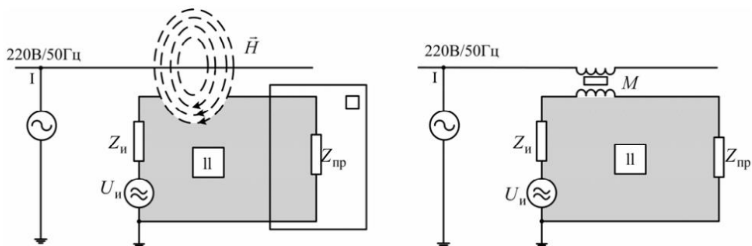
Рисунок 3 – Индуктивный путь передачи ЭМП
