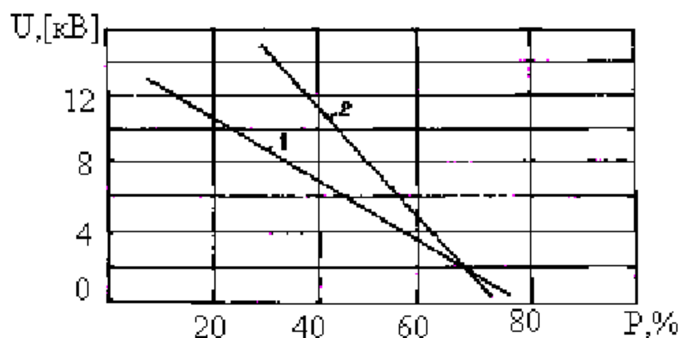
Рисунок 3 - Зависимость от влажности R потенциала человека при ходьбе по полу
