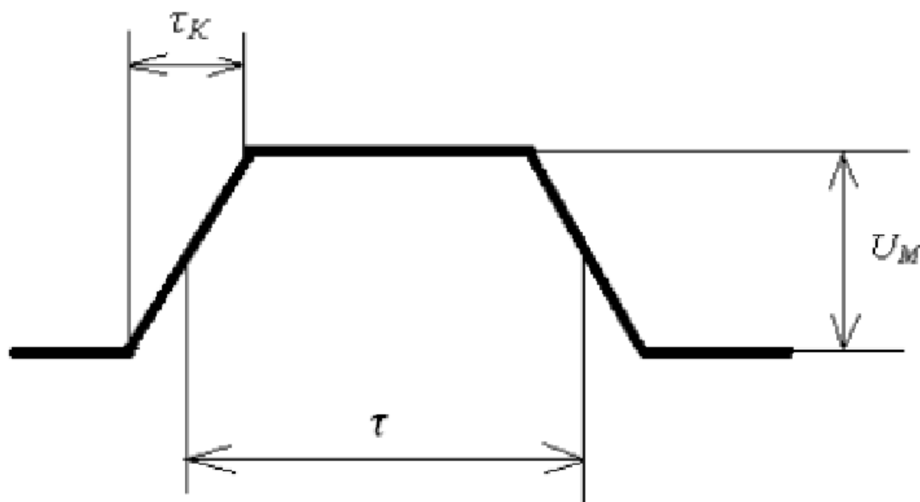
Рисунок 2- Трапециевидный импульс
