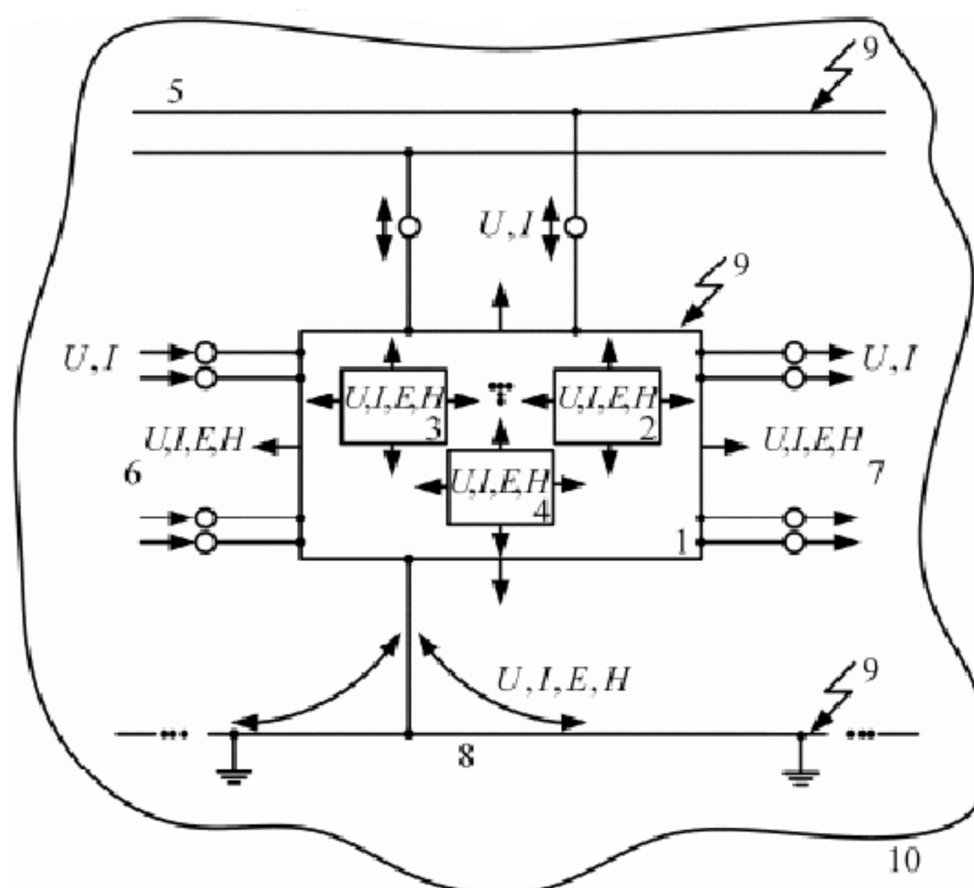
Р и с у н о к 6 – В н е ш н и е и в н у т р е н н и е и с т о ч - н и к и п о м е х , в и д ы п о м е х , п о с т у п а ю щ и х в у с т р о й с т в о и и с х о д я щ и х и з н е г о п о м е х : 1 - п р и б о р а в т о м а т и з а ц и и ; 2, 3 , 4 - э л е м е н т ы п р и - б о р а а в т о м а т и з а ц и и , в н у т р е н н и е и с т о ч н и к и Э М П ; 5 - с е т ь э л е к т р о п и т а н и я ; 6 - и н ф о р м а ц и - о н н ы е в х о д ы ; 7 - и н ф о р м а ц и о н н ы е в ы х о д ы ; 8 - з а з е м л е н и е ; 9 - Э М П , п е р е д а ю щ и е с я п о к о н т у - р у з а з е м л е н и я , р а з р ы д ы с т а т и ч е с к о г о э л е к - т р и ч е с т в а , к о р о т к и е з а м ы к а н и я в п и т а ю щ е й с е т и ; 10 - э л е к т р о м а г н и т н а я о б с т а н о в к а .
