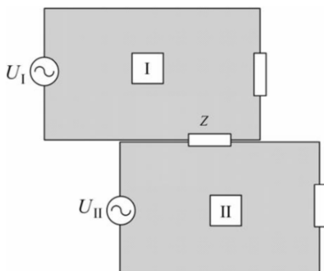
Рисунок 1 – Гальванический путь передачи ЭМС
