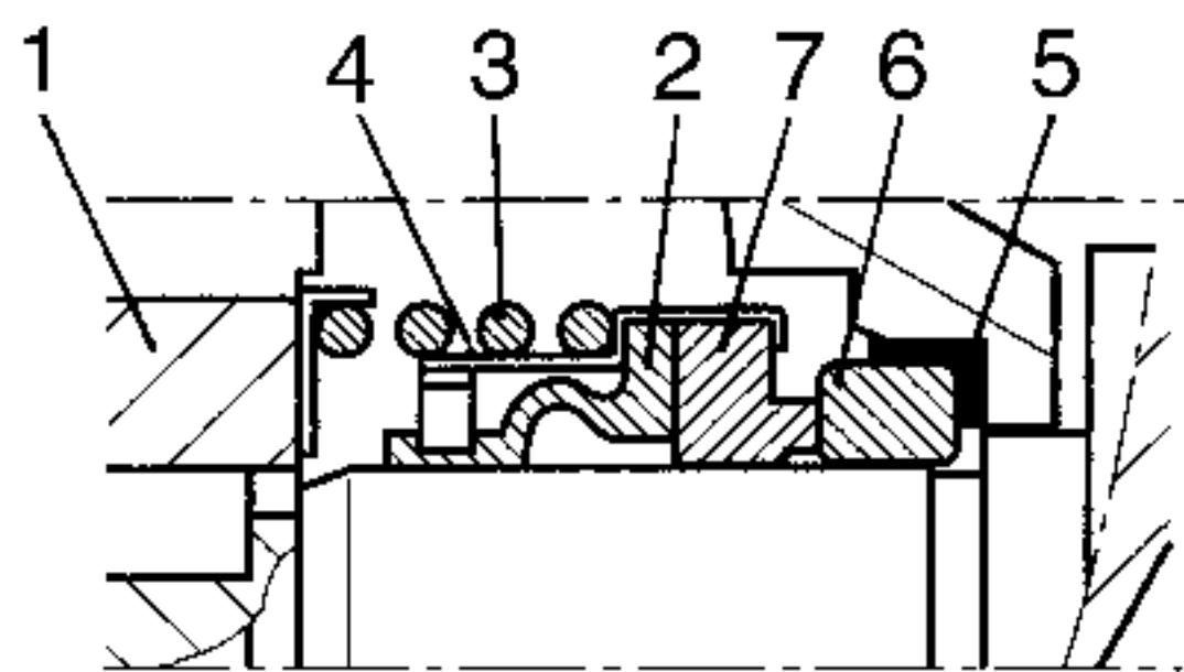
Рис. 3. Скользящее торцевое уплотнение
