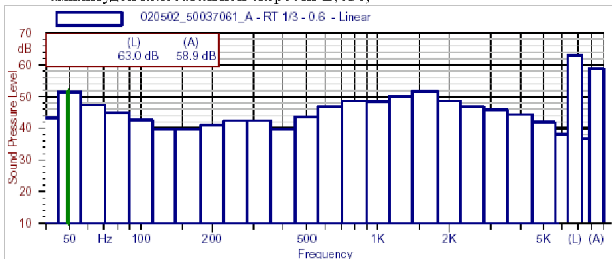
Рис. 3. Спектры уровня звука от частоты для насосной станции СО – 3МНІ402/ER-WMS
