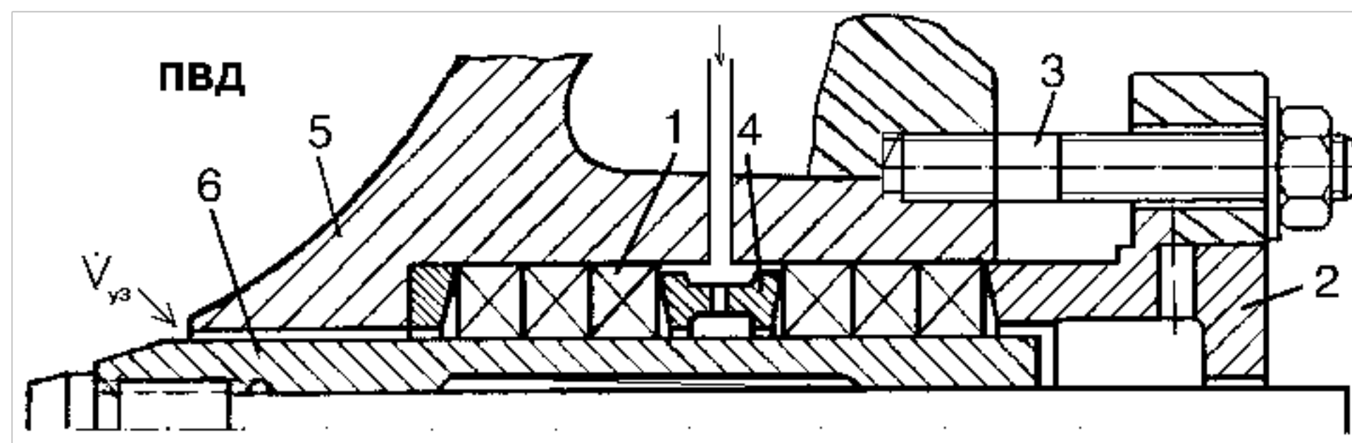
Рис. 2. Сальник
