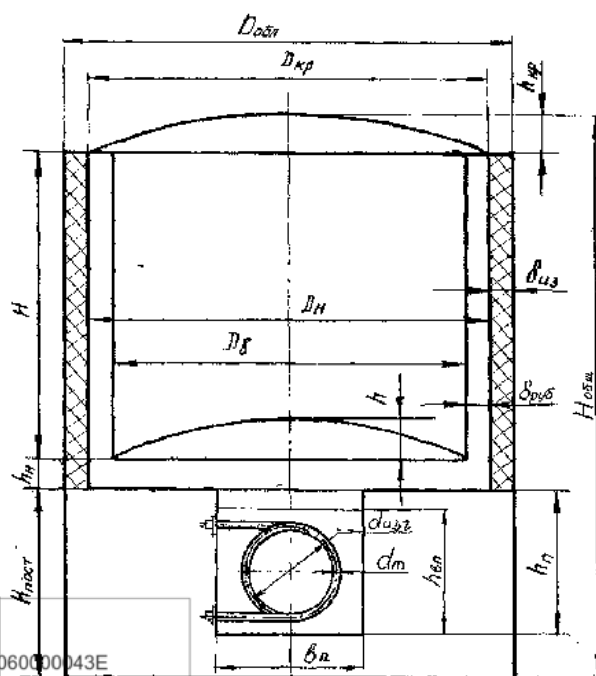
Рисунок 7.3 - Расчетная схема варочного котла с электрическим обогревом:
