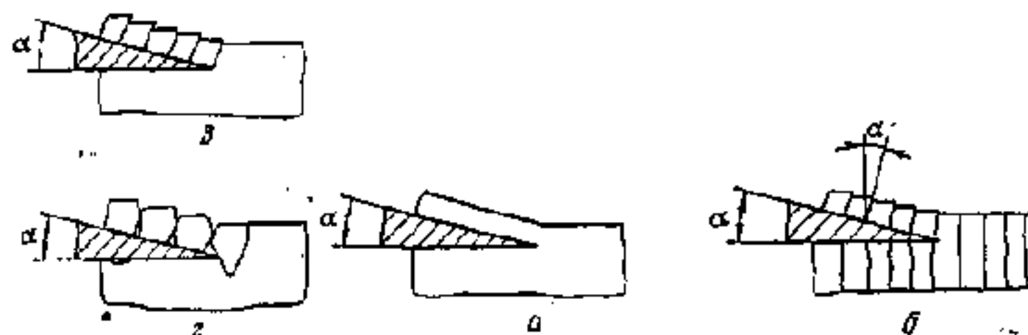
Рисунок 2.4 - Схема деформации различных продуктов при рубящем резании: а — пластичных продуктов; б — волоконистых продуктов; в — неволоконистых твердых продуктов; г — твердых хрупких продуктов
