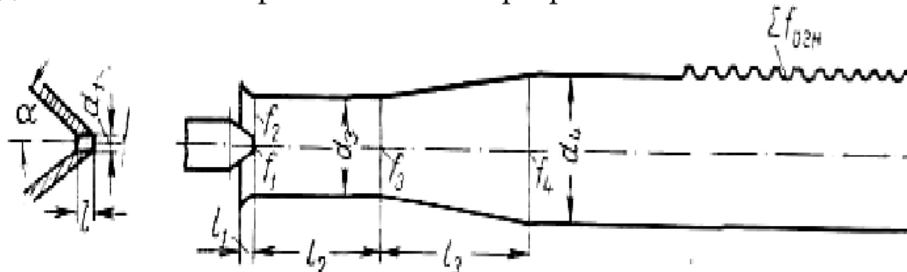
Рисунок 6.3 - Схема атмосферной горелки.
