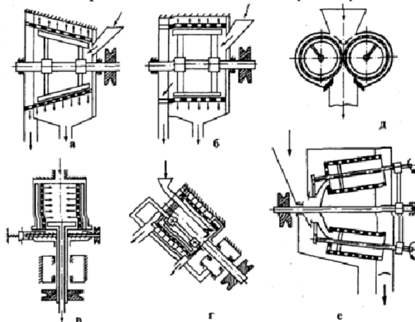
Рисунок 1.1 - Основные конструктивные схемы протирачных машин:
