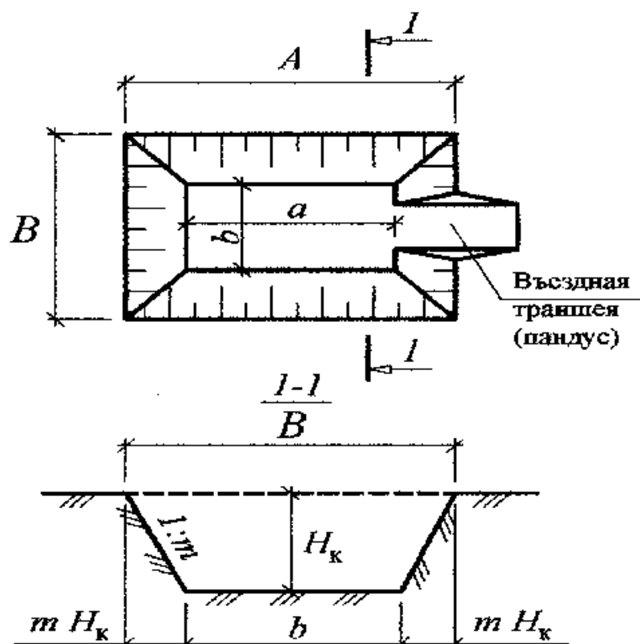
Рис. 5. Схема котлована
