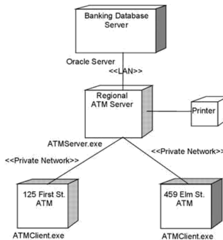
Рисунок 3.19 - Пример диаграммы размещения
