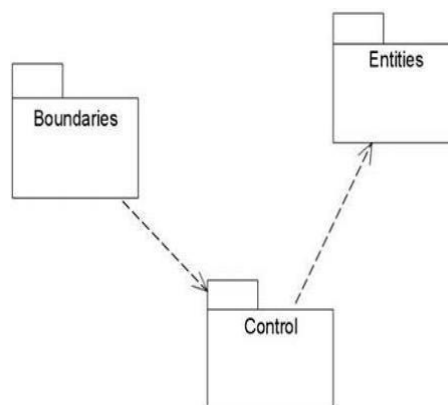
Рисунок 3.17 - Пример диаграммы пакетов
