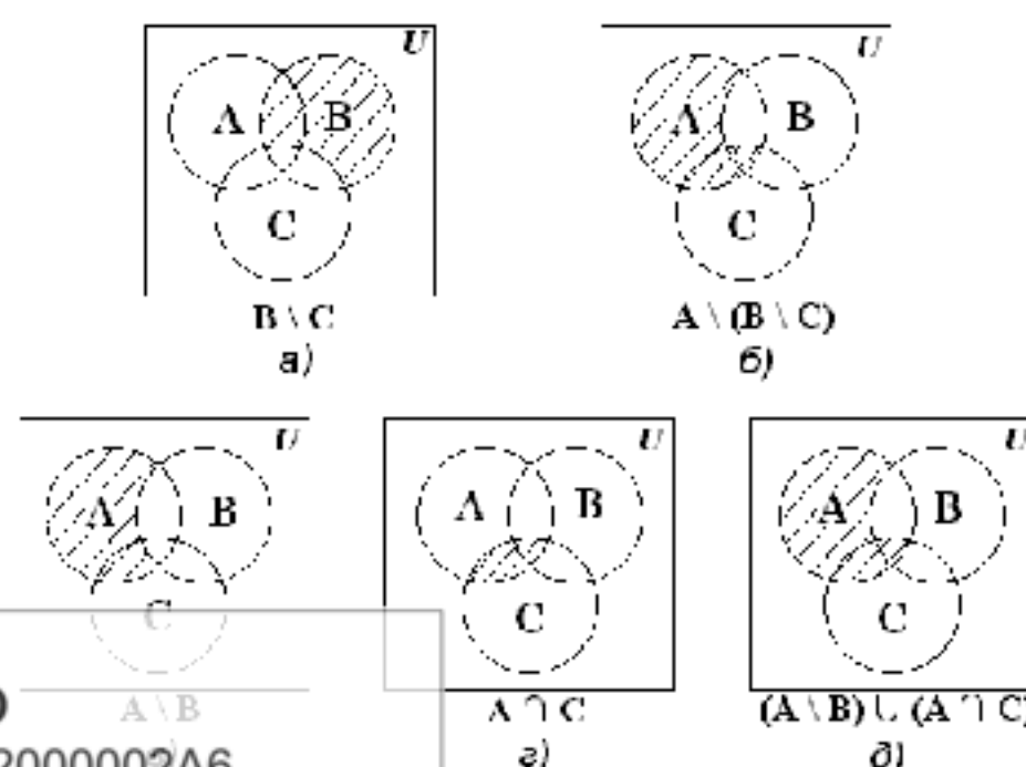
Рис. 1.2. Диаграммы Эйлера-Венна
