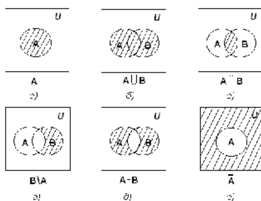
Рис. 1.1. Диаграммы Эйлера-Венна
