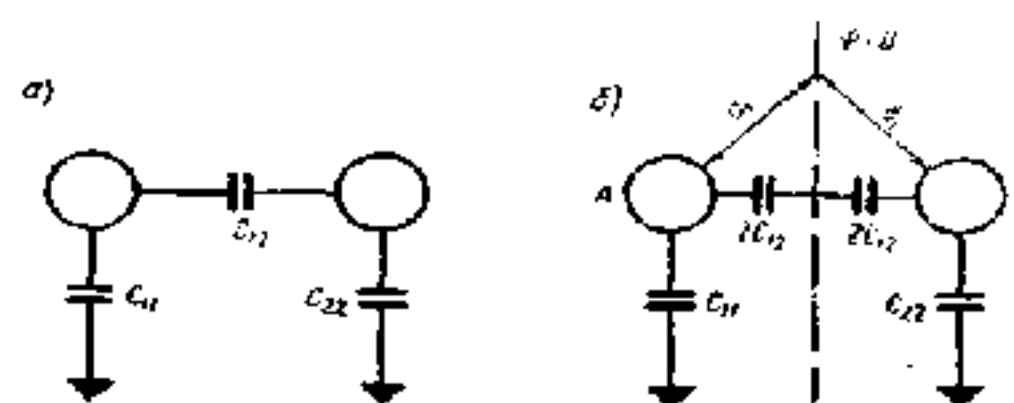
Рисунок 3.2 – Схема для расчета частичных емкостей двухпроводной линии: а — для расчета емкости линии; б — для расчета рабочей емкости провода
