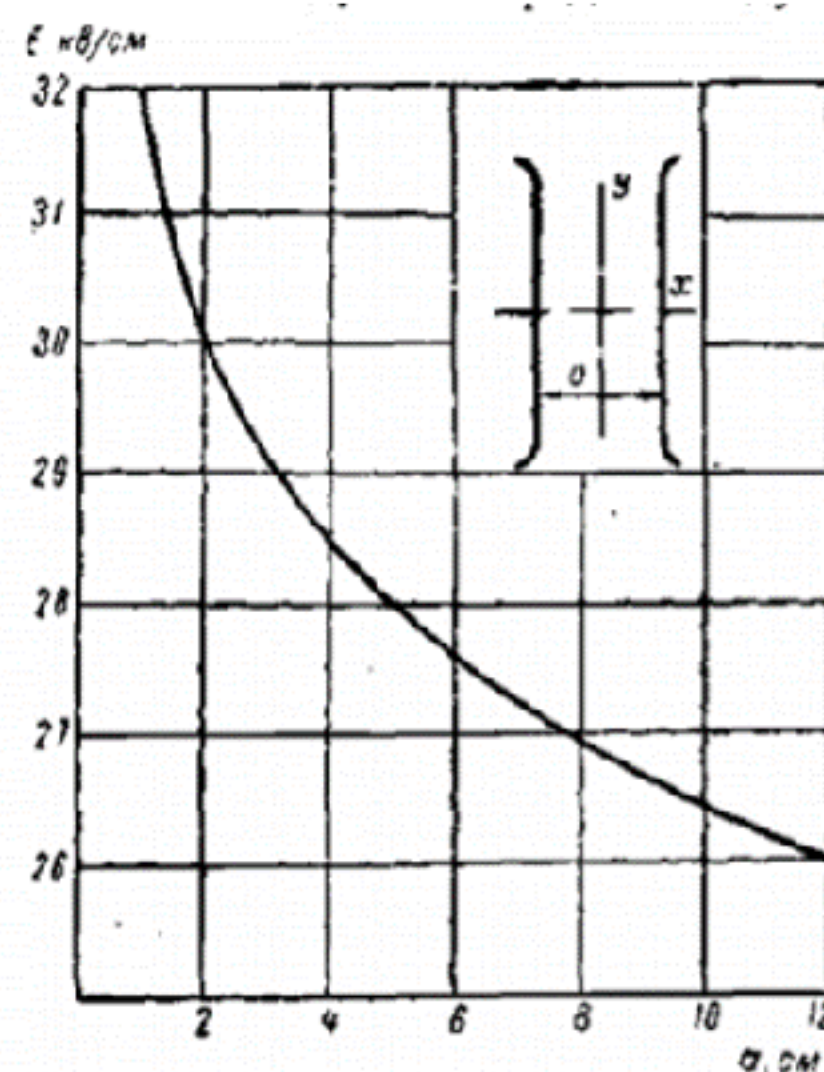
Рисунок 2.2 – Опытная характеристика зависимости пробивной
