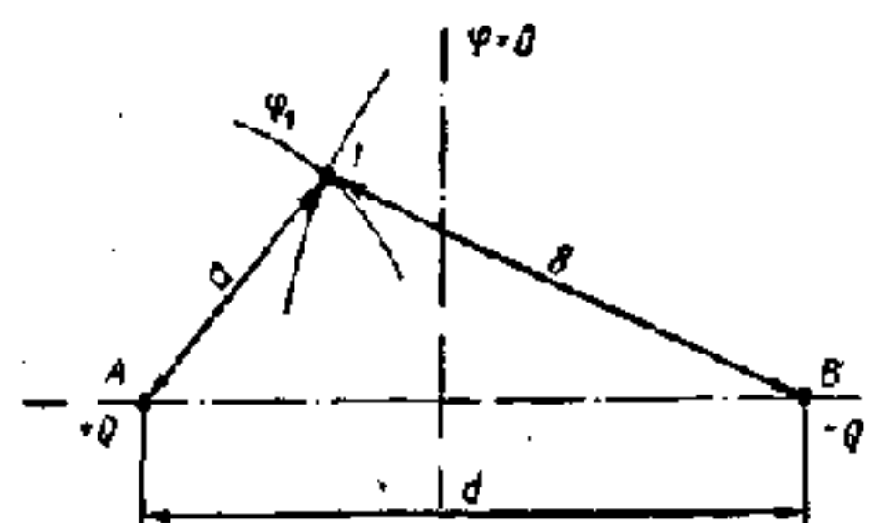
Рис. 10. Схема расположения электрических осей
