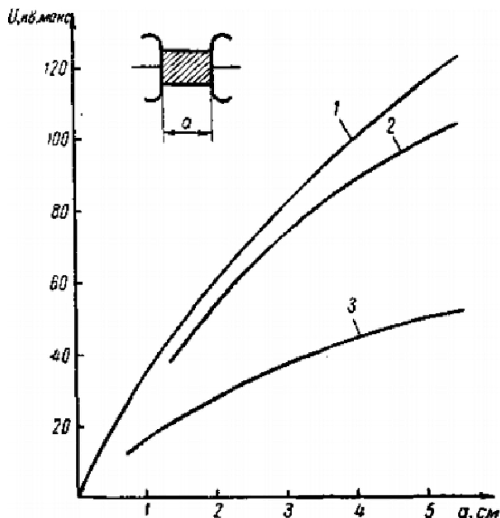
Рисунок 6.2 – Разрядные напряжения между плоскими электродами: 1 - по воздуху; 2 — по поверхности пар 3 — по поверхности стекла
