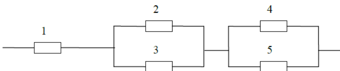
Рисунок 1. Структурная схема надежности
