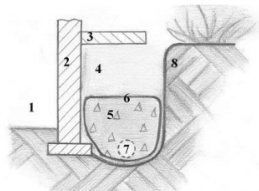
Рисунок 1 - Схема устройства пристенного дренажа
