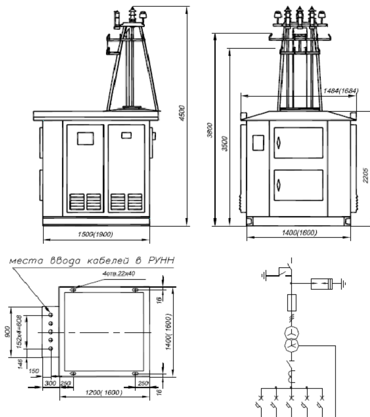
Рисунок 2 – КТП тушковая с воздушным вводом
