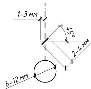
Рисунок 1. Правила оформления координационных осей
