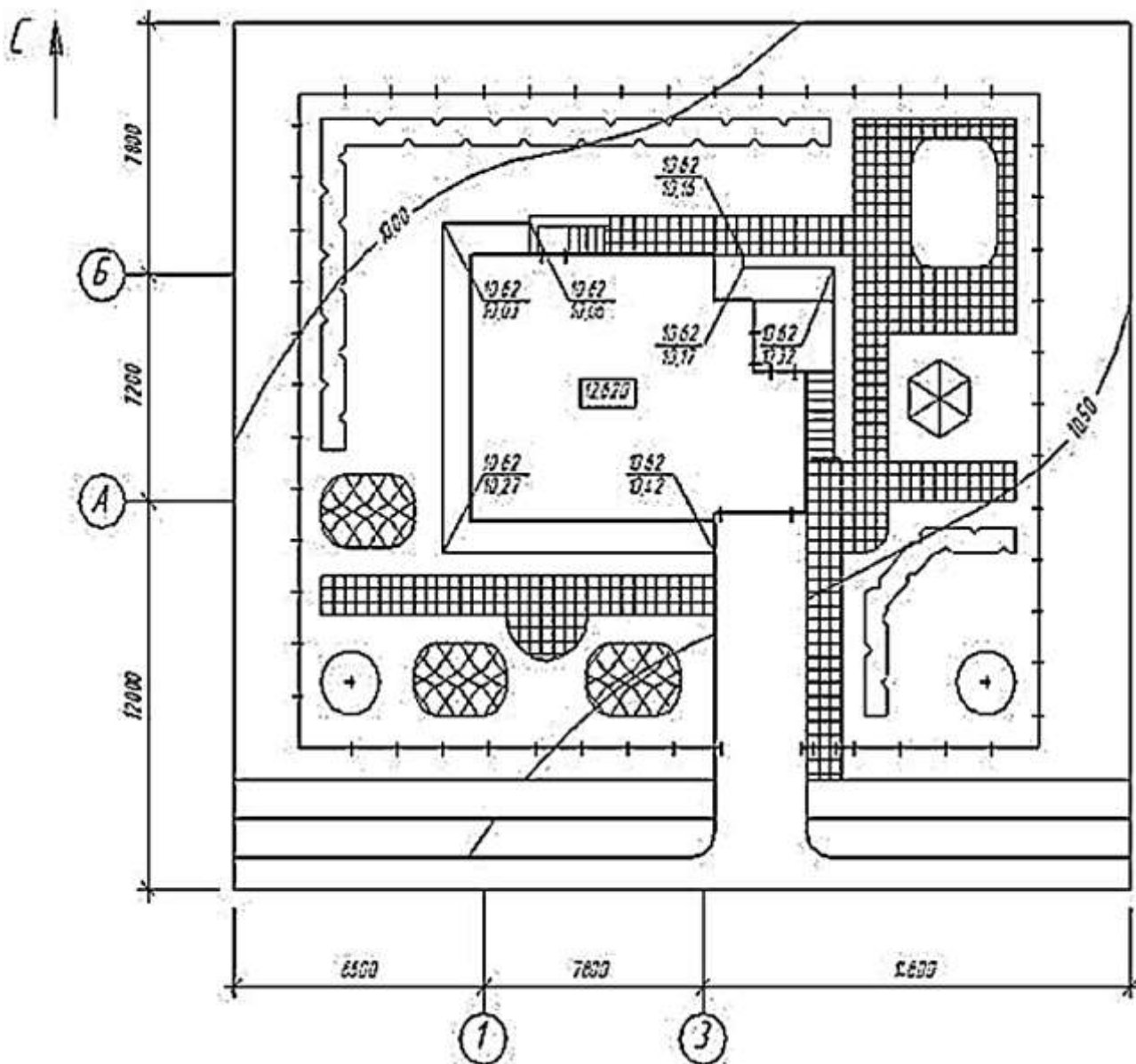
Рисунок 2. Вертикальная привязка здания.
