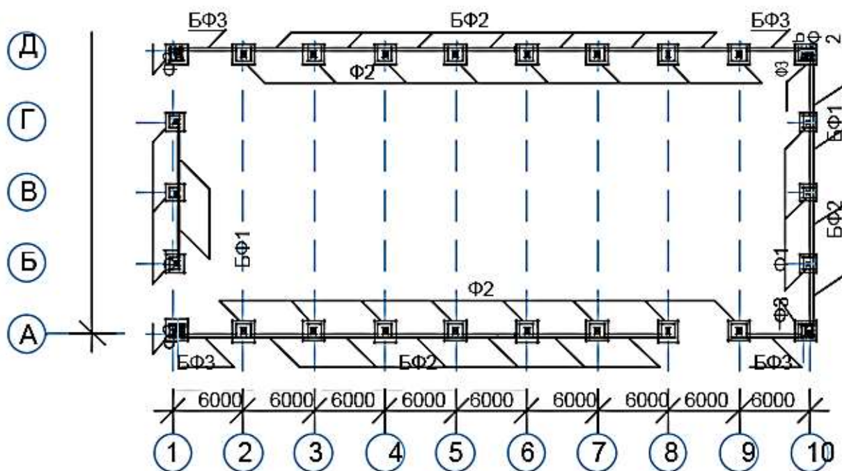
Рисунок 26 – Схема расположения фундаментов
