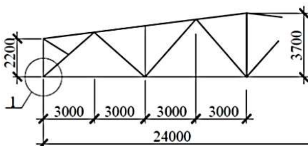
Схема фермы М 1:200
