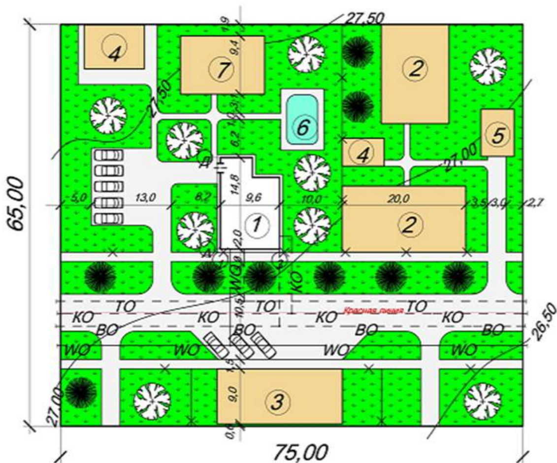
Рисунок 1 Генплан М 1:500
