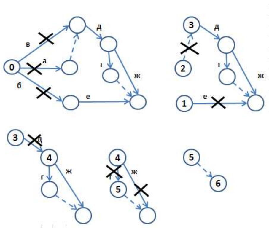
Рис. 11. Порядок нумерации сетевого графика
