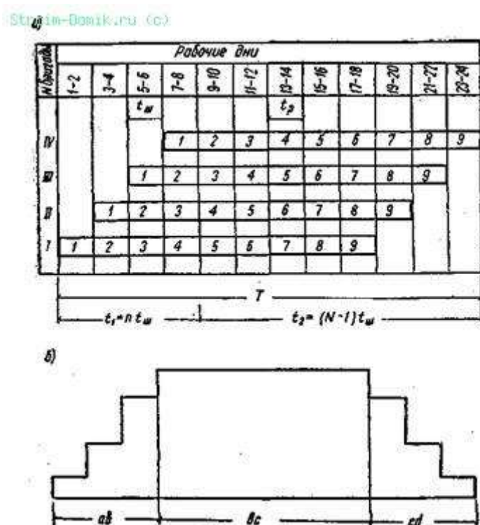
Рис. 2. Производство работ поточным методом с постоянным ритмом
