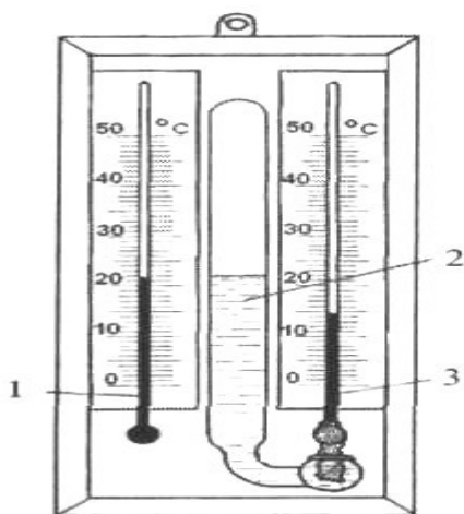
Рис. 1.4. Психрометр Августа:
