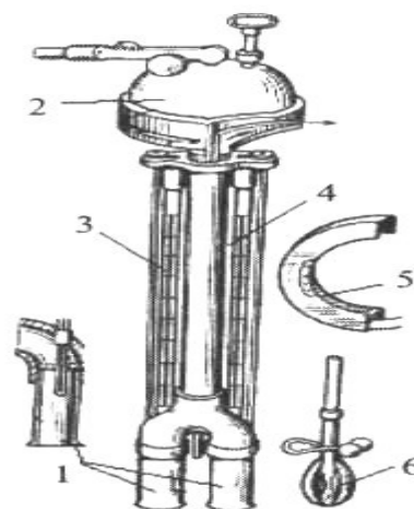
Рис. 1.5. Аспирационный психрометр Ассмана:
