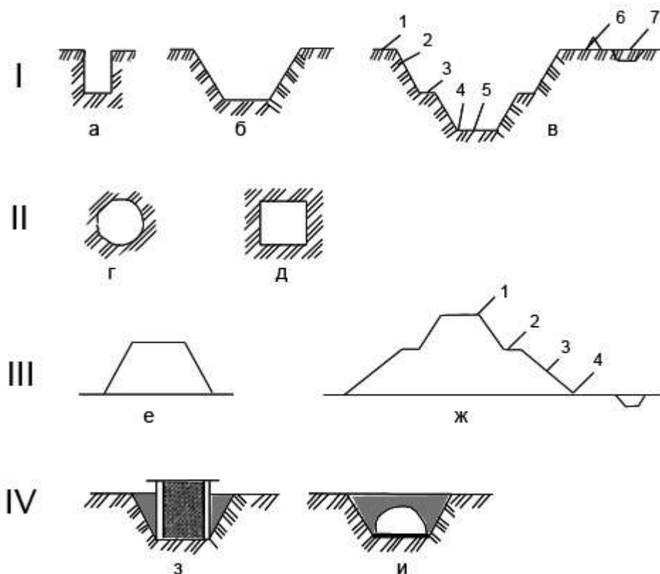
Рис.1. Виды земляных сооружений:
