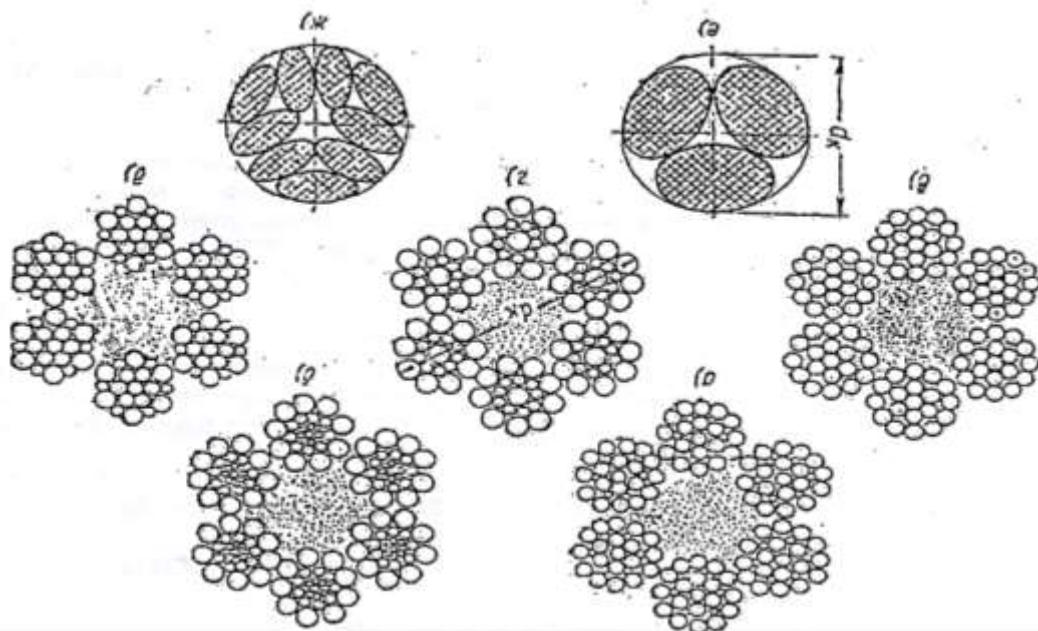
Рис. 3. Поперечные сечения канатов различных конструкций: а) ЛК-З 5х25+1ос; б) ТЛК-Р 6х27+1ос; в) ТК 6х19+1ос; г) ЛК-О 6х19+1ос д) ЛК-Р 6х19+1ос; е) пеньковый обыкновенный; ж) пеньковый отворотный
