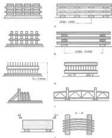
Рис. 2. Складирование стальных конструкций: а — балок и колонн плашмя; б — двухстеночных элементов; в — балок в вертикальном положении; г — фермы в полуклонном положении; д — свальцованных листов
