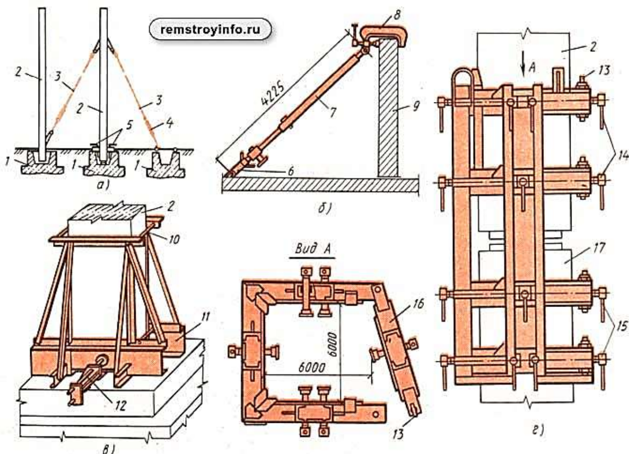
Рисунок 1. Приспособления для временного закрепления и выверки строительных конструкций
