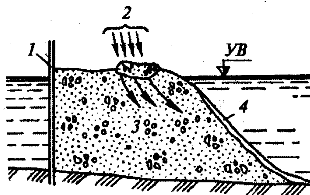
Рис. 1.4 Подводное бетонирование методом втрамбовывания:
