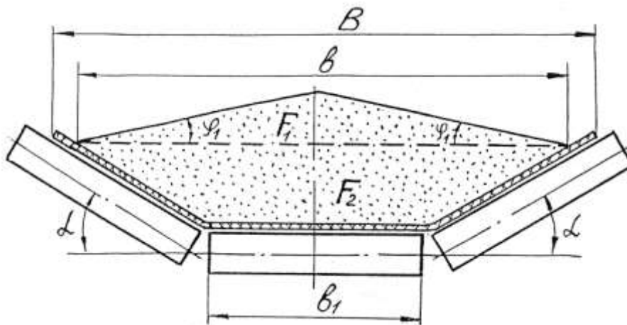
Рисунок 7 – Сечение потока материала на трёхроlikовой желобчатой роlikоопоре.
