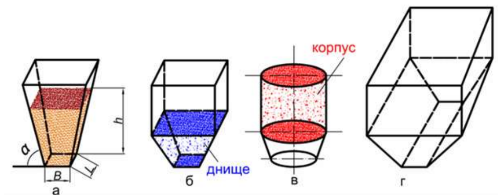
Рисунок 1. Схемы бункеров: а - пирамидальной формы; б - призма - пирамидальной формы; в - цилиндрической формы; г - лотковые
