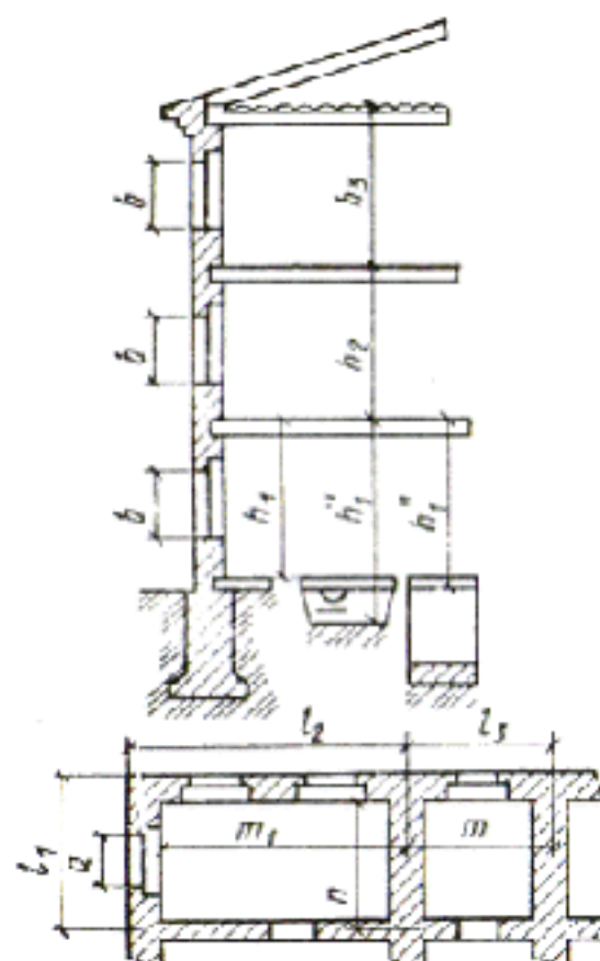
Рис. 1. Схе-ма обмера теплопередающих ограждений
