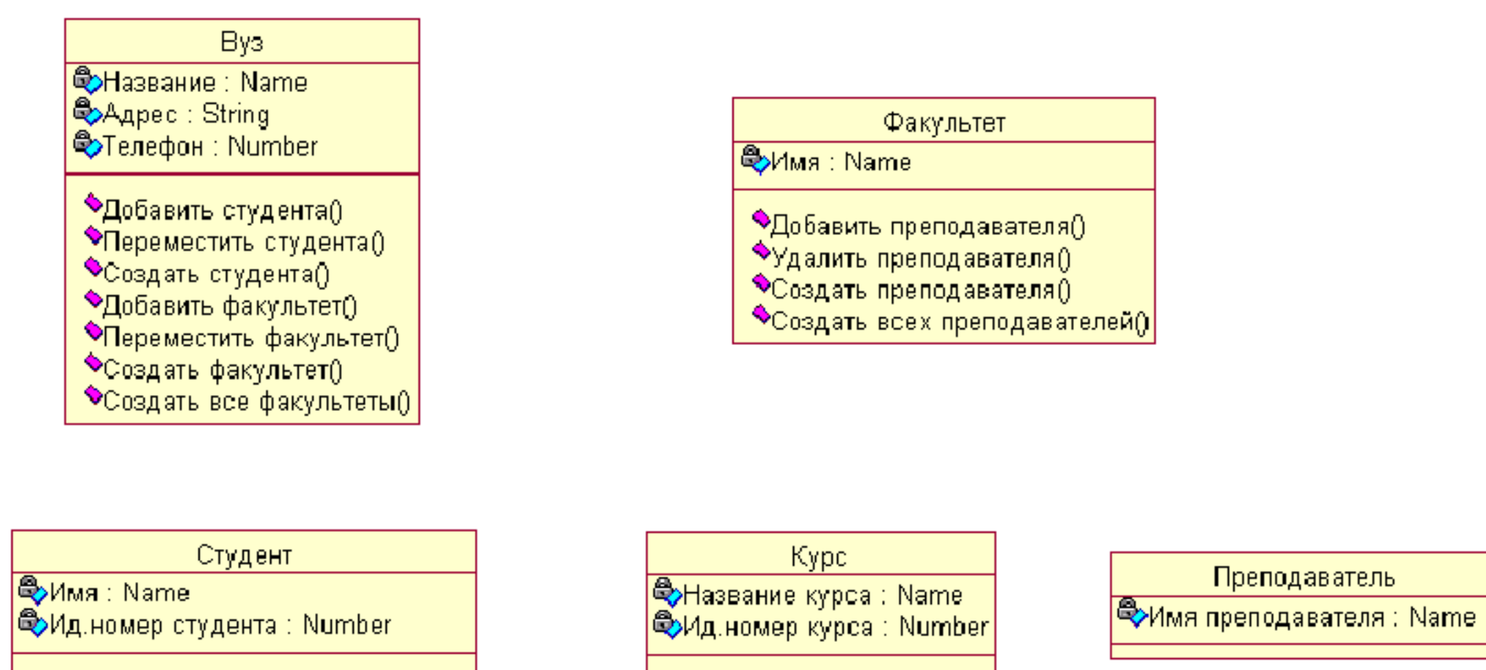
Рисунок 5.4 – Диаграмма классов с атрибутами
