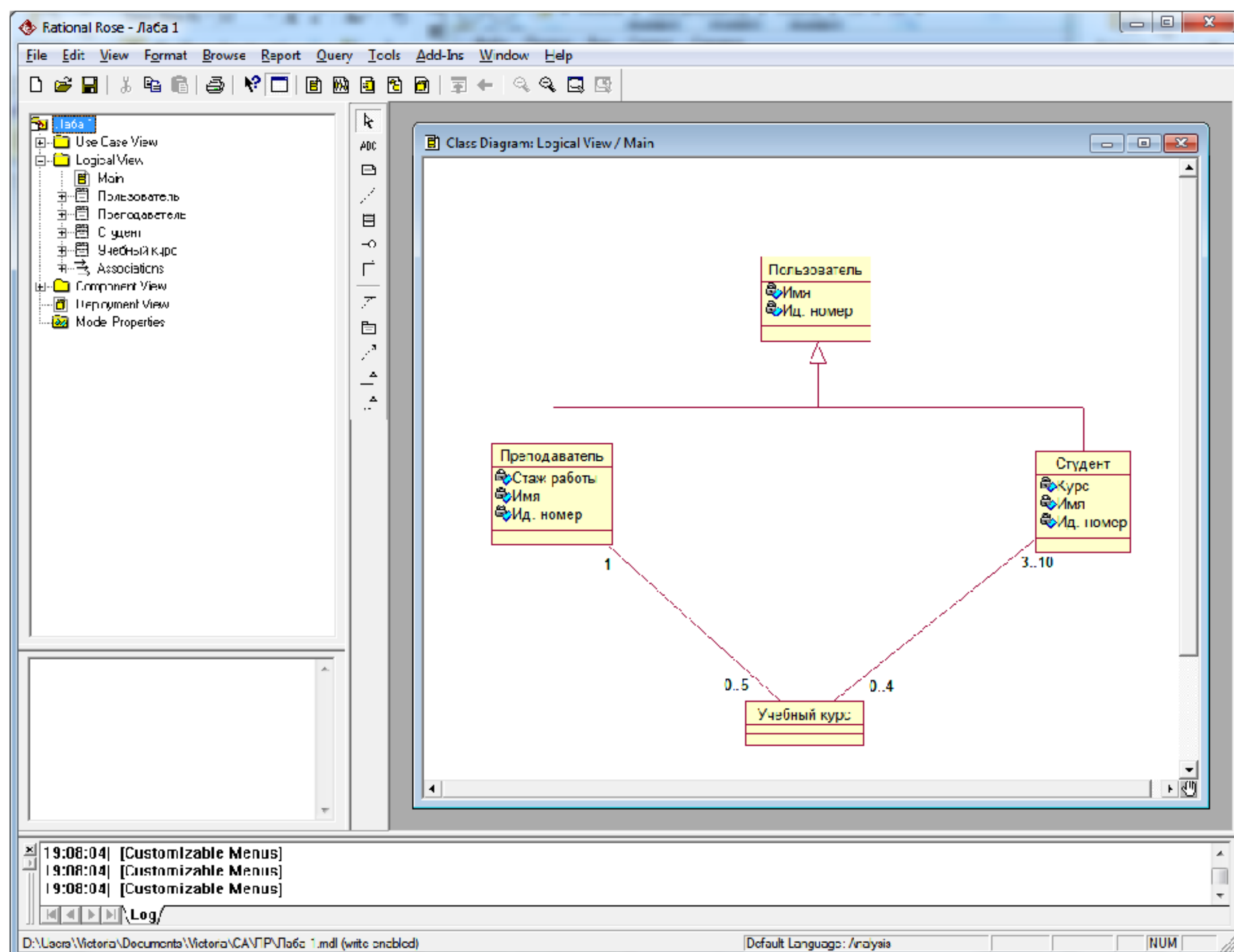
Рисунок 4.12 – Окончательный вариант простой диаграммы классов
