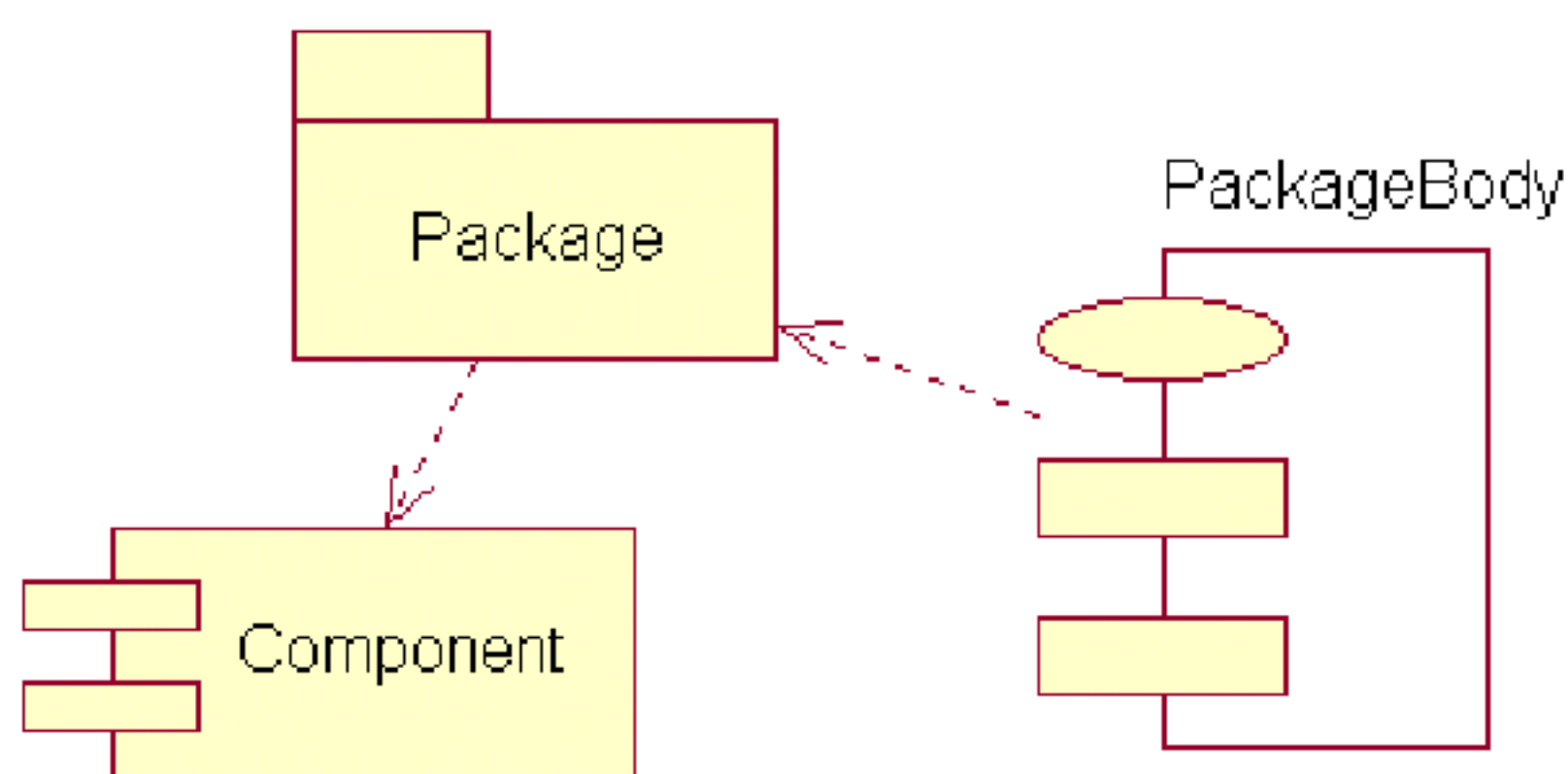
Рисунок 5.3 – Пример диаграммы компонентов
