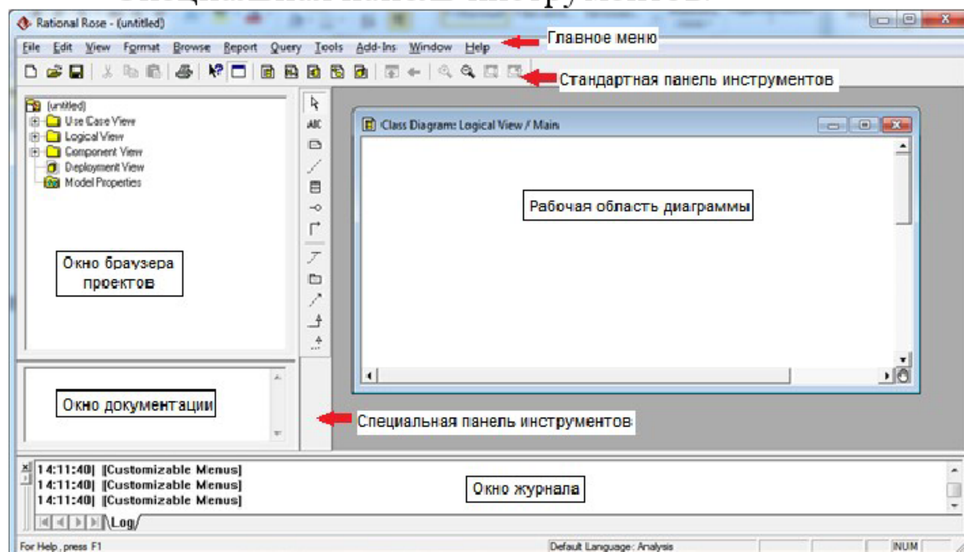
Рисунок 4.1 – Общий вид рабочего интерфейса CASE-средства Rational Rose
