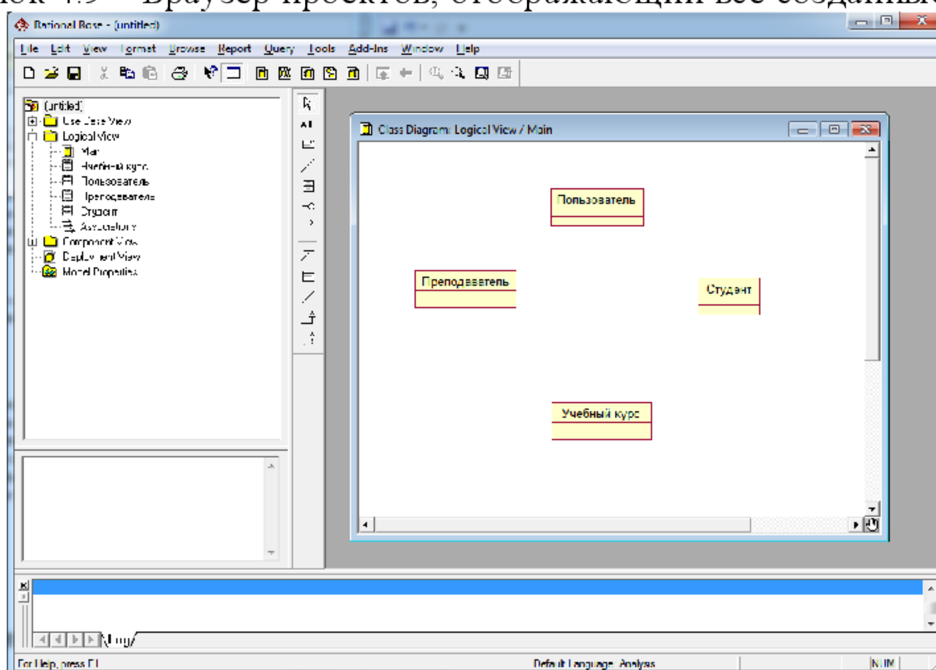
Рисунок 4.10 – Созданные классы в окне диаграммы классов
