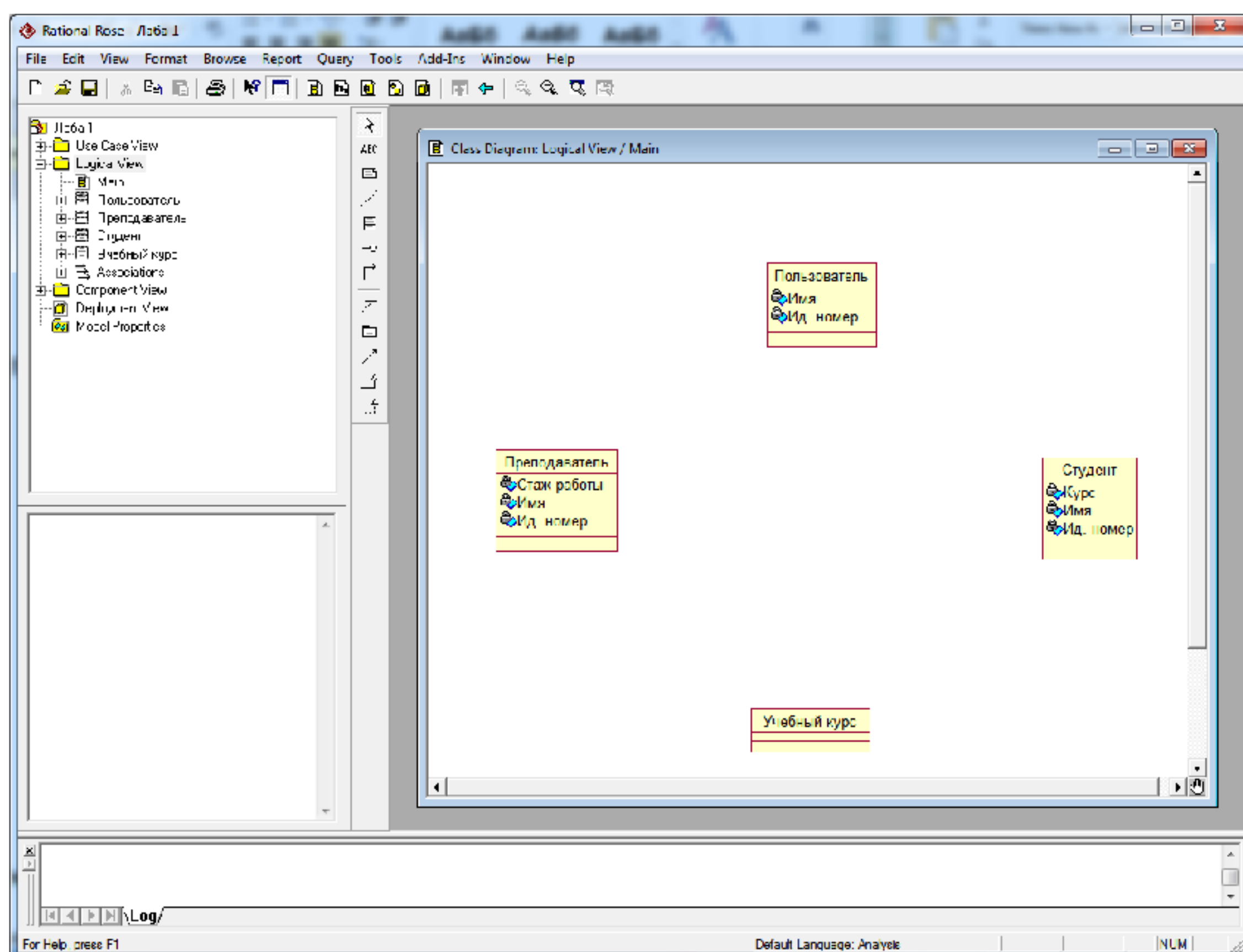
Рисунок 4.11 – Классы с атрибутами в окне диаграммы классов
