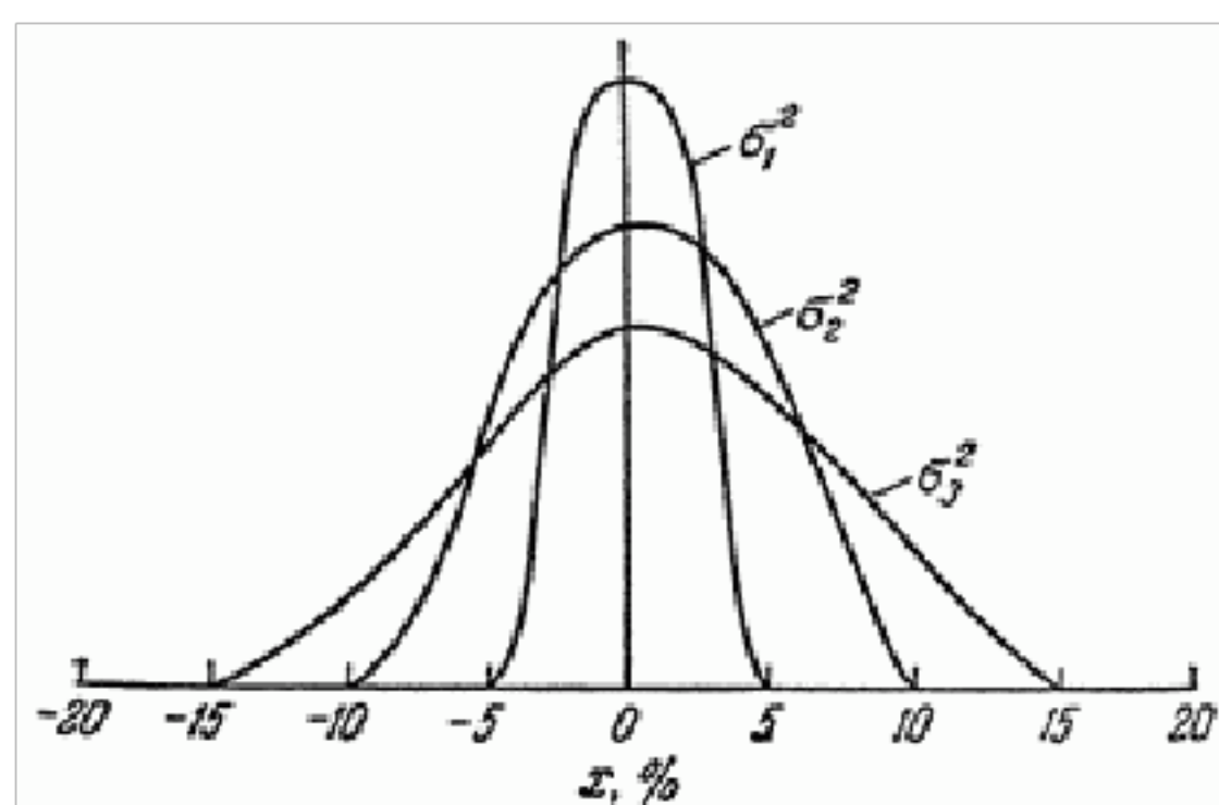
Рис. 2. Кривая Гаусса ( )
