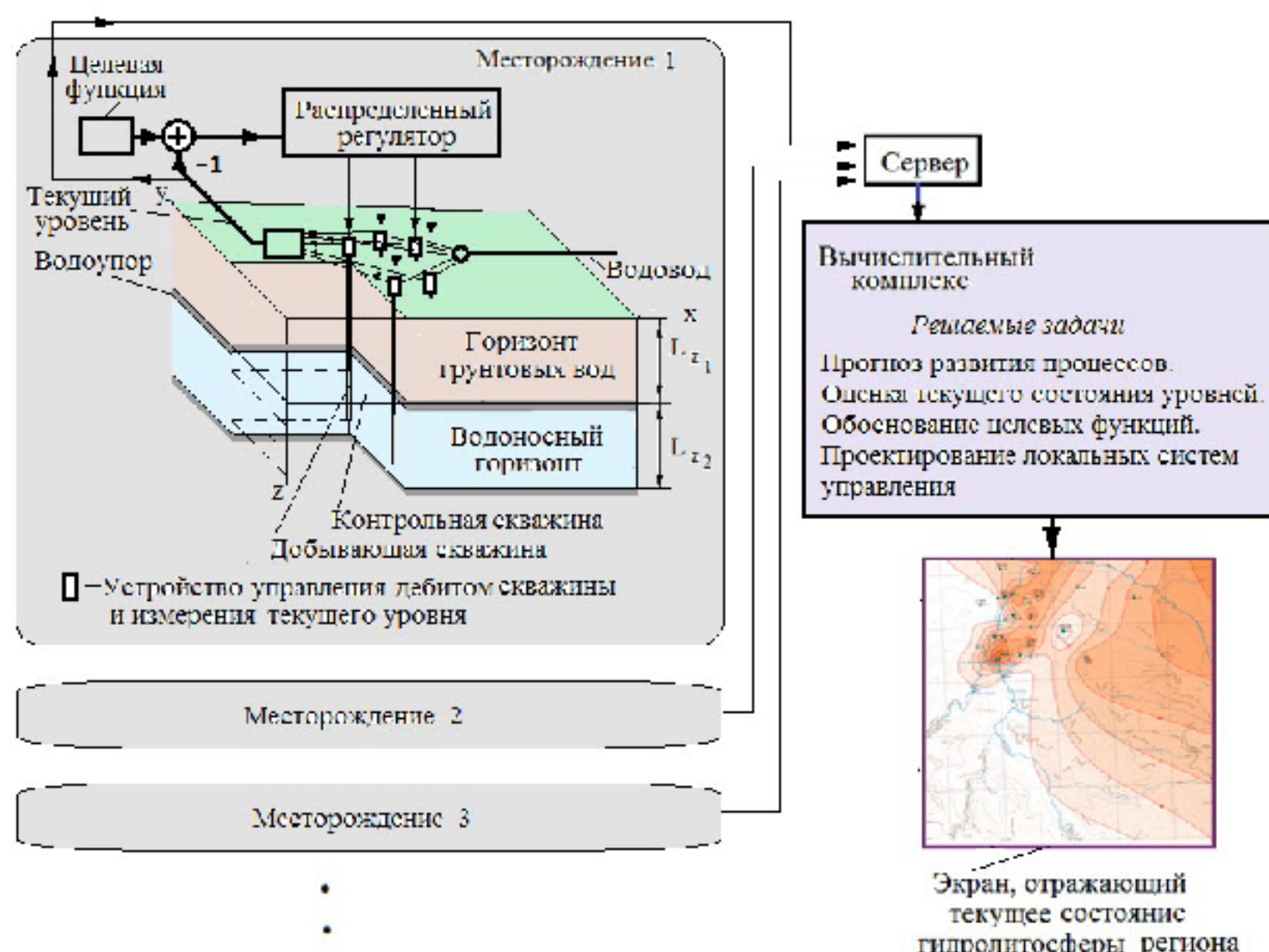
Рис.1.1. Сеть мониторинга и управления гидrolитосферными процессами региона .
