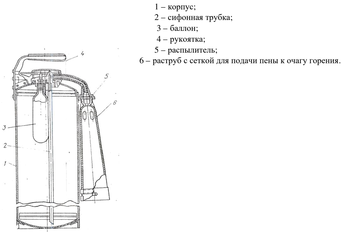
Рисунок 2 - Воздушно-пенный огнетушитель ОВП – 10
