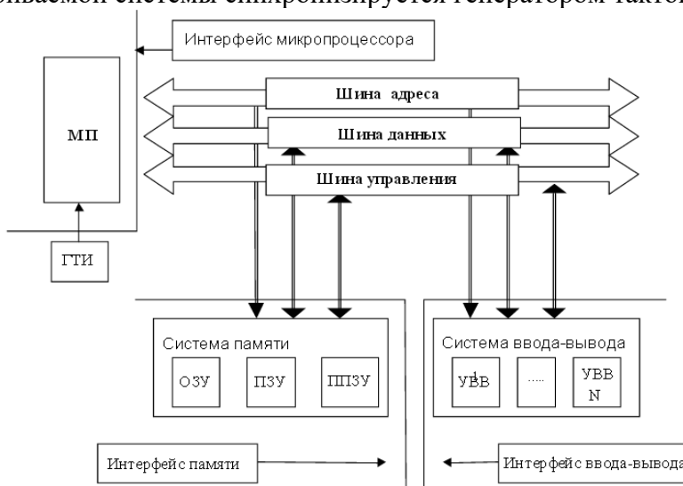
Рис. 1. Обобщенная структура МПС
