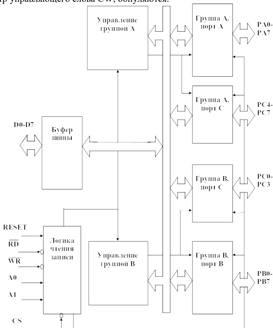
Рис. 1. Структурная схема БИС ППА К580BB55А
