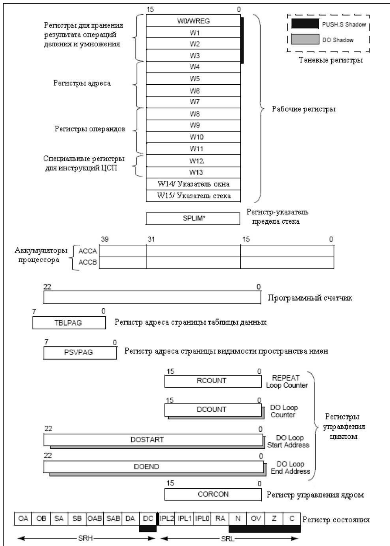
Рисунок 8 - Регистры микропроцессора
