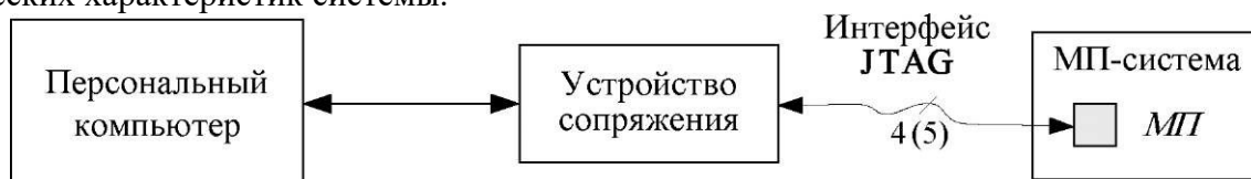
Рис. 33.3. Отладка с помощью внутрикристалльного эмулятора
