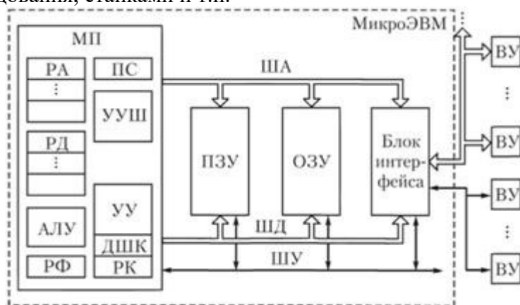
Рис. 1. Структура микропроцессорной системы
