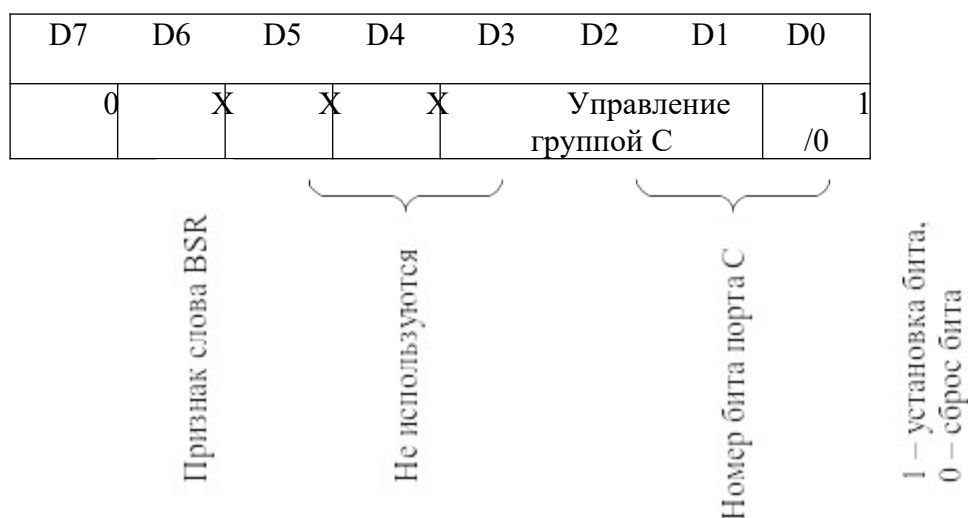
Рис. 3. Формат регистра BSR
