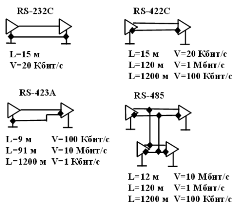
Рис.16. Стандарты последовательного интерфейса
