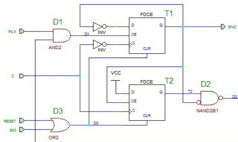
Рис. 28.1. Схема привязки сигнала SNO к тактовым сигналам
