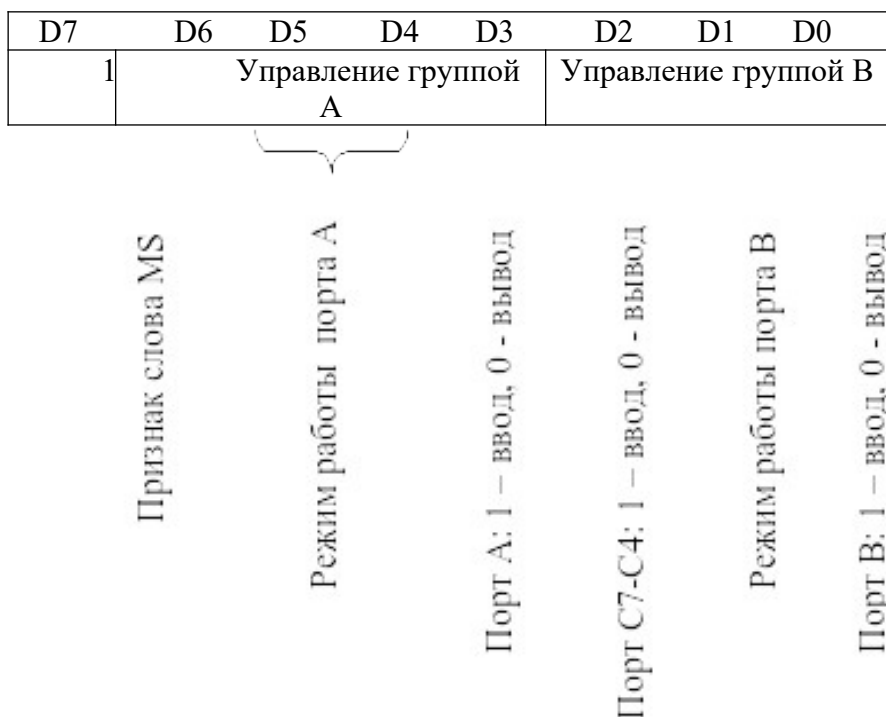
Рис. 2. Формат регистра CW
