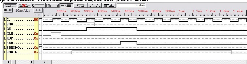
Рис. 28.2. Результаты моделирования схемы привязки сигнала SNO
