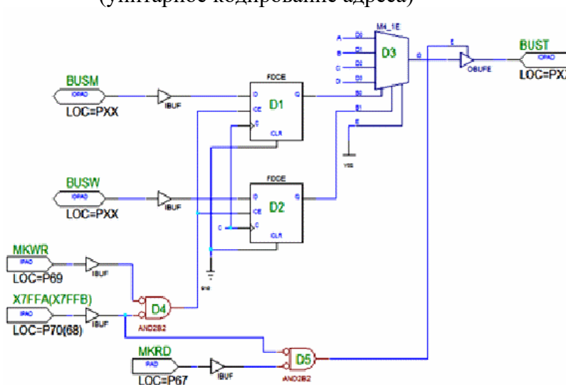
Рис. 29.8. Вариант подключения четырёх источников через мультиплексор (управление от регистра адреса)
