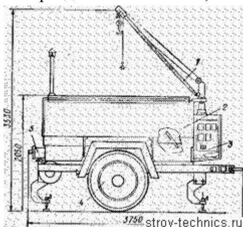
Рис. 183. Установка для варки битума передвижная УВВ-3 1 — кран-укосина; 2 — емкость; 3 — пульт управления; 4 — шасси; 5 — слив
