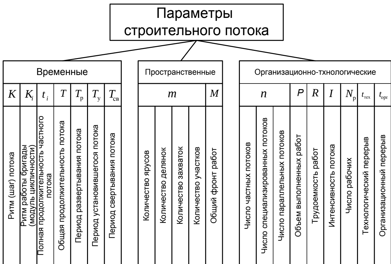
Рисунок 3.3 Классификация и обозначение параметров строительных потоков
