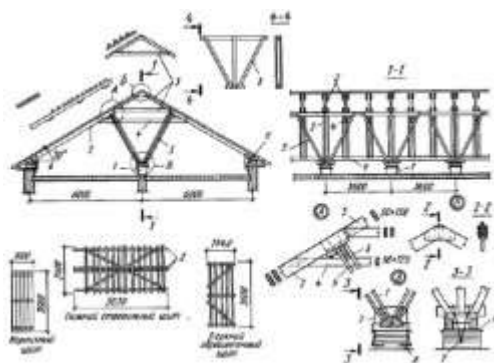
Рис. 5. Деревянные стропила промышленного типа: 1 — кирпичные или бетонные столбики, 2 — ноги стропильного щита, 3 — коньковые фермочки, 4 — схватка, 5 — опорные фермы, 6 — мауэрлат, 7 — проволочная скрутка, 8 — ерши, 9 — два слоя толя
