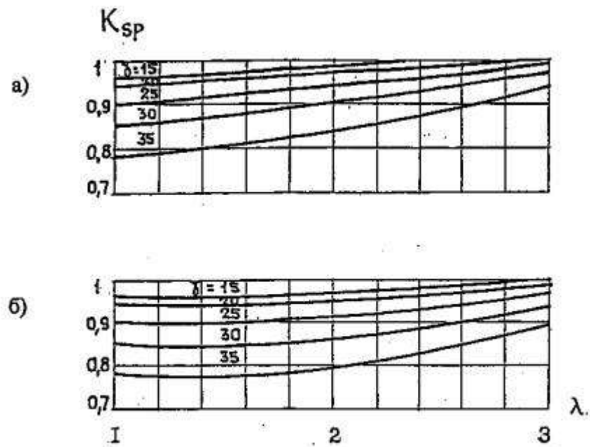
Рис. 3. Зависимости коэффициента K_{sp} от \lambda и \gamma в плитах, опертых по контуру; а - при равномерном армировании; б - с концентрацией арматуры A_{sl} у центра с коэффициентом \varphi_c = a_{s11}/a_{s12} = 2 ; \lambda = l_2/l_1 ; \gamma = l_1/h
