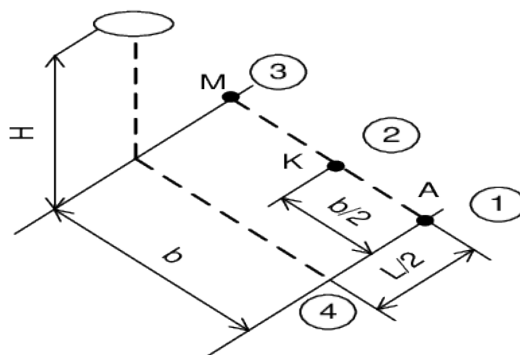
Рис.16. Иллюстрация к определению координат контрольных точек
