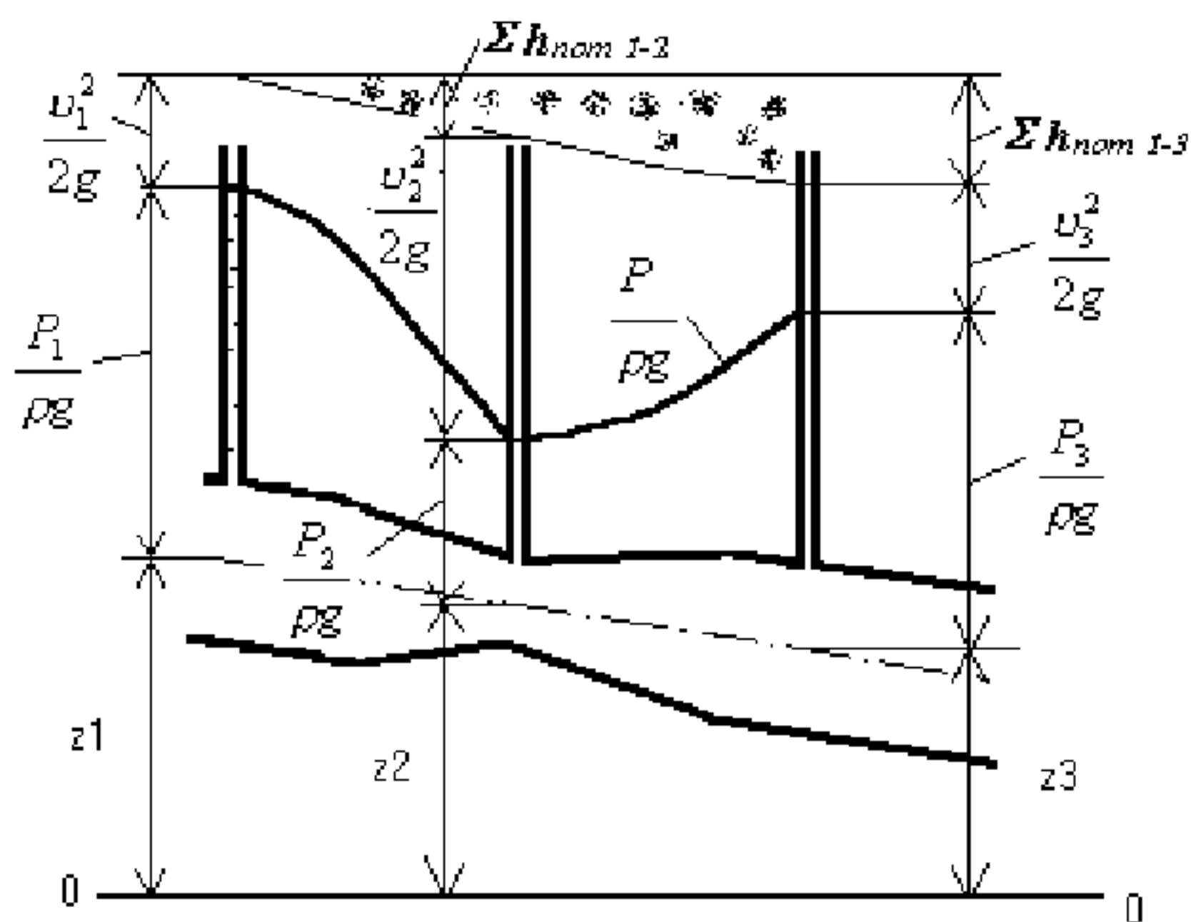
Рис. 1.6. 2. Графическая интерпретация закона Бернулли
