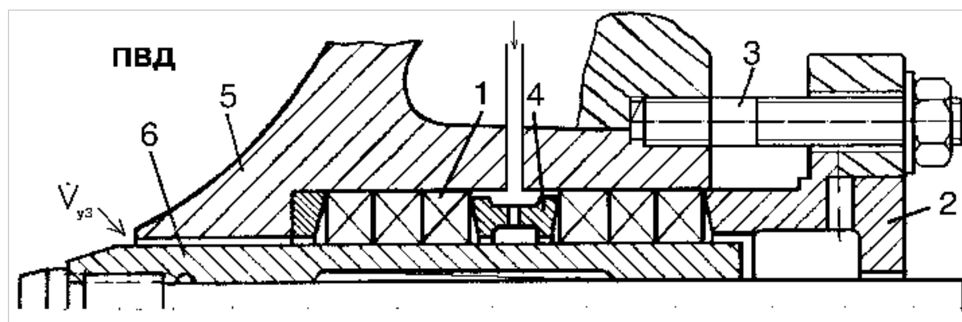
Рис. 2. Сальник
