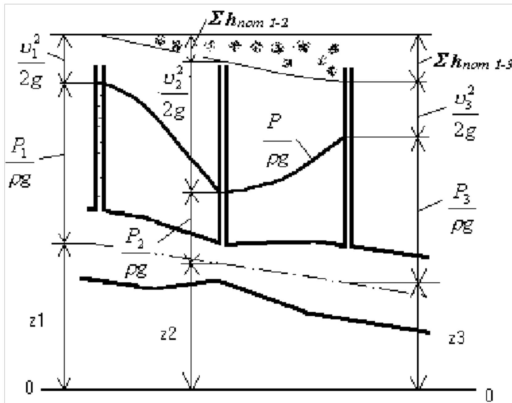
Рис. 1.6. 2. Графическая интерпретация закона Бернулли. Энергия, теряемая жидкостью на рассмотренном участке течения, разумеется не теряется бесследно, а лишь превращается в другую форму – тепловую, которая непрерывно рассеивается, поэтому повышение температуры бывает практически незаметным.
