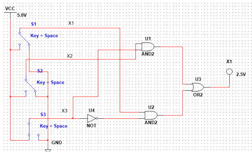
Рисунок 2 - Комбинационная схема
