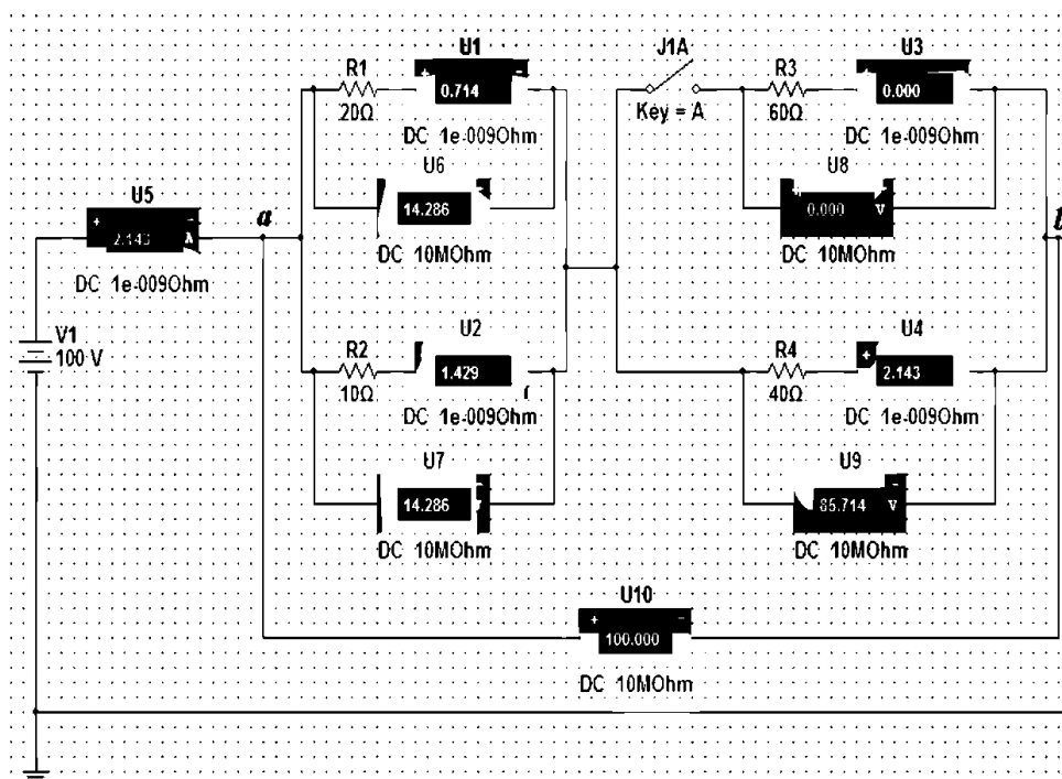
Рисунок 2.1 – Схема цепи
