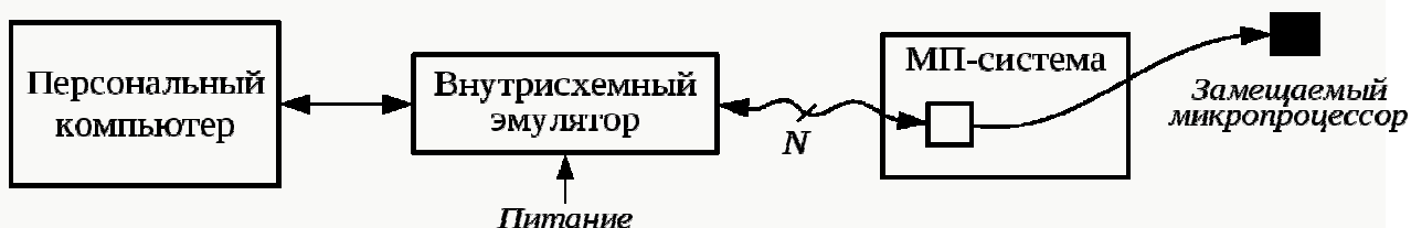
Рисунок 16.2 – Отладка с помощью внутрисхемного эмулятора
