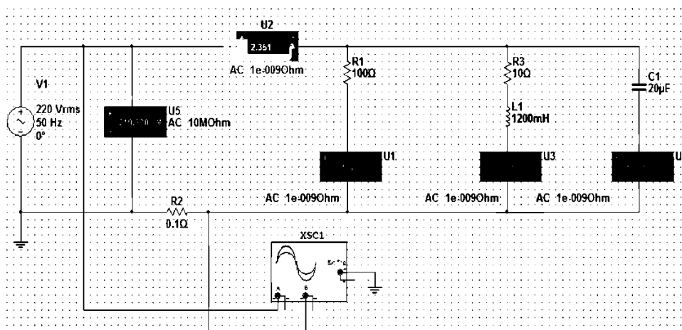
Рис. 3.6. Схема цепи с параллельным соединением резистора, катушки и конденсатора
