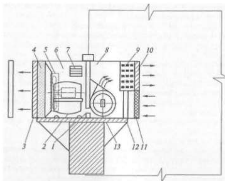
Рис. 1. Схема устройства кондиционера оконного типа:
