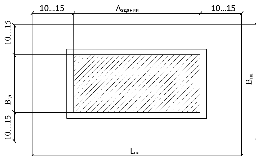
Рисунок 2.2-План площадки
