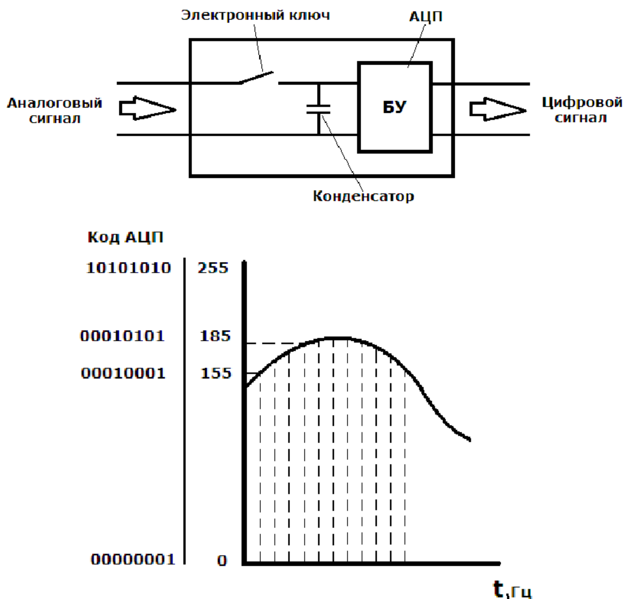
Рис. 2. Принципиальная схема АЦП.
