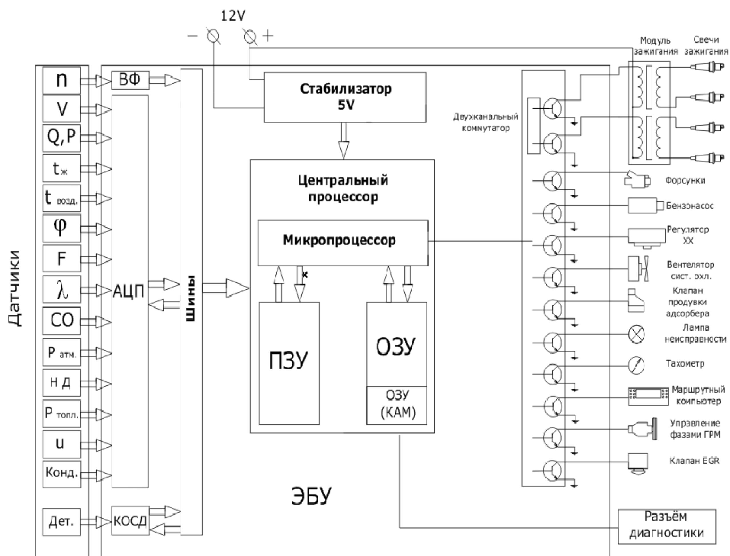
Рис 1. Блок-схема управления впрыском топлива и зажигания:
