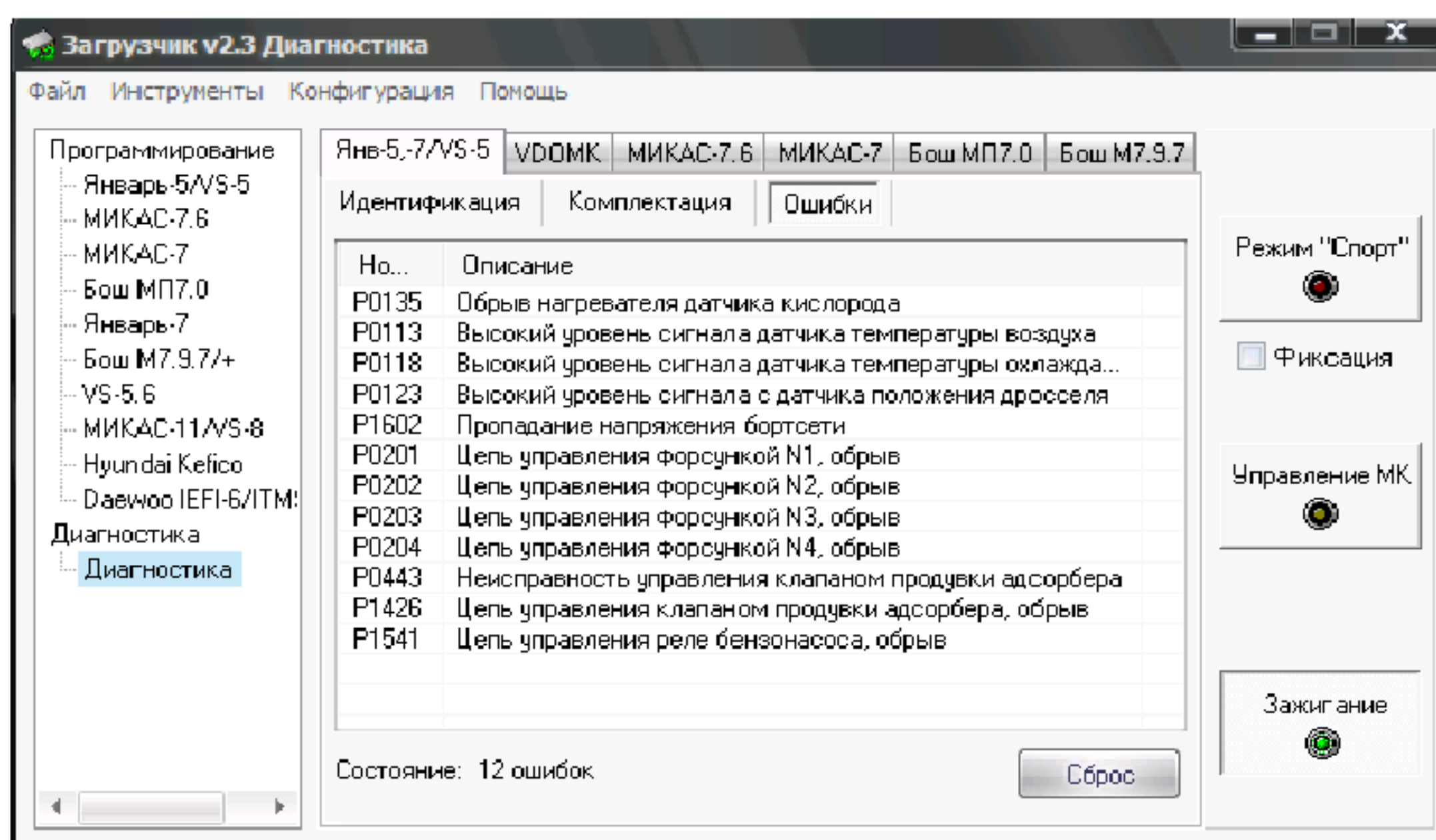
Рис. 14. Ошибки - просмотр и сброс кодов неисправностей
