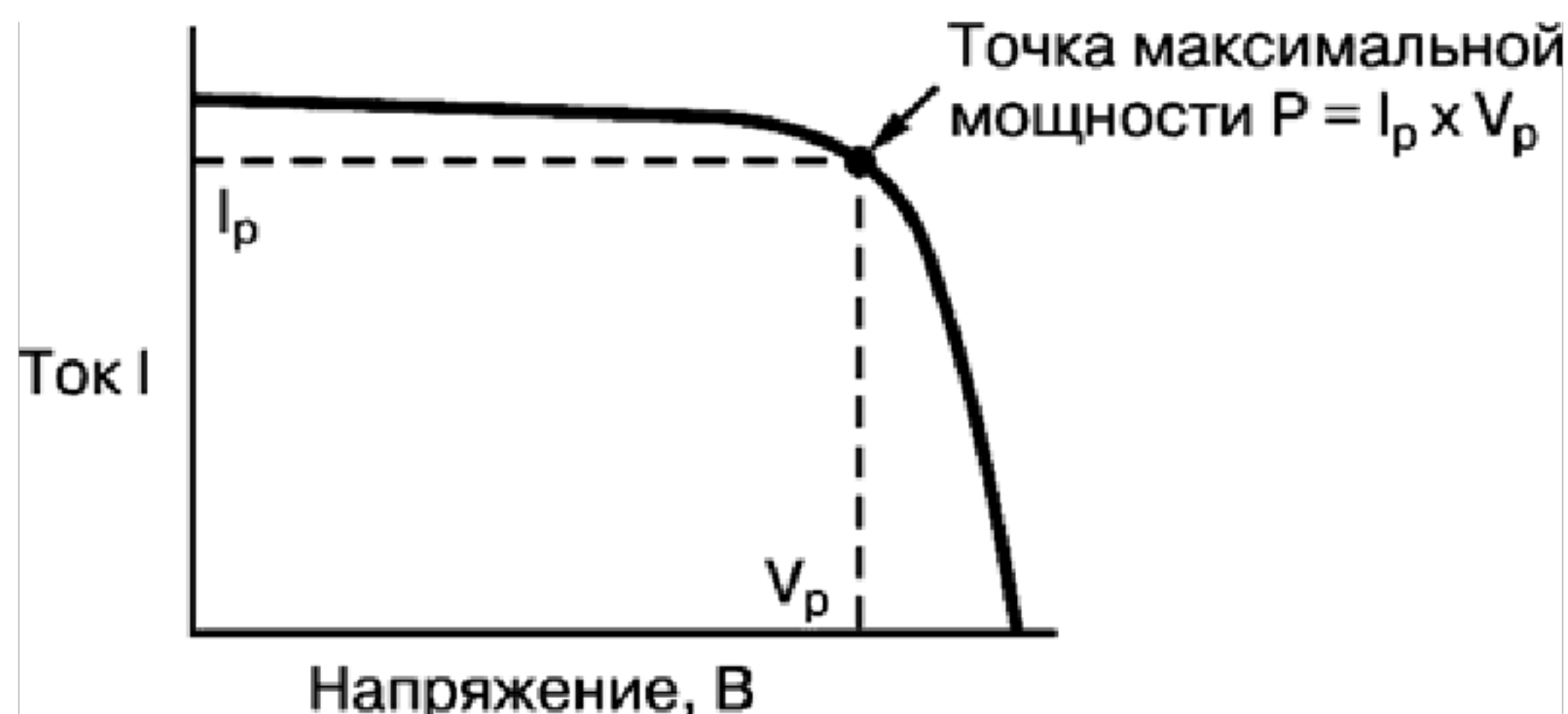
Рисунок 2 – Вольт-амперная характеристика фотоэлемента
