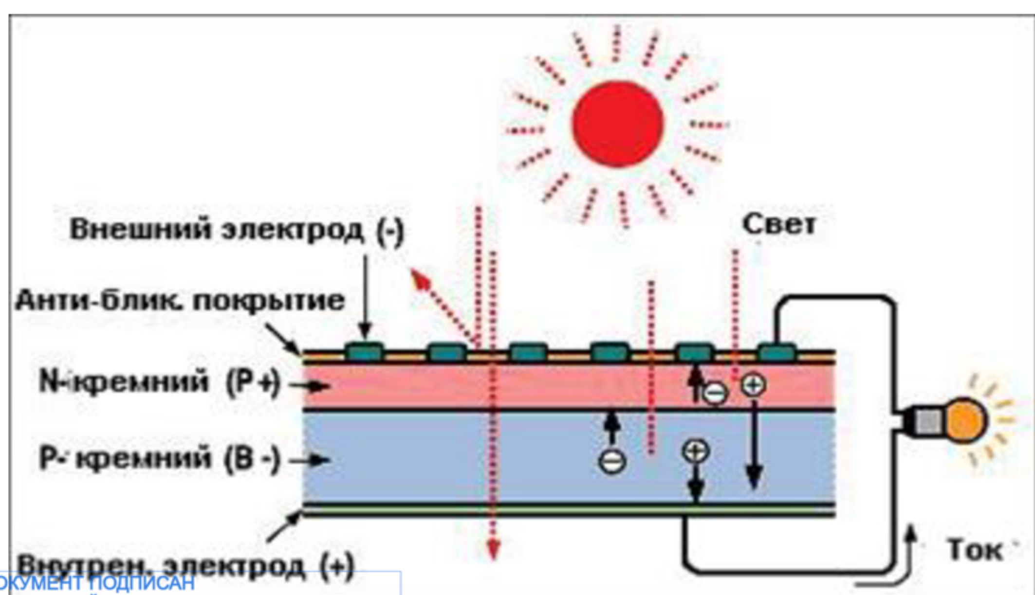
Рисунок 1 – Простейшая конструкция фотоэлектрического элемента
