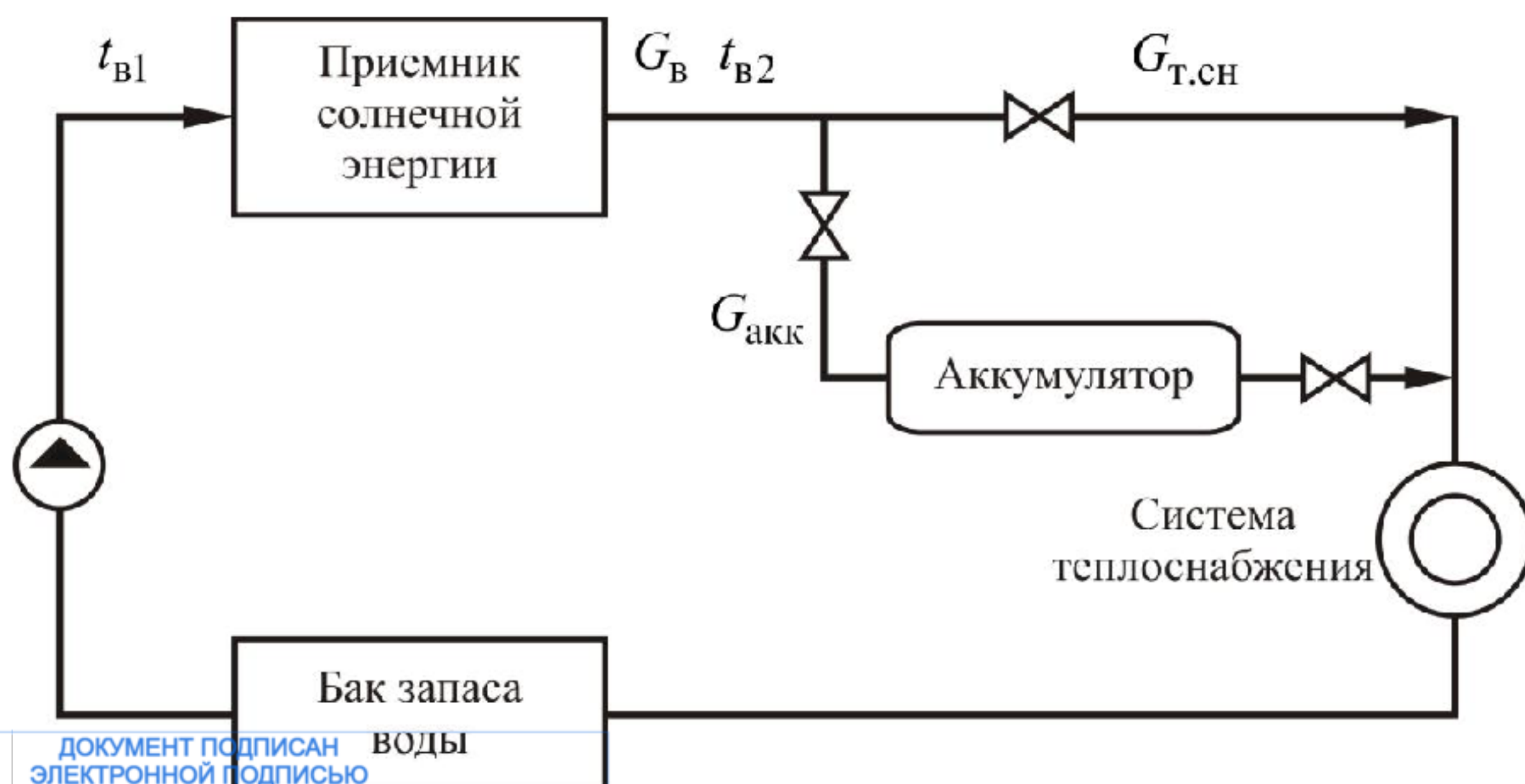
Рисунок 3 – Принципиальная схема системы солнечного теплоснабжения здания
