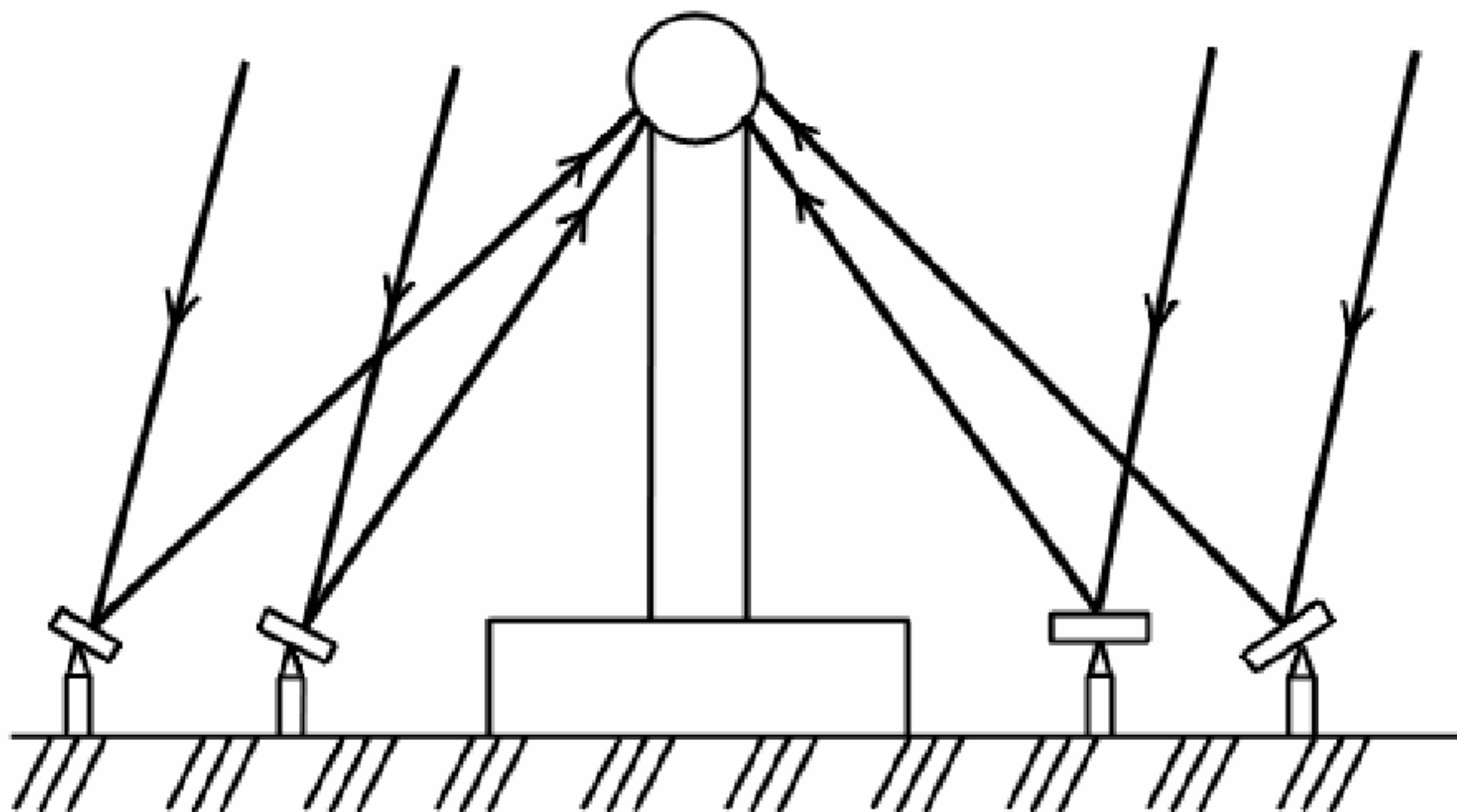
Рисунок 8 – Схема СЭС башенного типа
