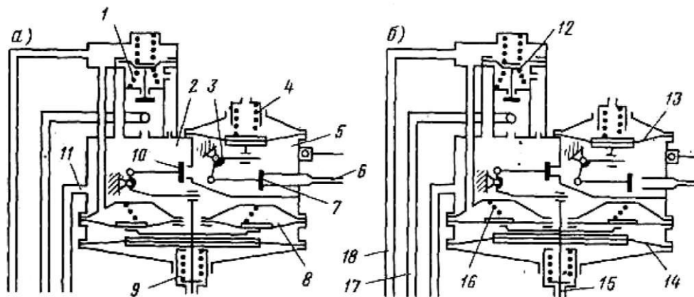
Схема работы двухступенчатого редуктора
