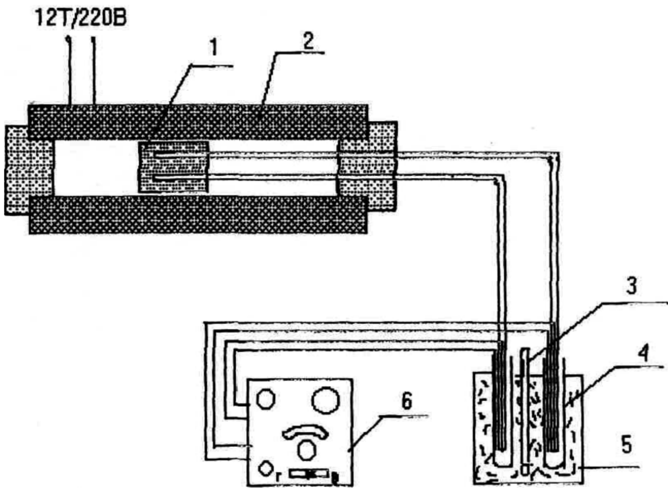
Рисунок 4 – Металлический блок
