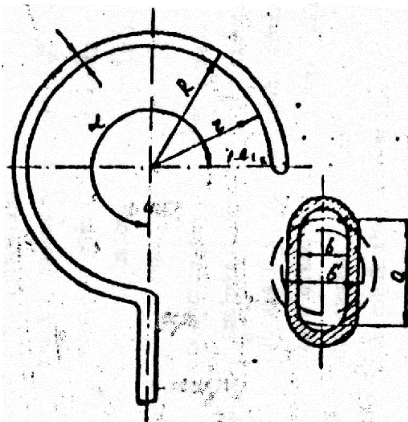
Рисунок 2 – Трубчатая пружина
