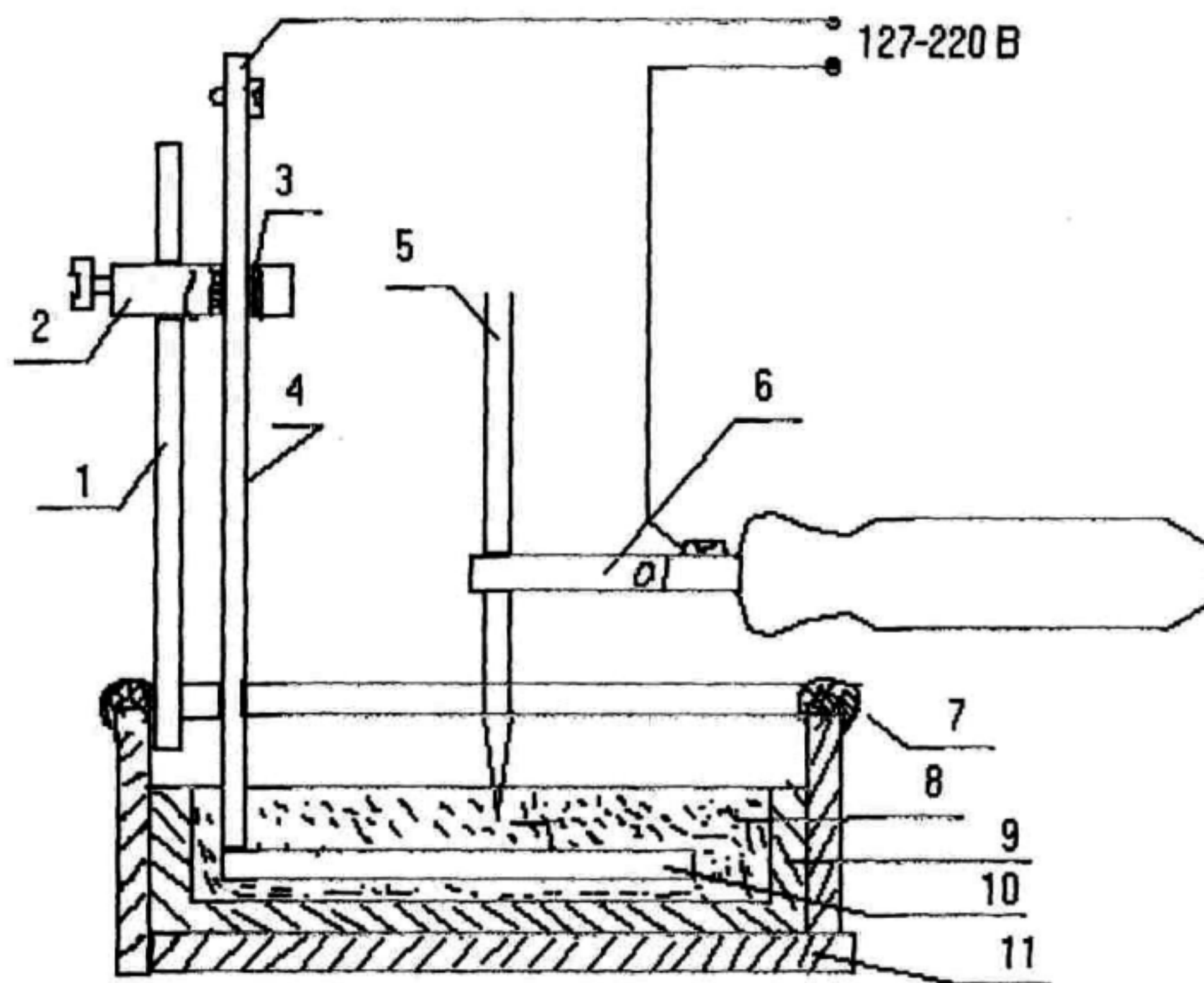
Рисунок 3 – Специальное устройство
