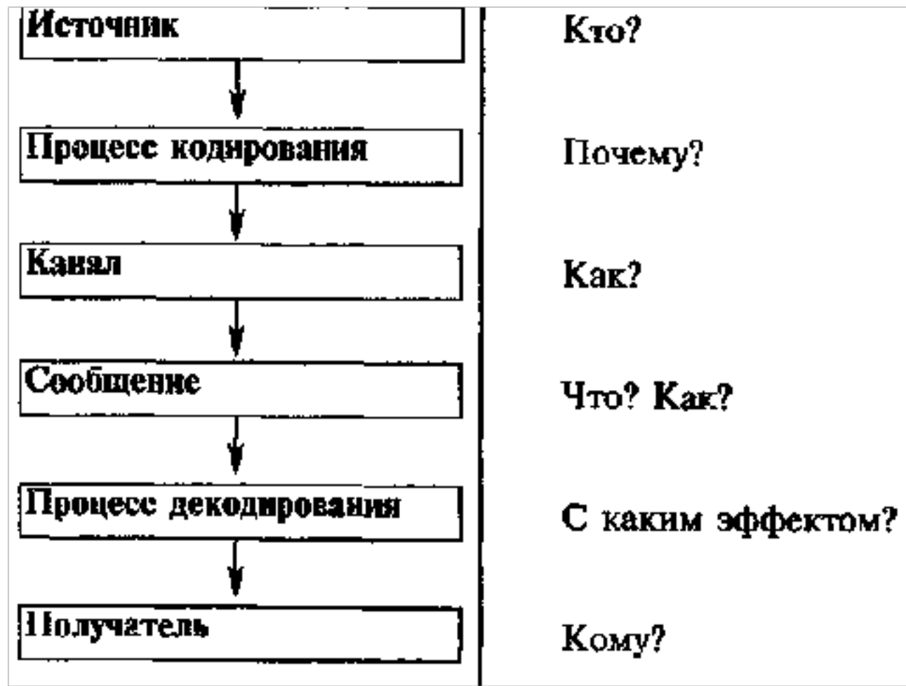
Рис.2.3 Модель контент-анализа
