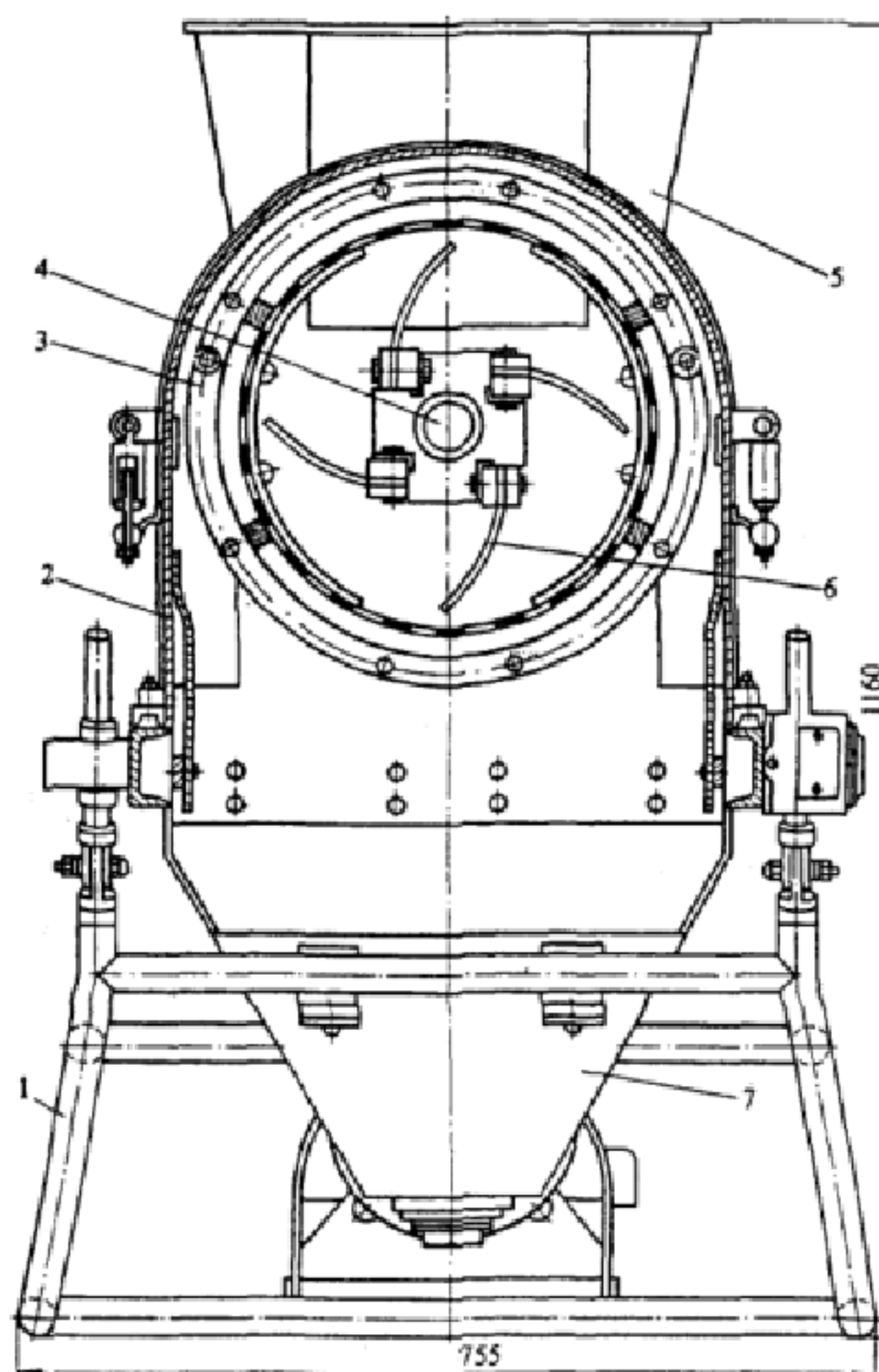
Рисунок 1.2 - Протирочная машина:
