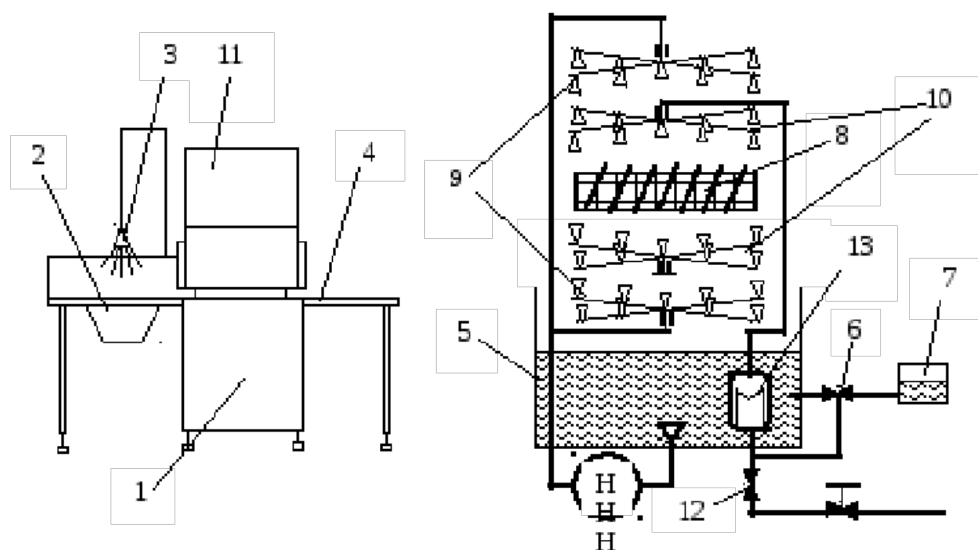
Рисунок 5.1 - Схема капотной посудомоечной машины
