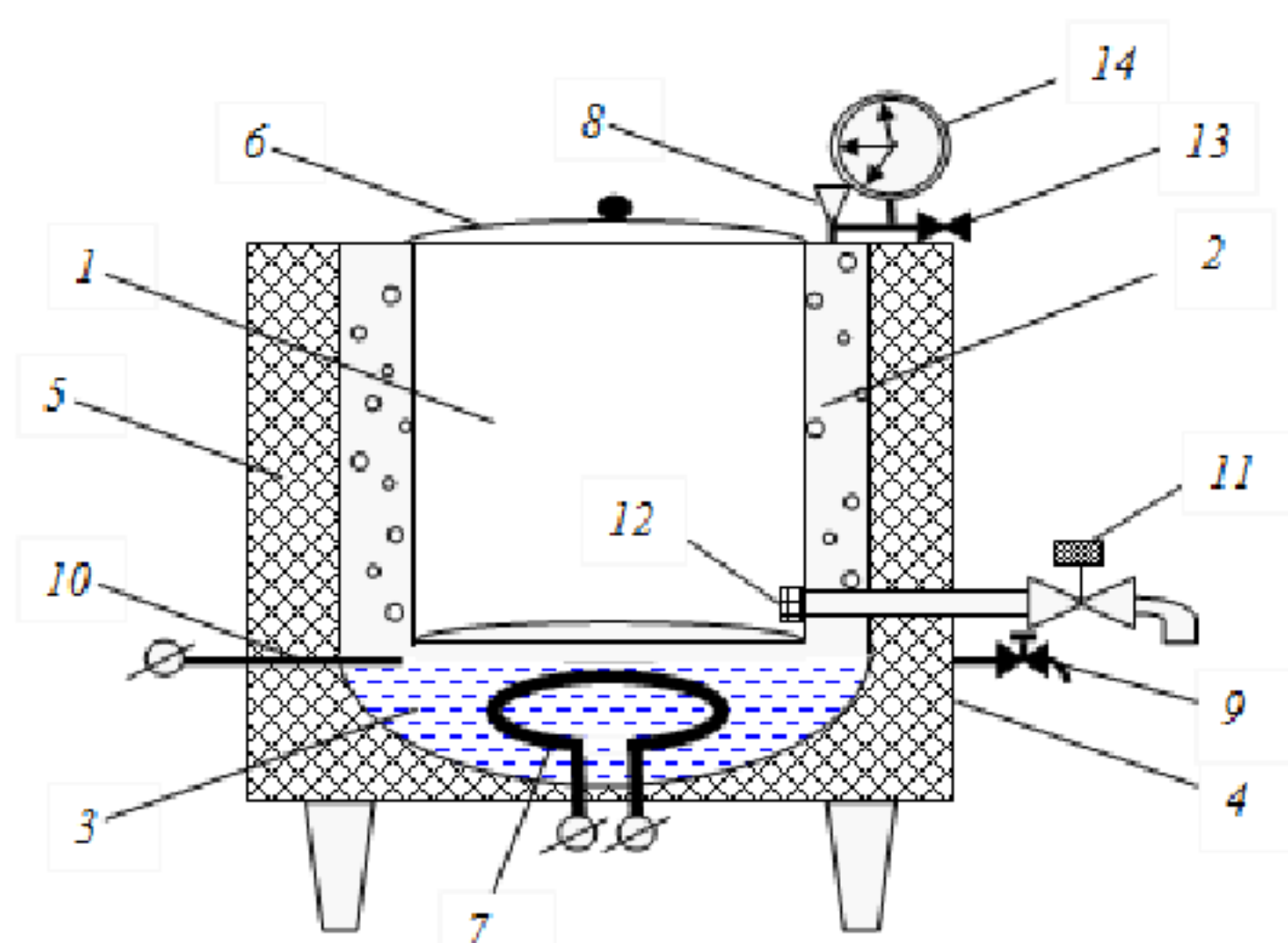
Рис. 7.2 - Схема электрического пищеварочного котла
