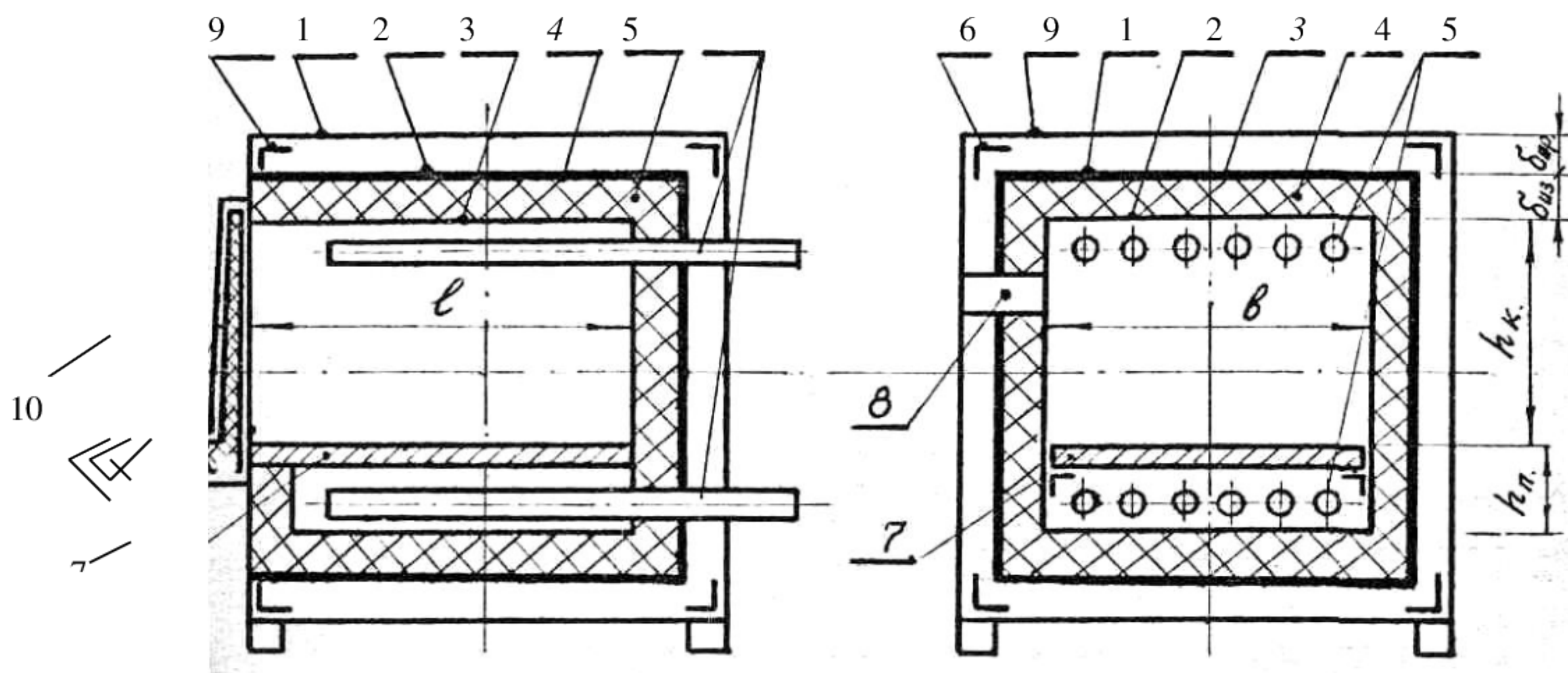
Рисунок 9.7 - Схематический разрез пекарного шкафа.
