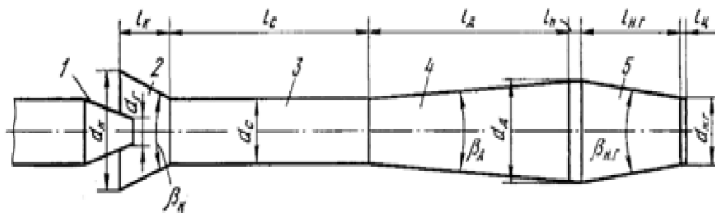
Рисунок 6.7 – Расчетная схема инжекционной горелки:
