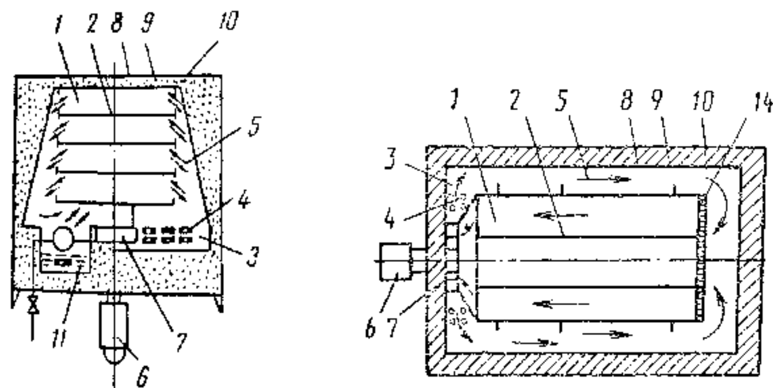
Рисунок 9.2 – Принципиальные схемы шкафов
