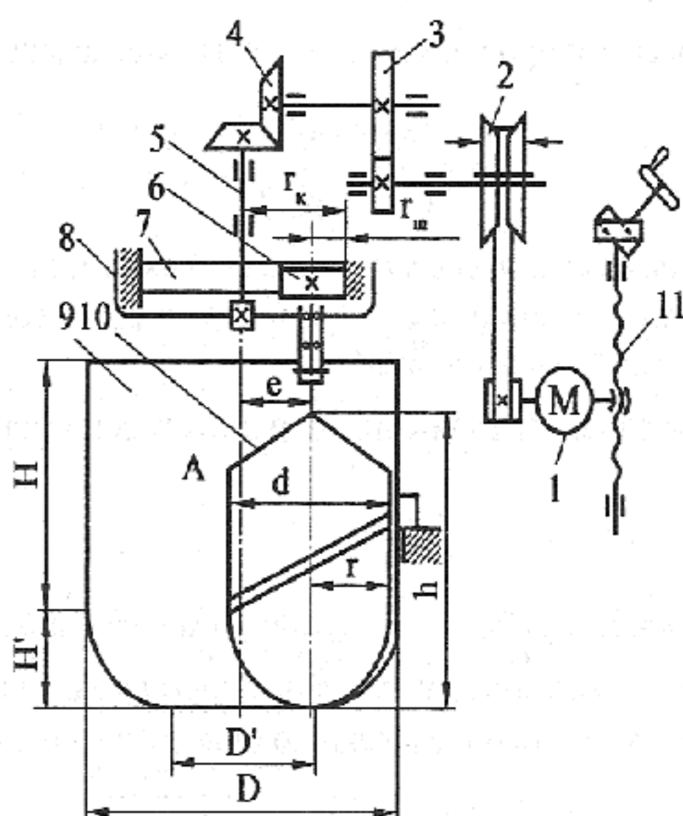
Рисунок 7.2 - Расчётная схема взбивальной машины типа MB-6:
