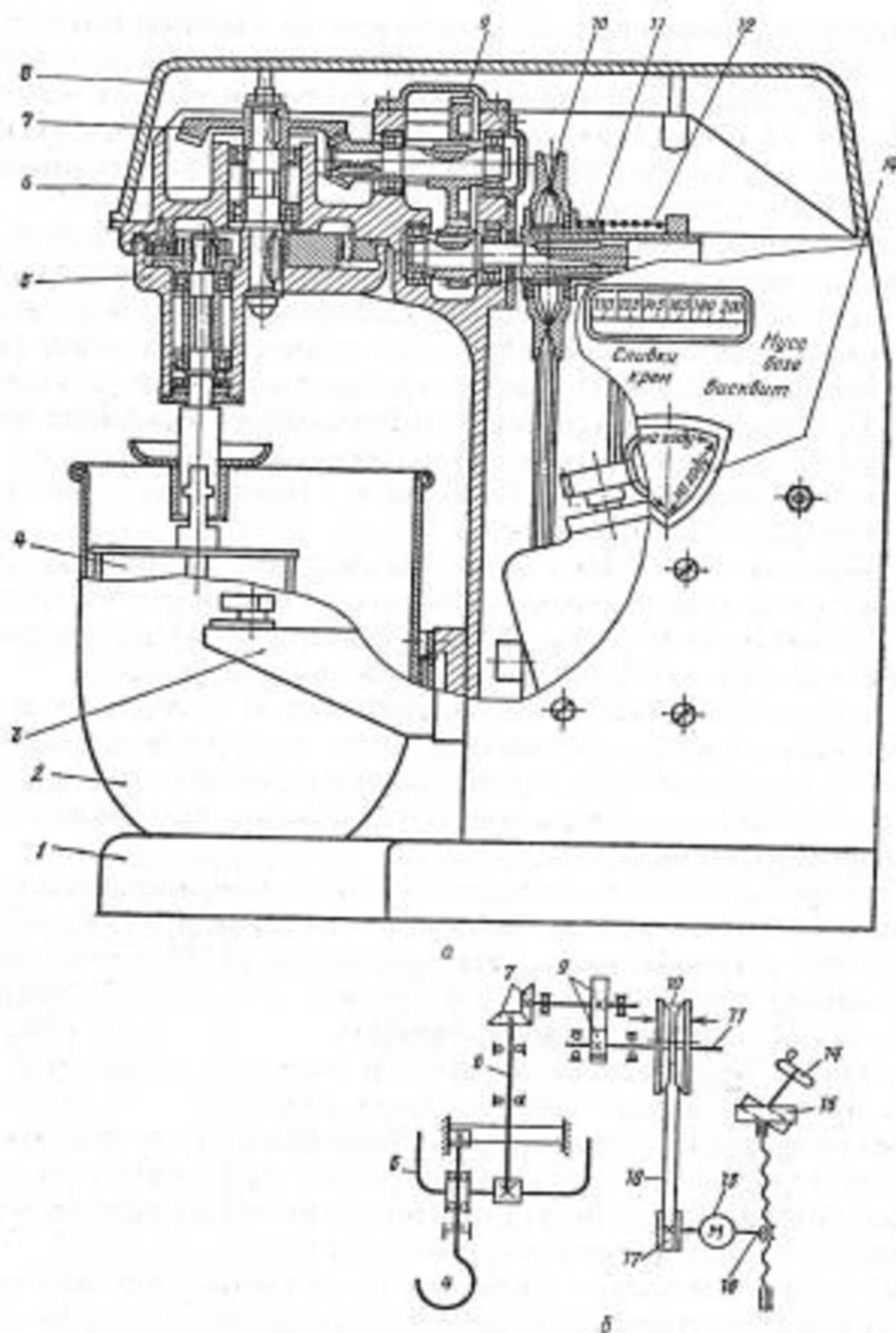
Рисунок 4 1 - Взбивальная машина МВ-6:
