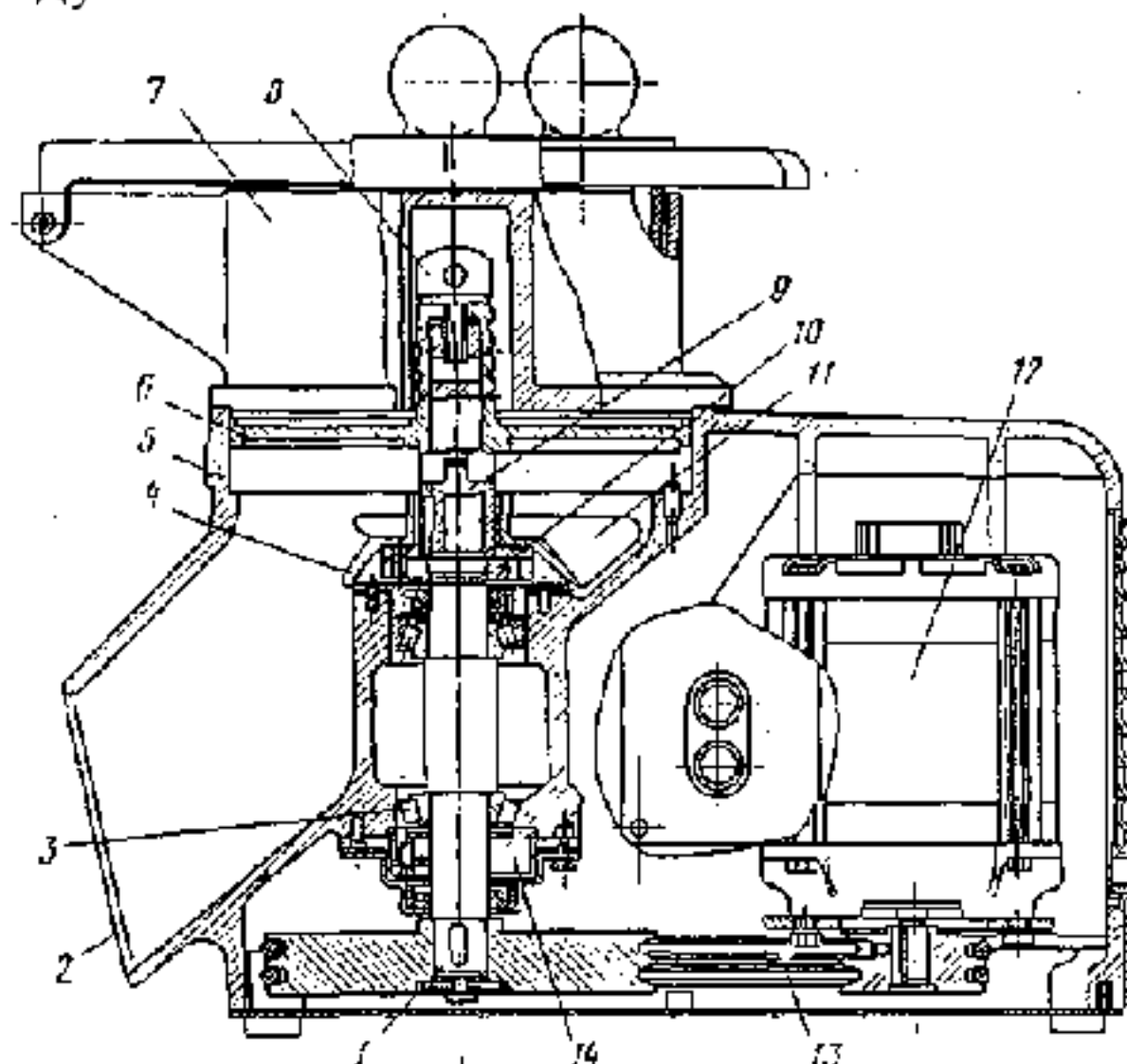
Рисунок 2.7 - Универсальная овощерезательная машина МРО 50-200
