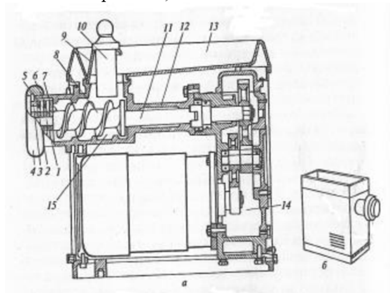
Рисунок 3.1 - Мясорубка МИМ-300
