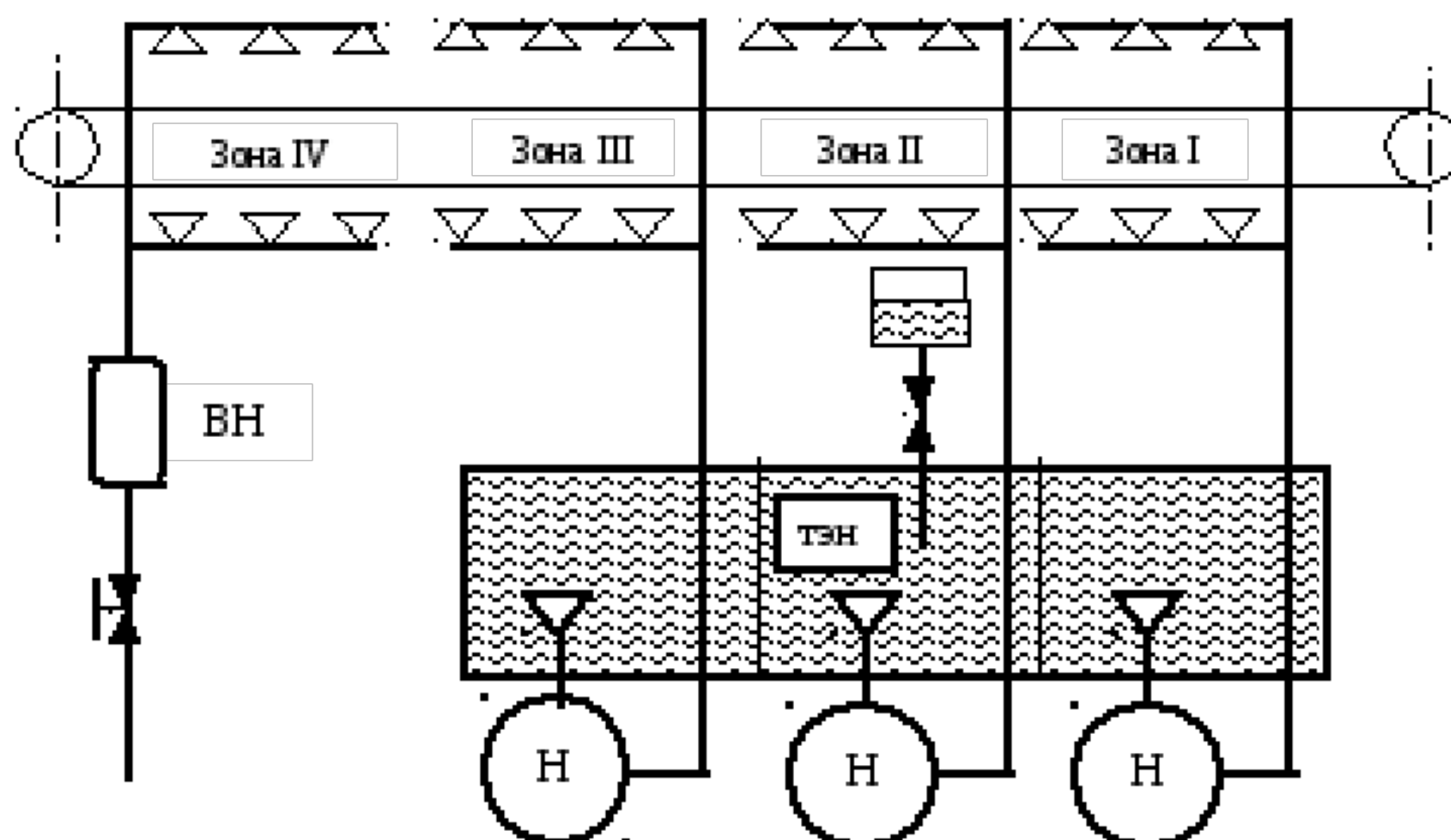
Рисунок 5.2 - Схема посудомоечной машины туннельного типа.
