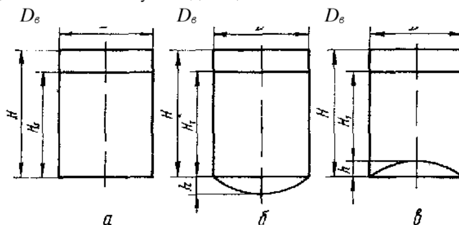
Рисунок 7.4 - Конфигурация варочных сосудов:
