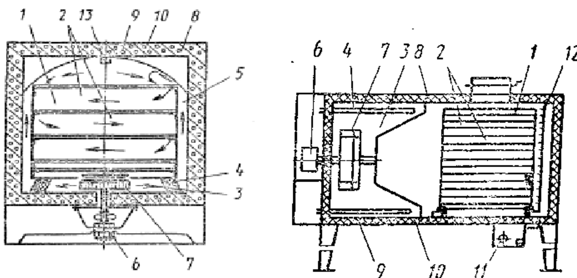
Рисунок 9.1 – Принципиальные схемы шкафов
