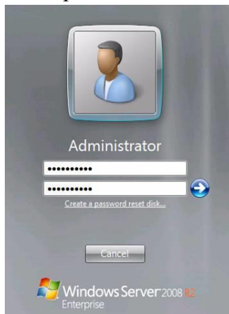
Рисунок 16. Подтверждение пароля
