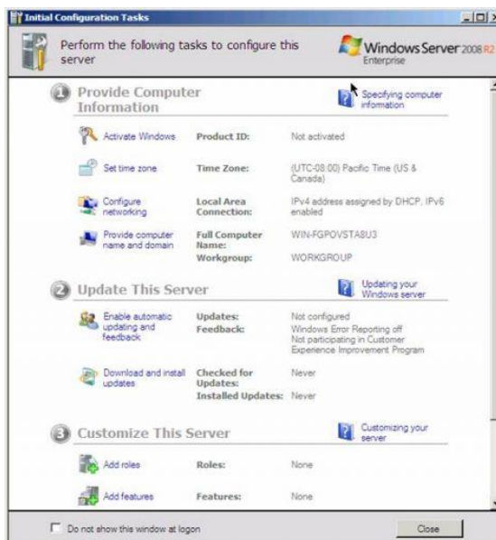
Рисунок 18. Настройки
