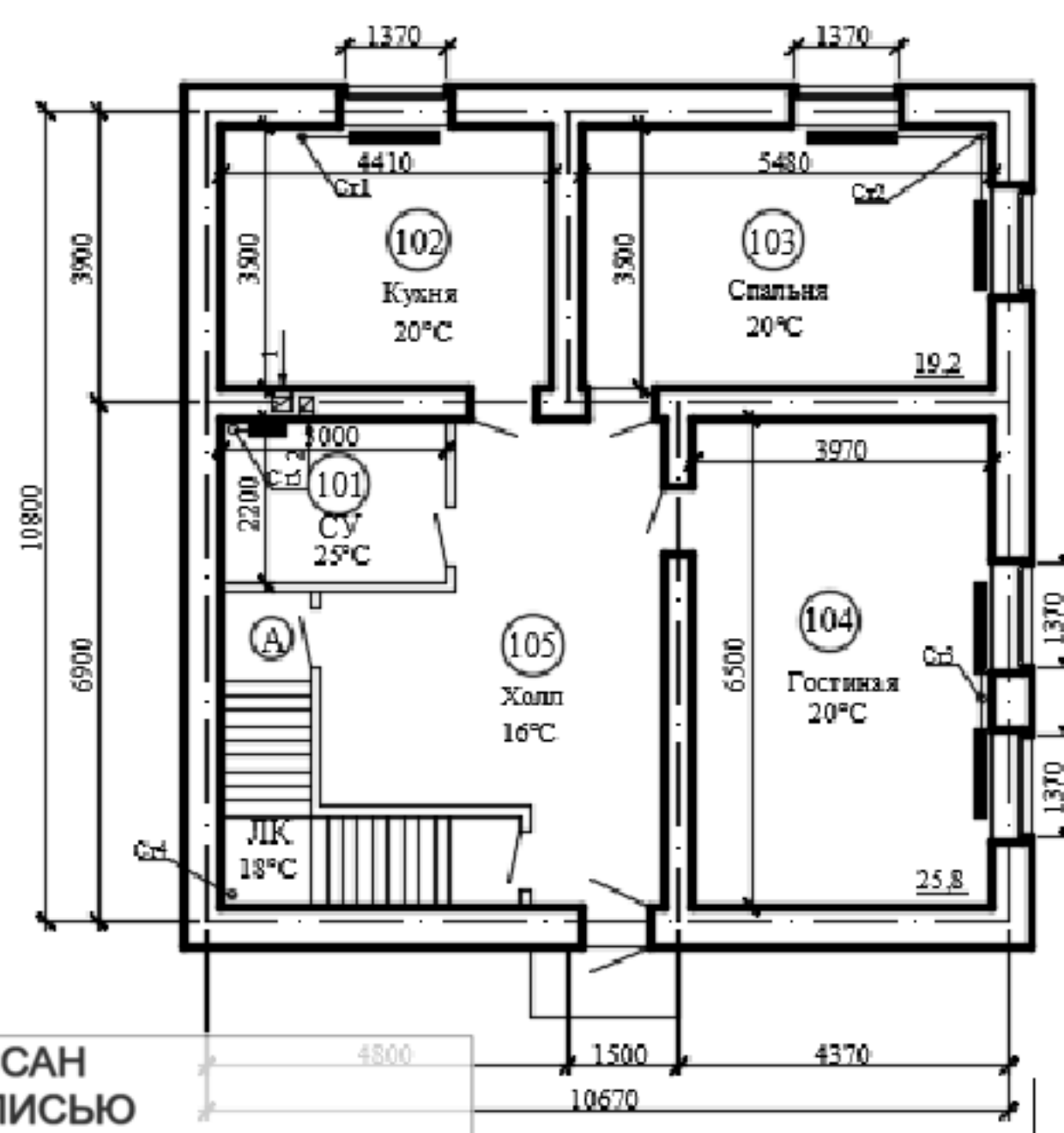
Рисунок 4.2 – План первого этажа двухэтажного жилого дома
