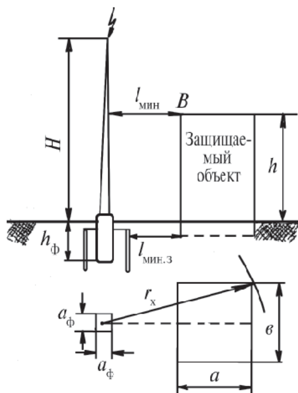
Рисунок 2 – Схема расположения молниеотвода и защищаемого объекта
