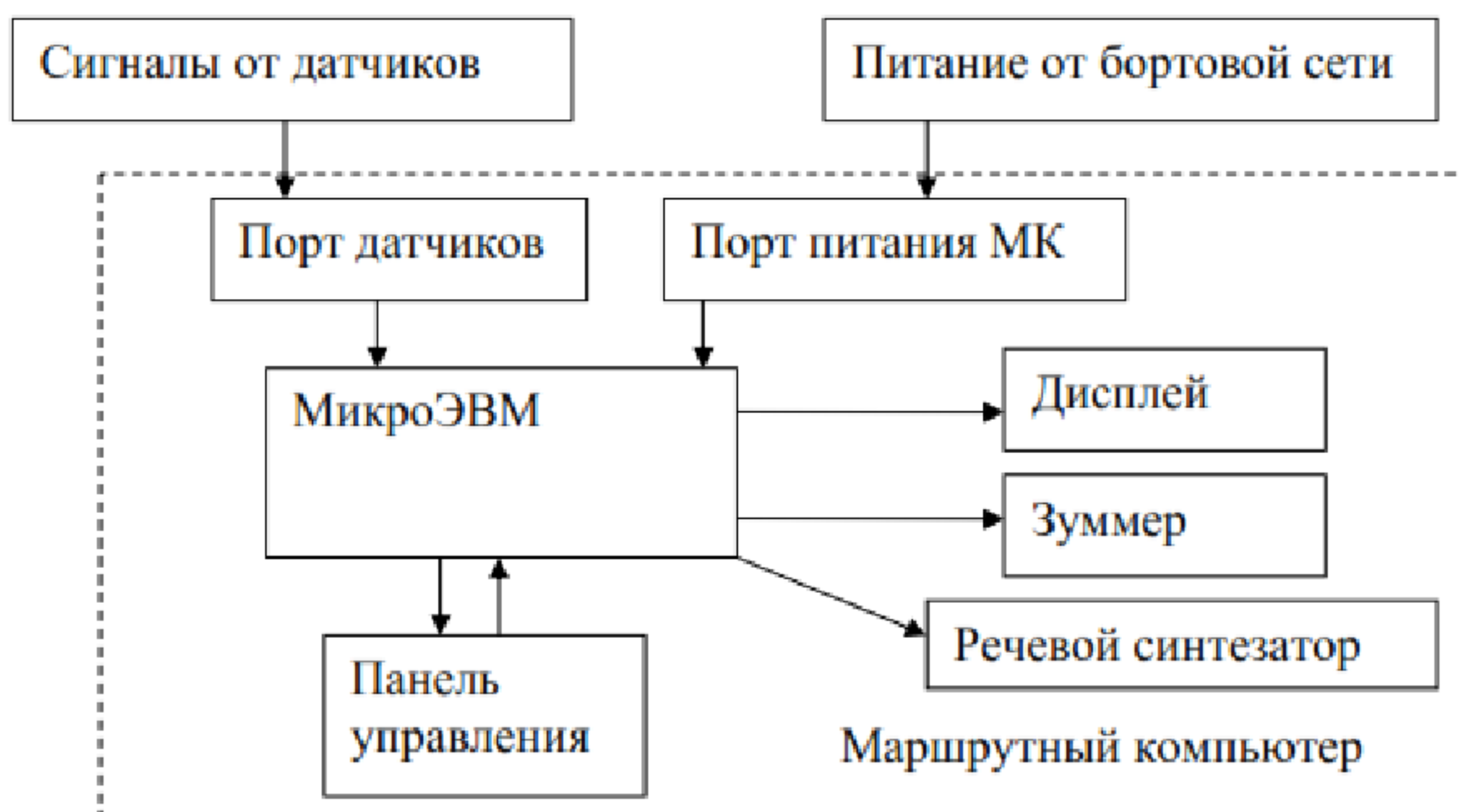
Рисунок 3 - Структурная схема автомобильного маршрутного компьютера
