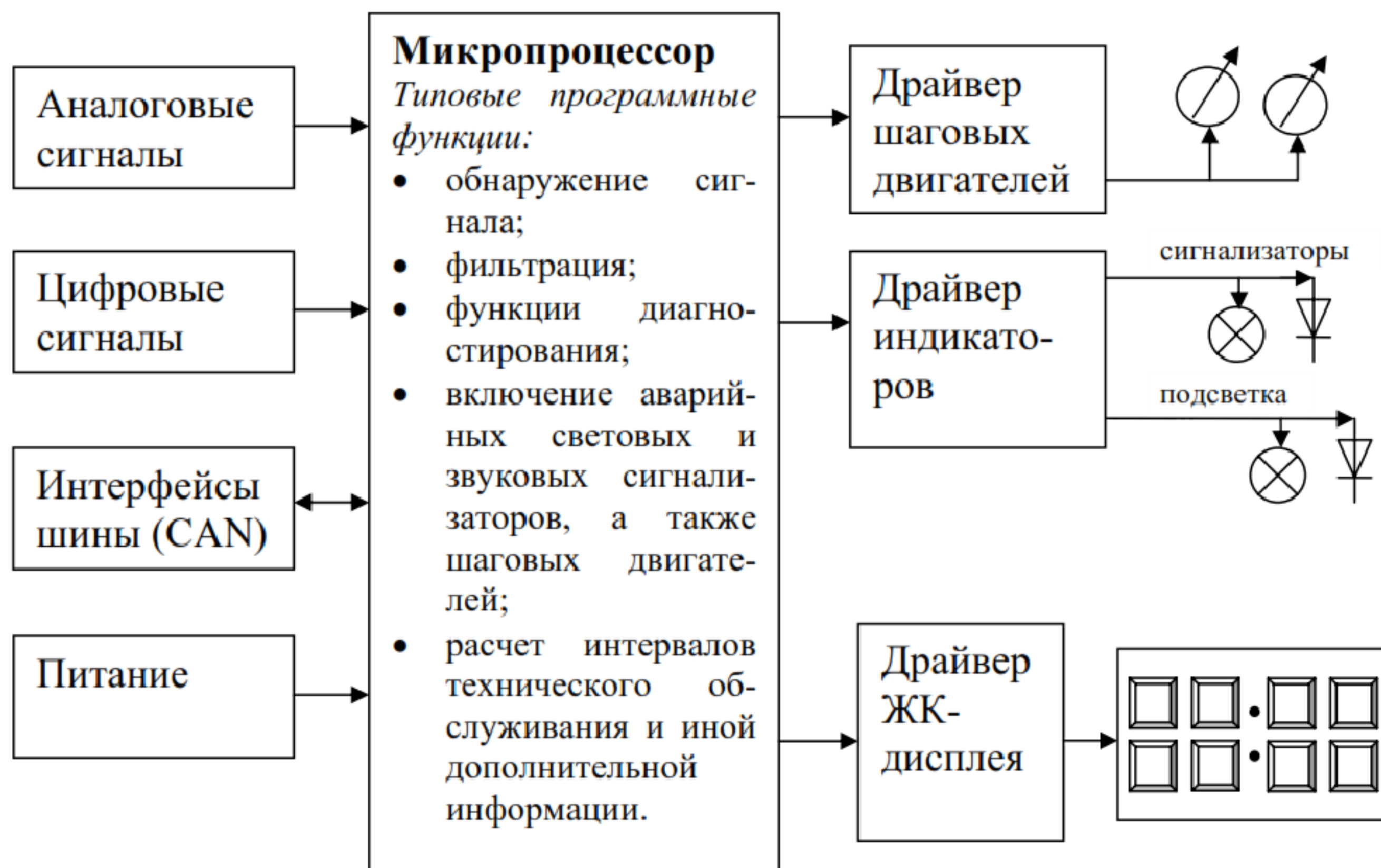
Рисунок 6 - Блок-схема электронной приборной панели с применением микропроцессора
