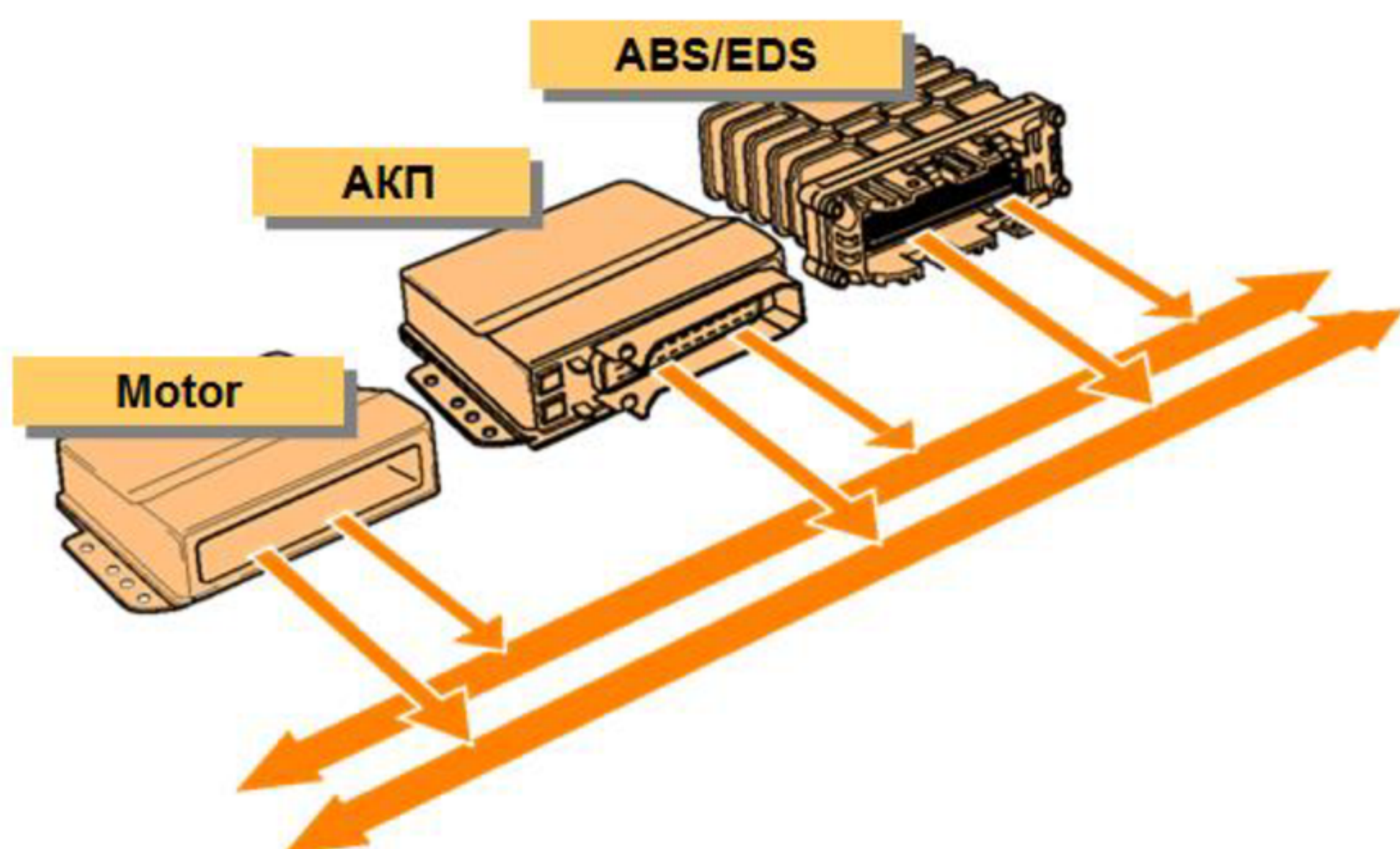
Рисунок 4 – Подключение блоков управления к двухпроводной шине CAN
