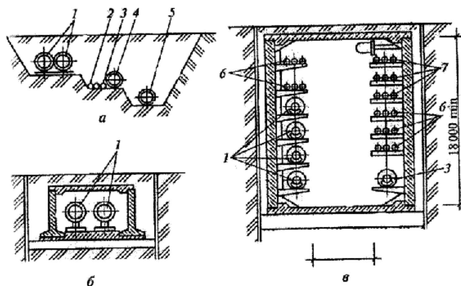
Рис. 2. Способы размещения инженерных сетей: а) в общей траншее; б) в непроходном коллекторе; в) в проходном коллекторе; 1 – теплосеть; 2 – газопровод; 3 – водопровод; 4 – водосток; 5 – канализация; 6 – кабели связи; 7 – силовые кабели.
