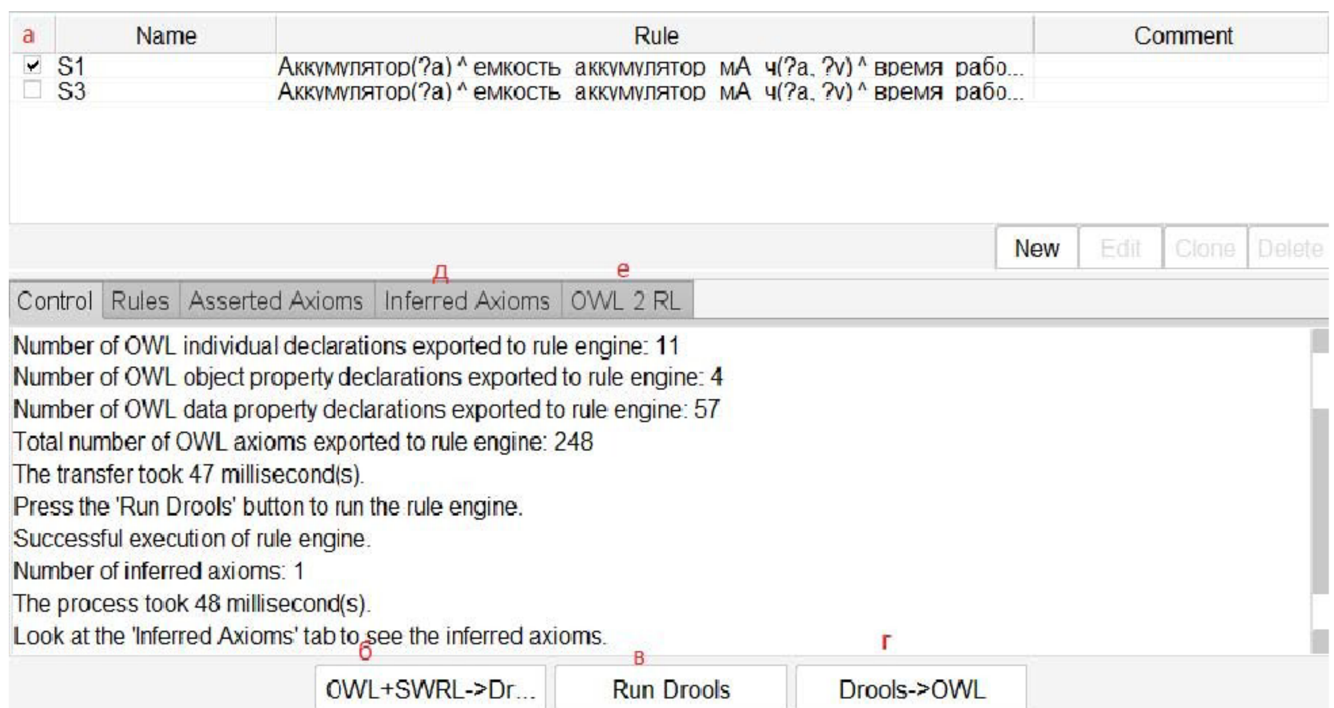
Рис. 26 Вкладка SWRL в системе Protégé (а – активность правила; б – кнопка запуска правила; в – загрузка понятий из онтологии и списка правил; г – запуск вывода на основе правил; д – внесение выведенных понятий в онтологию; е – список правил)
