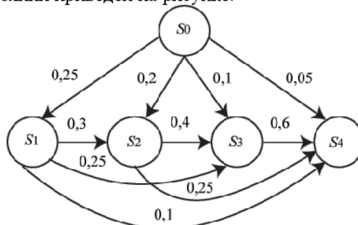
Размеченный граф состояний четырех объектов
