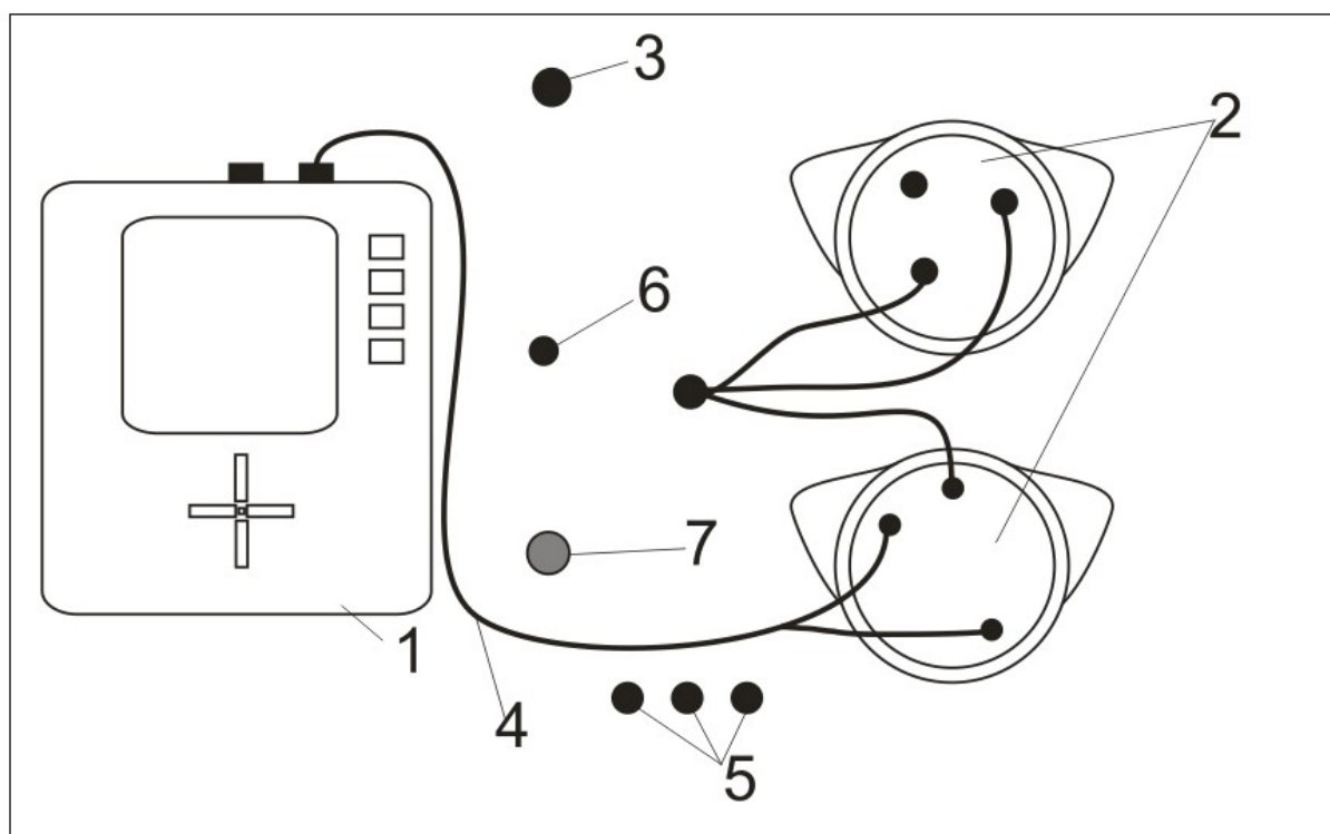
Рис. 1. Схема лабораторной установки для испытания генераторов: 1 – осциллограф; 2 – генераторы; 3 – лампа индикатор включения питания генератора; 4 – кабель второго канала осциллографа; 5 – выключатели имитаций неисправностей; 6 – лампа нагрузки; 7 – выключатель питания; 8 – мультиметр.
