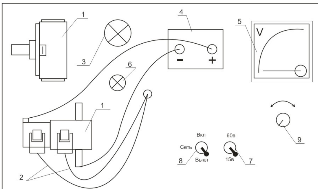
Рис. 3. Схема лабораторной установки для испытания регуляторов напряжения: 1 – регуляторы напряжения; 2 – выводы контрольной лампы; 3 – контрольная лампа включения питания; 4 - контактная площадка блока питания; 5 – вольтметр; 6 – контрольная лампа; 7 – переключатель режима вольтметра; 8 – выключатель питания; 9 – регулятор напряжения.
