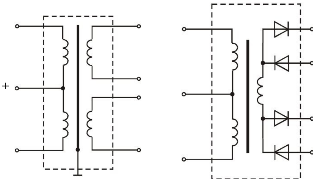
Схемы четырехвыводных катушек зажигания
