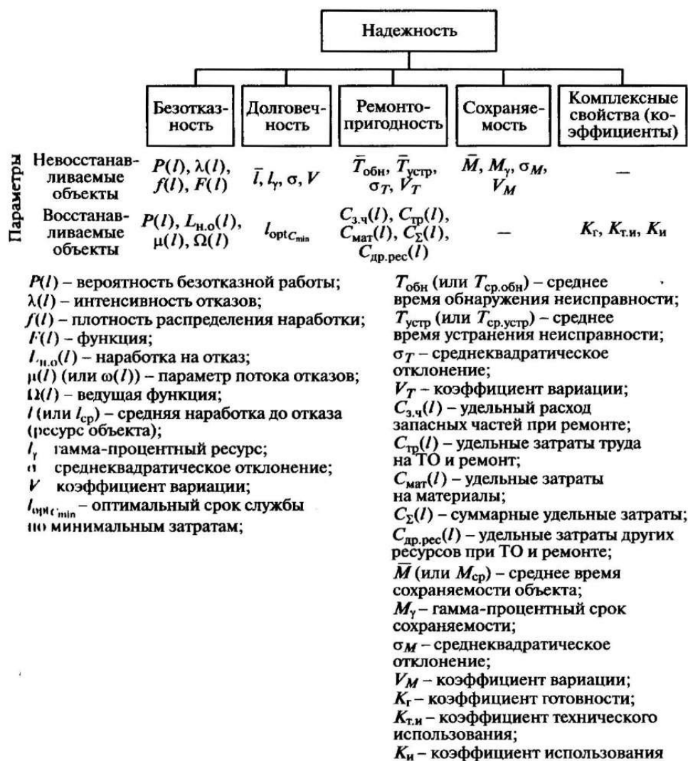
Рис. 3.9. Структура надежности
