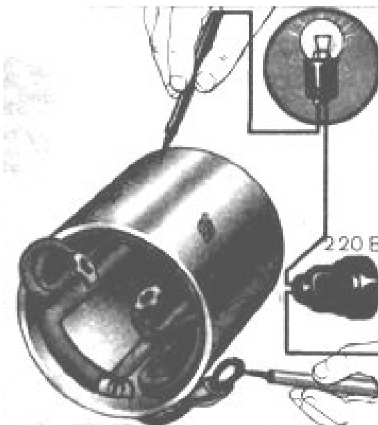
Рис. 7. Испытание обмоток возбуждения на замыкание с корпусом.
