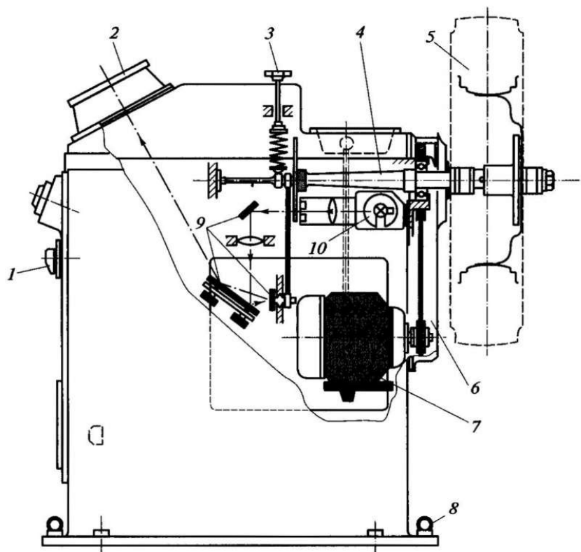
Рис. 5.25. Стенд для балансировки колес, снятых с автомобиля: 1 — выключатель станка; 2 — экран станка; 3 — регулировочный винт; 4 — балансирующий вал; 5 — колесо, снятое с автомобиля; 6 — ремни привода станка; 7 — электромотор привода; 8 — транспортные рым-болты; 9 — зеркала, направляющие отклоненный луч на экран; 10 — источник света
