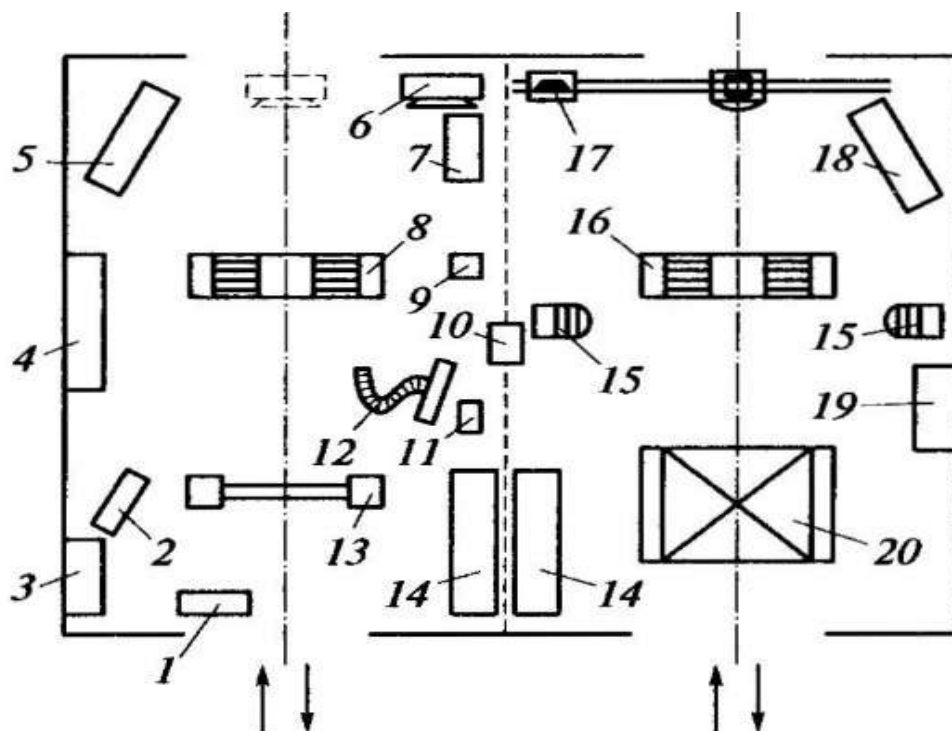
Рис. 3. Схема организации диагностирования автомобилей на СТОА
