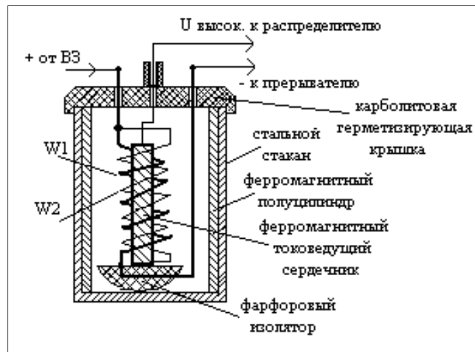
Схема катушки зажигания
