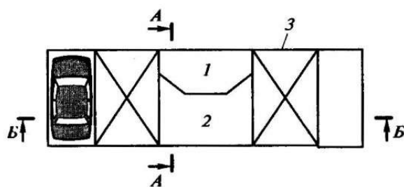
рис. 4.12. Схема механизированной стоянки на 50 автомобилемест:
