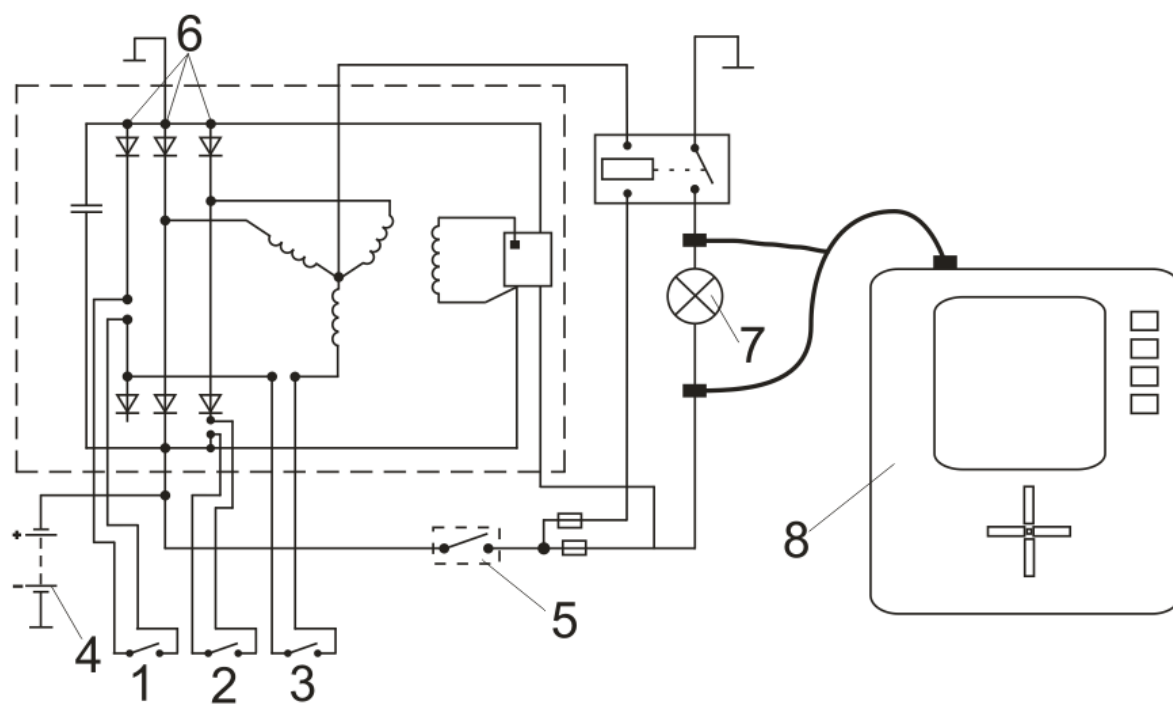
Рис 5. Электрическая схема лабораторной установки для испытания генераторов: 1 – выключатель имитации обрыва положительного диода; 2 – выключатель имитации отрицательного диода; 3 – выключатель имитации обрыва обмотки; 4 – аккумуляторная батарея; 5 – выключатель обмотки возбуждения, 6 – выпрямительные диоды, 7 – нагрузочная лампа, 8 - осциллограф DMO 510.
