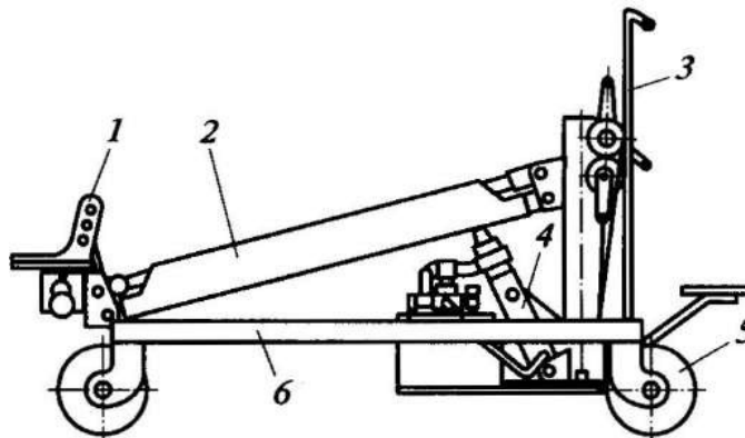
Рис. 5.16. Тележка для снятия и постановки рессор: 1 — захват для рессор; 2 — стрела; 3 — рукоятка; 4 — гидроцилиндр; 5 — колесо; 6 — щитовая балка
