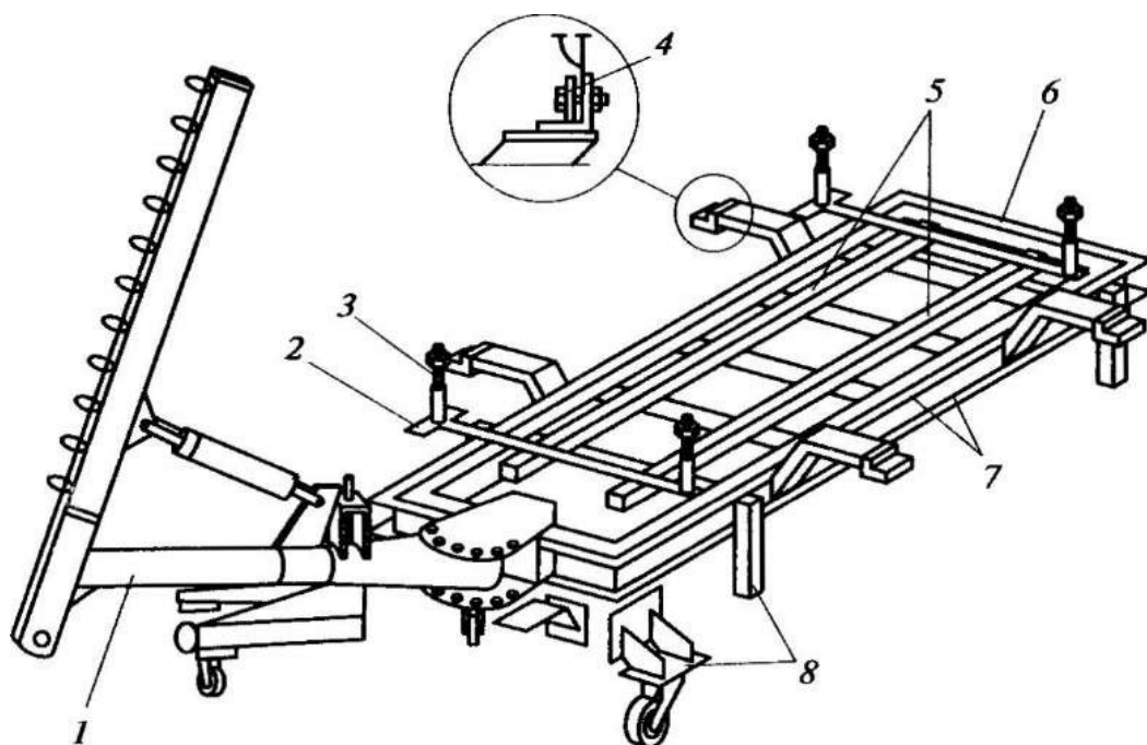
1'ис. 5.27. Стенд для правки и контроля фирмы «Каролинер»:
