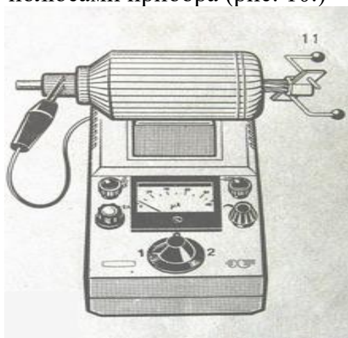
Рис.10. Проверка ротора на наличие межвиткового замыкания.
