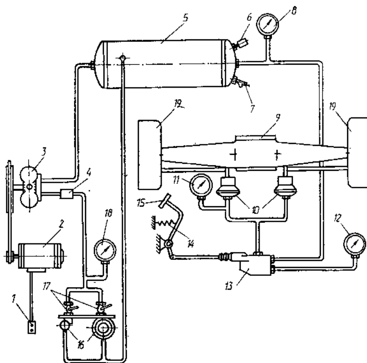
Рис.1. Схема установки для проверки и регулировки тормозов с пневматическим
