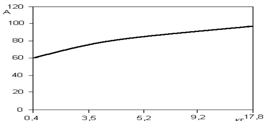
Рис. 5. Диаграмма зависимости величины тока от нагрузки на стартер
