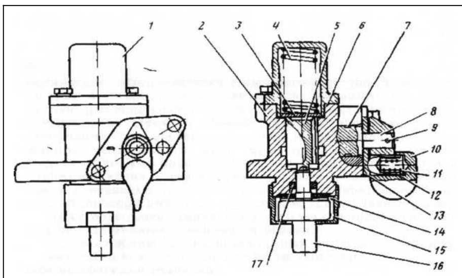
Включатель гидромфты двигателя КамАЗ 740
