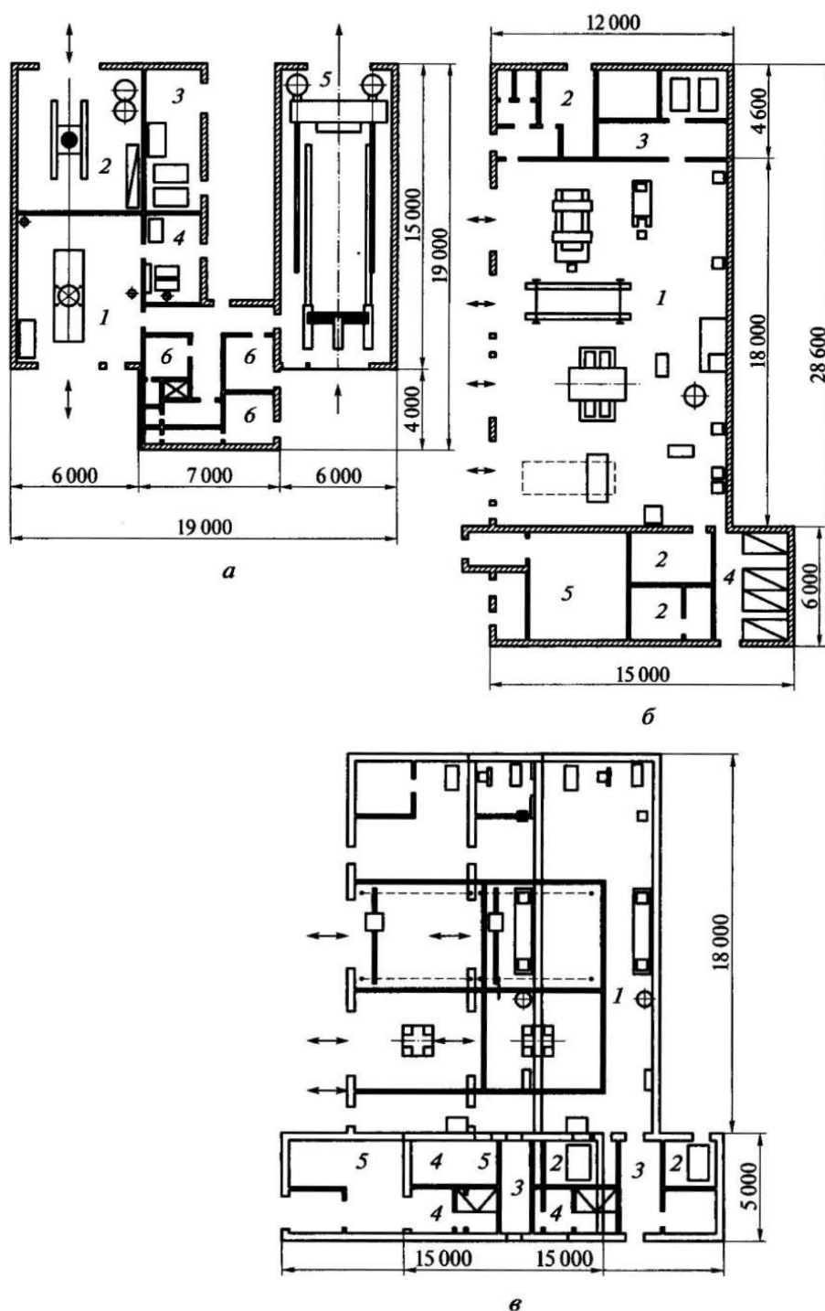
Рис. 2. Планировка дилерской СТОА на 35 рабочих постов: Бытовые помещения; 2 — кладовая красок; 3 — краскоприготовительная; 4 — окрасочный участок; 5 — ТО и ТР погрузчиков; 6 — зарядная; 7 — компрессорная; 8- инженерный блок; 9 — сварочно-жестяницкий участок; 10 — кладовая масел; 11- шинный участок; 12— инструментально-раздаточная кладовая; 13— бытовые помещения; 14 — промежуточный склад; 15 — участок ТО и ТР автомобилей; 16 — шиномонтажный участок; 17 — линия мойки автомобилей; 18 — линия предпродажной подготовки автомобилей; 19 — административные помещения; 20 — выставка автомобилей; 21 — центральный склад
