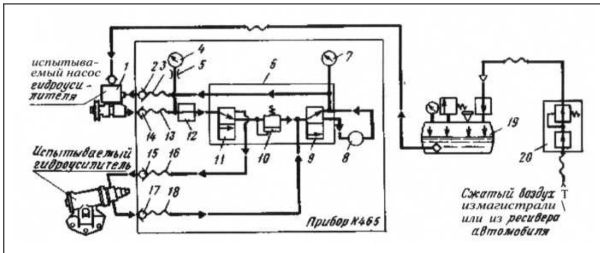
Схема подключения установки модели K465M
