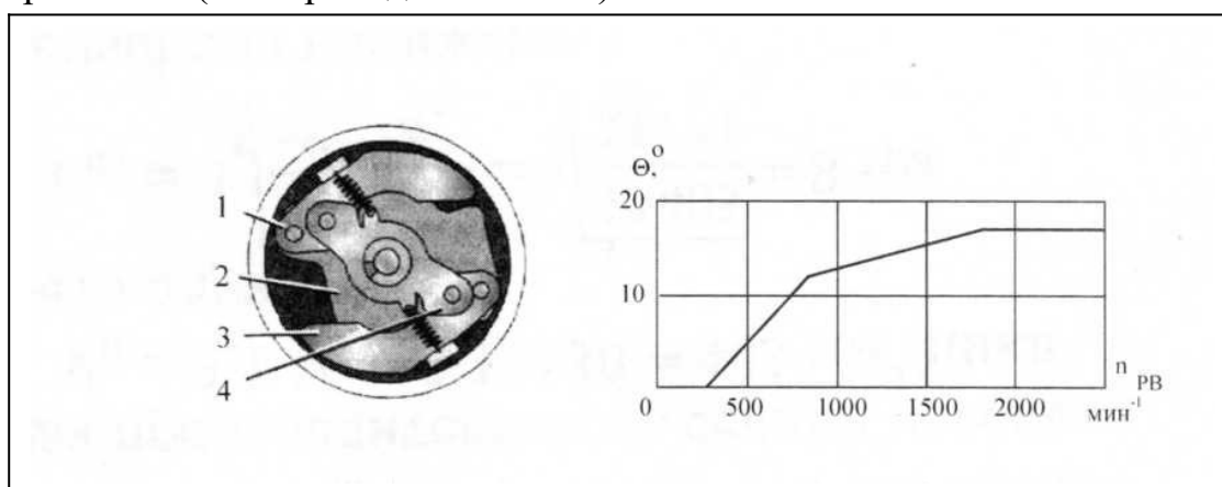
Конструктивное исполнение центробежного регулятора опережения зажигания и его характеристика 1, 3 – грузики, 2 – опорная пластина, 4 – траверса с пружинами.
